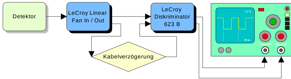
Abbildung 4.36: Aufbau zur Bestimmung der Doppelpulsauflösung
