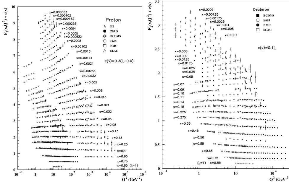
Abbildung 2.2: Gemessene Strukturfunktionen F_2^p und F_2^d in tiefinelastischen Streuexperimenten von Positronen [ C^+01 , A^+01 ], Elektronen [ W^+92 ] und M\mu onen [ B^+89 , A^+96a , A^+97d ] an Protonen bzw. Deuteronen. Aufgetragen sind F_2^p und F_2^d als Funktion von Q^2 bei konstanten Werten für x .
