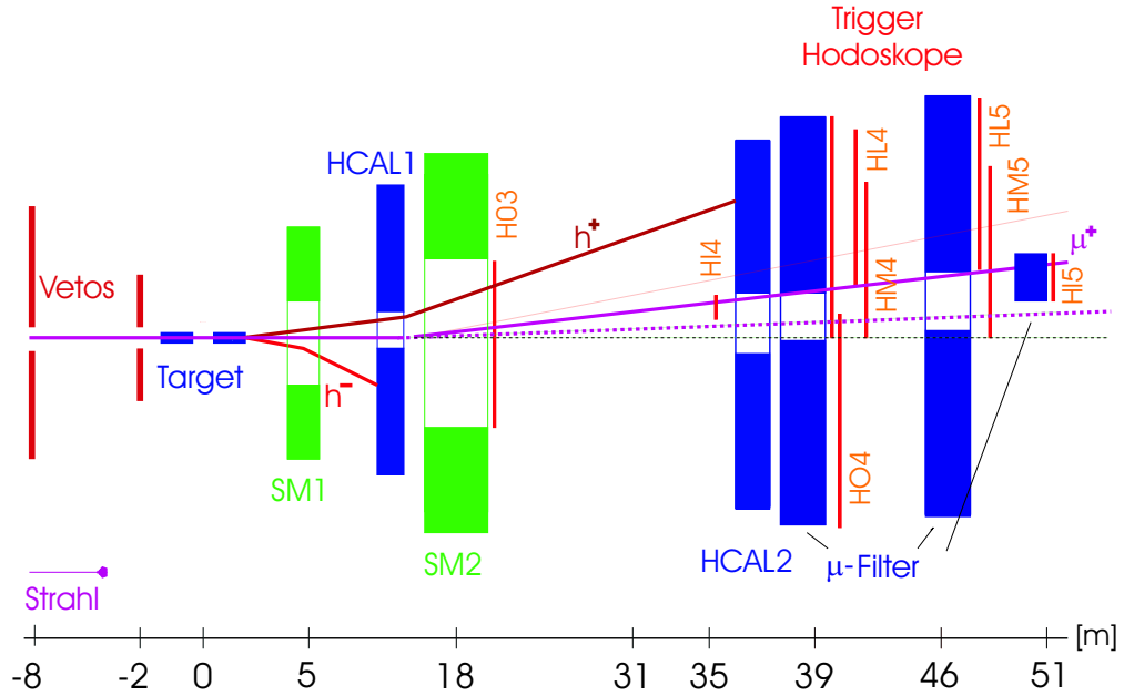
Abbildung 3.10: Schematischer Aufbau des Triggersystems bei COMPASS. Die Spektrometermagnete SM1 und SM2 trennen unter Energieverlust gestreute M\mu onen von Strahl \mu onen (punktiert). In diesem Fall lösen die Hodoskope HI4, HM4 und HI5 ein Triggersignal aus, das mit Q^2 \leq 0.5 \text{ GeV}^2 und dem Nachweis von Hadronen in den Kalorimetern ein Kandidat für ein PGF-Ereignis ist.
