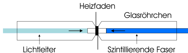
Abbildung 4.22: Aufbau zum Verschweißen von Fasern.
