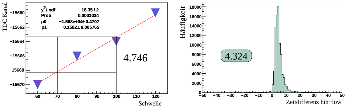
Abbildung 5.8: Links: Der aus dem Schwellenscan erwartete Wert für die Zeitdifferenz bei den im Experiment gesetzten Schwellen von thr_{low} = 70\text{mV} und thr_{hih} = 100\text{mV} . Rechts: Korrigiertes Zeitdifferenzspektrum. Der Meanwert hat sein Maximum der Verteilung im theoretisch erwarteten Bereich.
