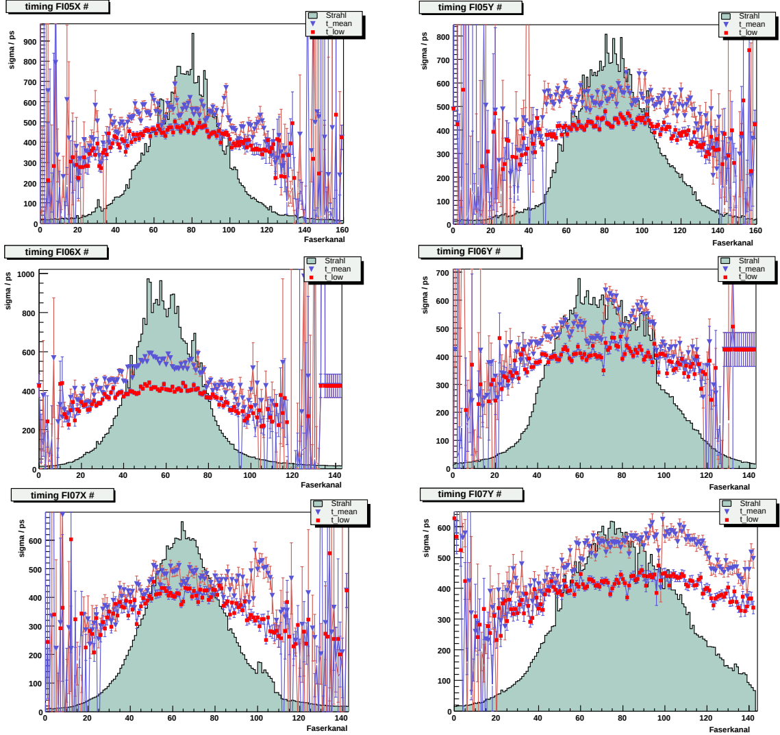
Abbildung 5.21: \sigma_{t_{low}} und \sigma_{<t_{low}>^{n-1/n}} gemessen über die Breite des Strahlprofils der Ebenen FI05XY (oben), FI06XY (mitte) und FI07XY (unten). Die Werte der durch mean timing gewonnen Datenpunkte (blaue Dreiecke) eines Clusters sind gegenüber den Zeitaufösungen \sigma_{t_{low}} der zeitführenden Faser (rote Quadrate) erhöht.
