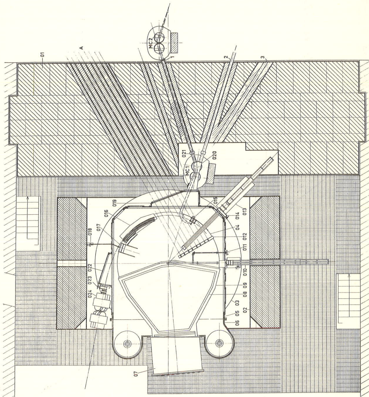
Schéma des canaux d'extraction des faisceaux à l'intérieur du mur de protection, côté salle des neutrons.
