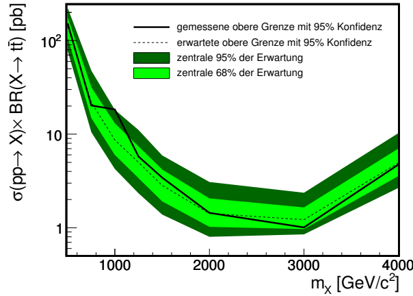
Abbildung 3: Erwartete und gemessene Ausschlussgrenzen mit einer Konfidenz von 95% für den Wirkungsquerschnitt des Prozesses pp \rightarrow X \rightarrow t\bar{t} mit einem hypothetischen Austauschteilchen X als Funktion der Masse dieses Teilchens.
