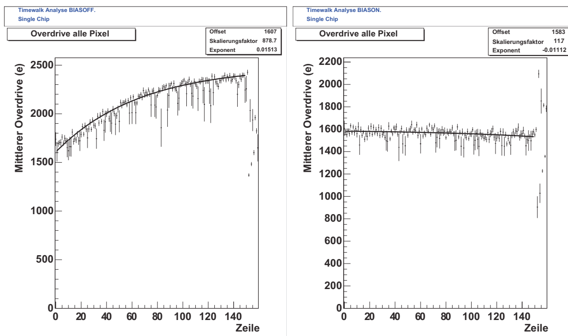
Abbildung 6.25: Die beiden Messungen zeigen den mittleren Overdrive einer Zeile aufgetragen gegen die Zeilennummer gemessen ohne Bias-Kompensation (links) und mit Bias-Kompensation (rechts)
