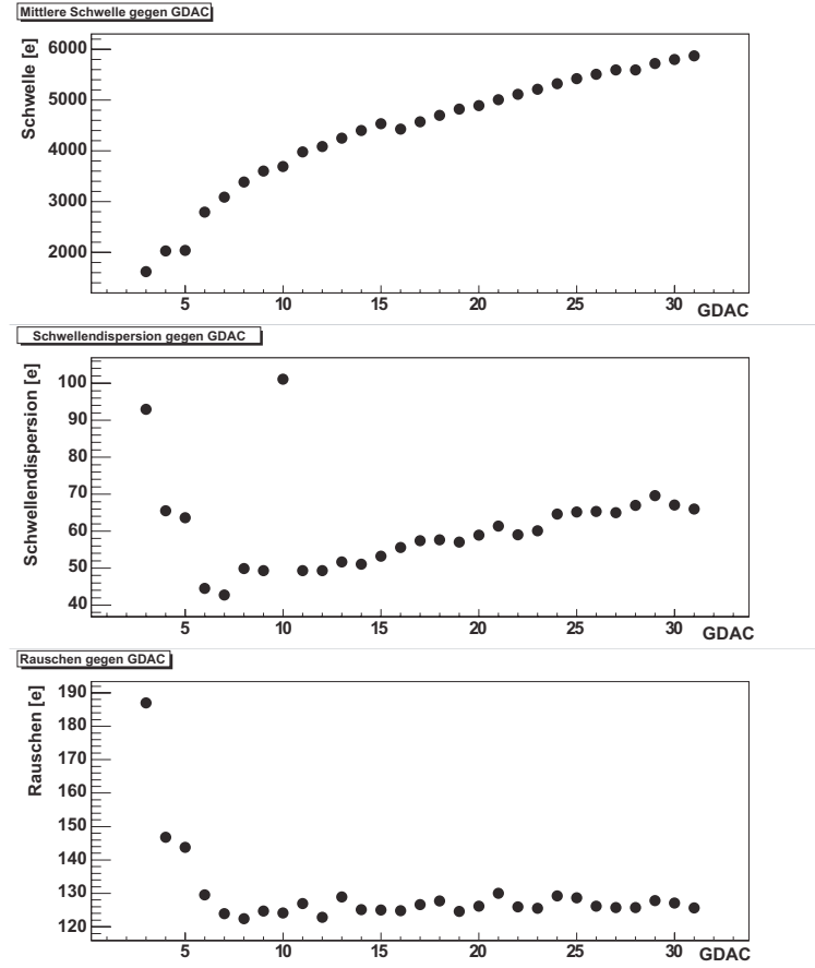
Abbildung 6.22: Änderung der Schwelle, der Schwelligendispersion und des Rauschens mit der globalen Schwelleneinstellung GDAC. Die Feineinstellung der Schwellen wurde bei einem GDAC-Wert von 7 vorgenommen.
