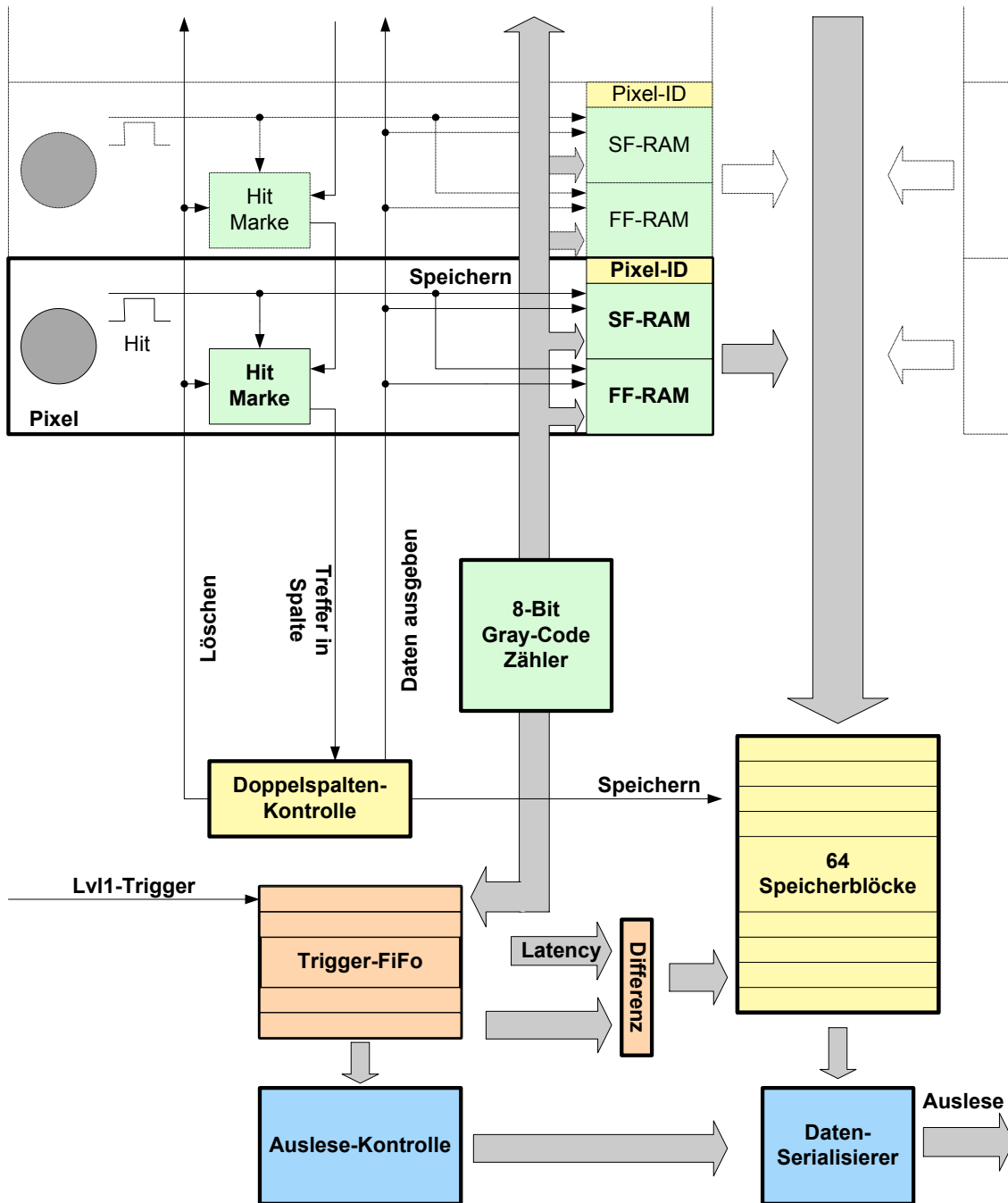
Abbildung 5.12: Schematische Darstellung der Auslese der Trefferdaten im FE-I2 Chip
