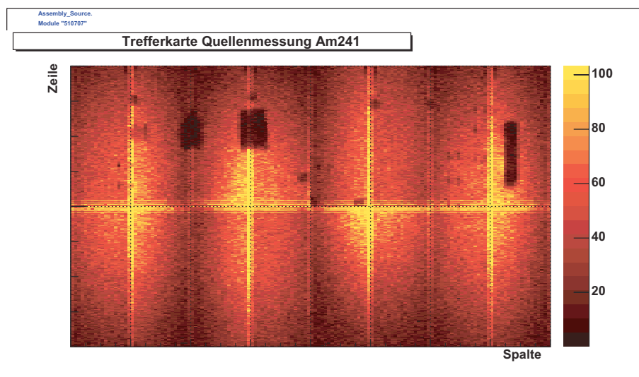
Abbildung 6.38: Anzahl der Treffer pro Pixel nach Bestrahlung eines Moduls (510707) mit einer ^{241}\text{Am} -Quelle
