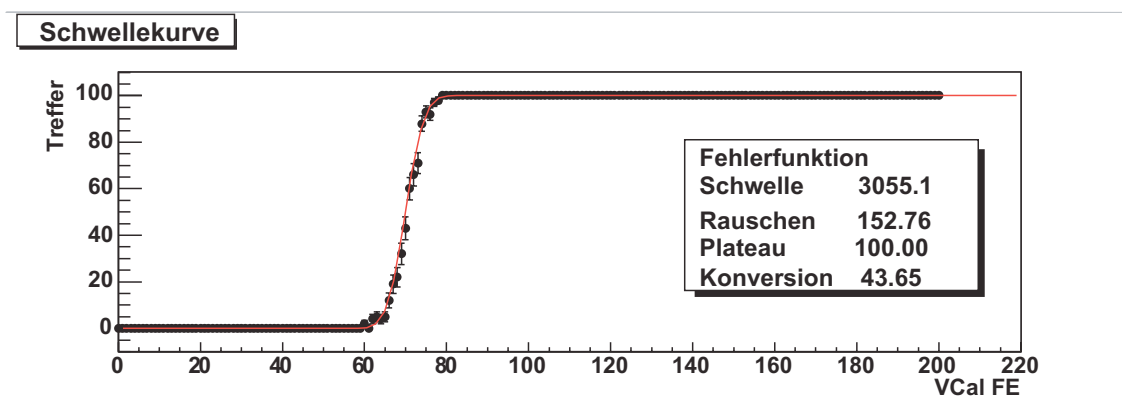
Abbildung 6.15: Mittels des internen Pulsgenerators gemessene S-Kurve eines Pixels und den daraus errechneten Parametern Schwelle und Rauschen
