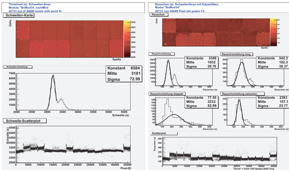
Abbildung 7.15: Schwellen (links) und Rauschmessung (rechts) des Moduls BnMod34 mit konstantem Strom, nachdem 11 der 16 FE-Chips mit individuellen Endkoppelkapazitäten von 100 nF verbunden worden sind.
