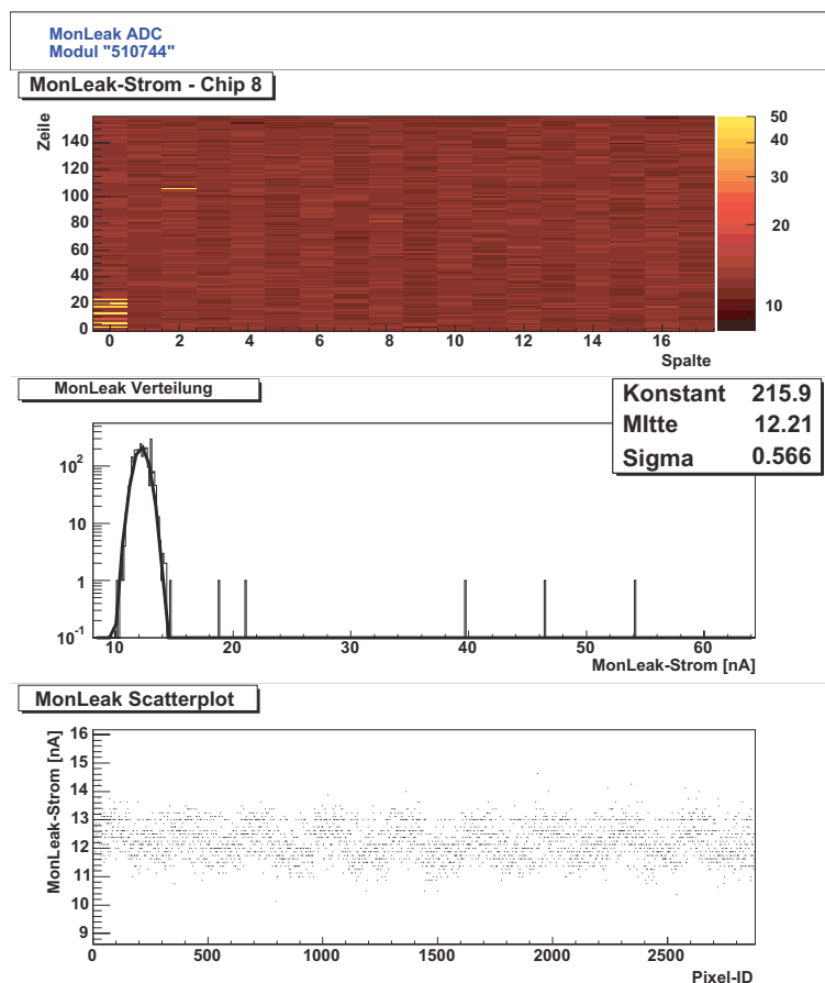
Abbildung 6.34: Leckstrommessung von FE-Chip 8 auf Modul 510744 über den internen ADC
