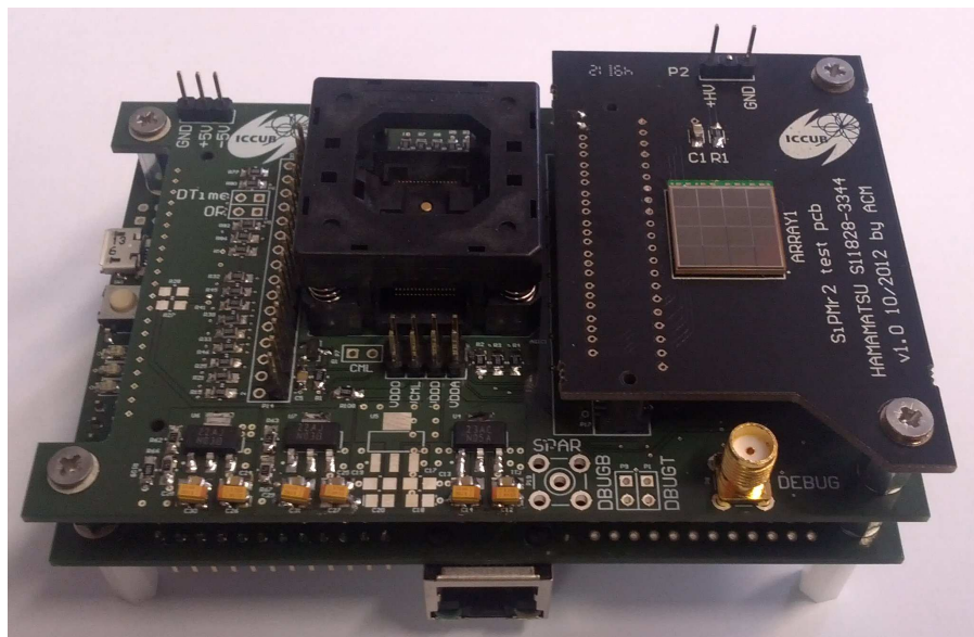
Figure 11: Sistema de test
