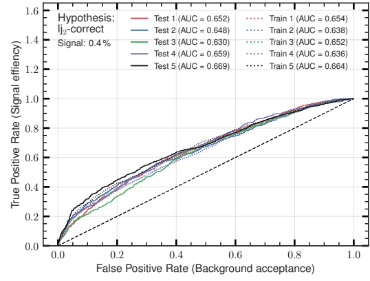
(d) ROC curves of permutation 24 of the l_{j_2\text{correct}} -DNN.
