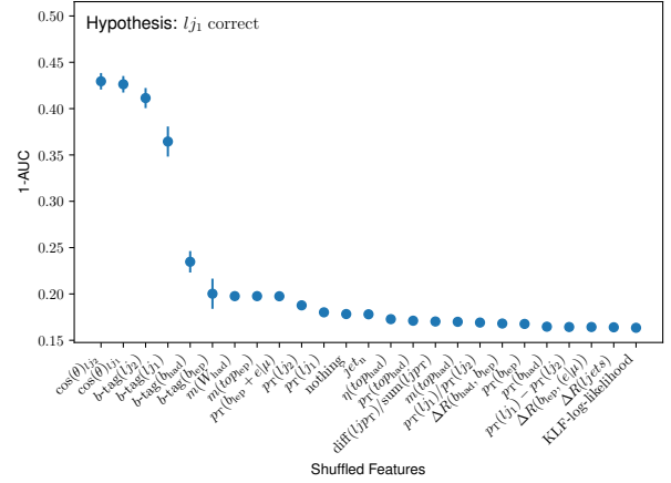
(d) Feature importance diagram of the lj_{1,\text{correct}} -DNN.
