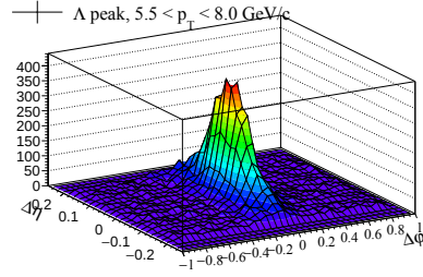
(d) \Lambda : 5.5 < p_T < 8.0 GeV/c
