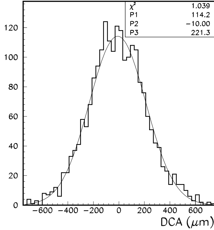
Figura 7. Mínima distancia transversa (en \mu\text{m} ) al vértice de las trazas reconstruidas en la cámara de vértice de L3. El ajuste corresponde a una gaussiana de anchura P3.
