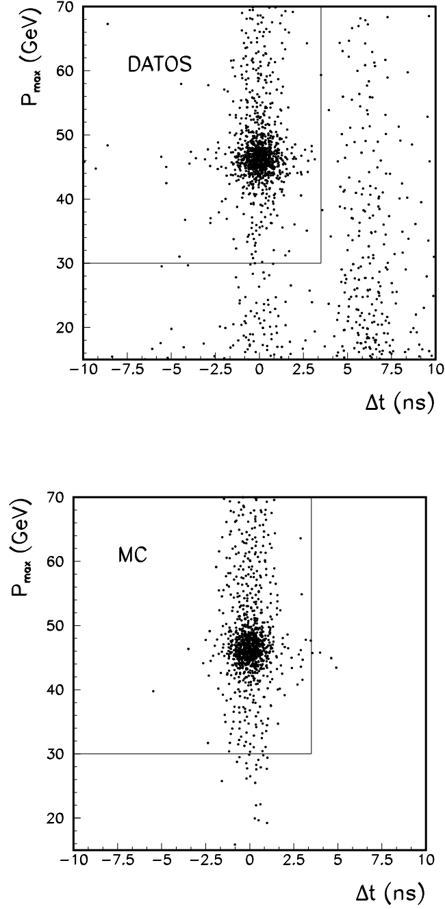
Figura 12. Momento del muón más energético frente a la diferencia de tiempos entre ambos muones. En la figura se representan datos y Monte Carlo, donde se han impuesto ligeros cortes en la extrapolación al vértice de las trazas muónicas (200 mm). La concentración de sucesos en torno a \Delta t = 6 ns corresponde a rayos cósmicos que no aparecen en la simulación, pero que son fácilmente identificables. La concentración de sucesos en torno a \Delta t = 0 ns y bajo momento corresponde a sucesos e^+e^- \rightarrow e^+e^-\mu^+\mu^- y e^+e^- \rightarrow \tau^+\tau^- \rightarrow \mu^+\mu^-\nu\nu
