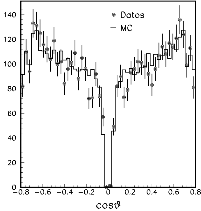
Figura 11. Distribución de los sucesos e^+e^- \rightarrow \mu^+\mu^-(\gamma) según \cos \theta . Se observa un claro descenso de la eficiencia para valores |\cos \theta| > 0.7 , debido a las celdas muertas existentes en el detector de muones.
