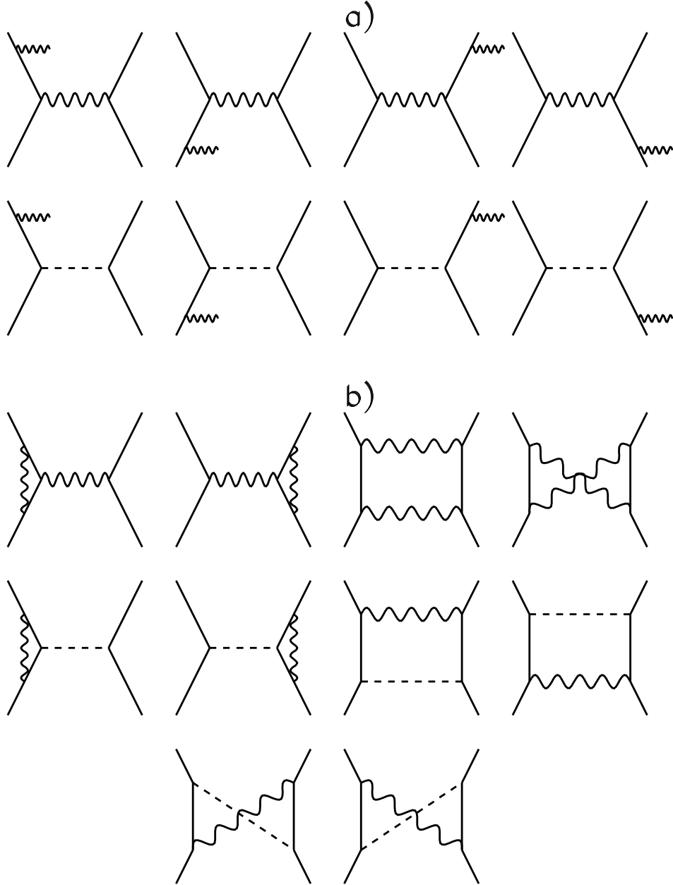
Figura 2. Correcciones radiativas QED en primer orden al proceso e^+e^- \rightarrow f\bar{f} : a) diagramas con emisión real de fotones, b) correcciones virtuales.
