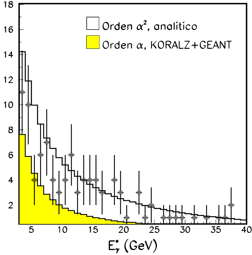
Figura 11. Espectro de energías en la variable E_\gamma^* para sucesos \mu^+\mu^-\gamma\gamma . Se observa un buen acuerdo entre datos y simulación cuando se añaden las predicciones analíticas de orden \alpha^2 . Sólo se muestran sucesos con E_\gamma^* > 3 GeV para evitar la zona afectada por el corte aplicado en la energía mínima del fotón.
