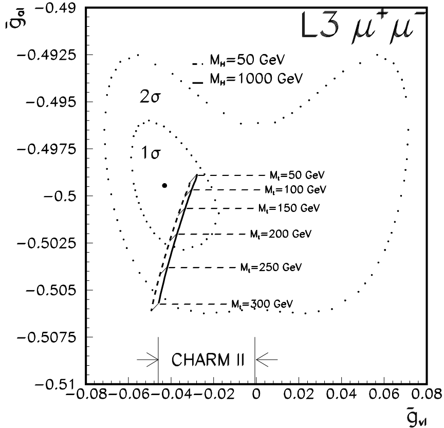
Figura 5. Valores de las constantes de acoplo leptónicas usando los canales e^+e^- \rightarrow \mu^+\mu^-(\gamma) y e^+e^- \rightarrow \text{hadrones} en L3. Se representan asimismo los contornos correspondientes a 1 y 2 desviaciones estándar con respecto a la medida central, la predicción del modelo estándar y una de las medidas más precisas fuera del marco de LEP, la del cociente g_v/g_a por el experimento CHARM II [7].
