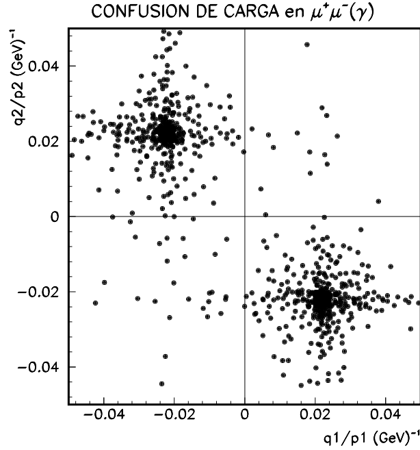
Figura 9. Histograma doble en el que se puede apreciar cuál es la confusión de carga y el efecto de la resolución en momento para la muestra e^+e^- \rightarrow \mu^+\mu^-(\gamma) . Los sucesos con confusión de carga aparecen en los cuadrante superior derecho e inferior izquierdo, respectivamente. El hecho de que estos sucesos estén muy alejados del resto demuestra que la resolución del espectrómetro de muones no es la causa de la confusión existente.
