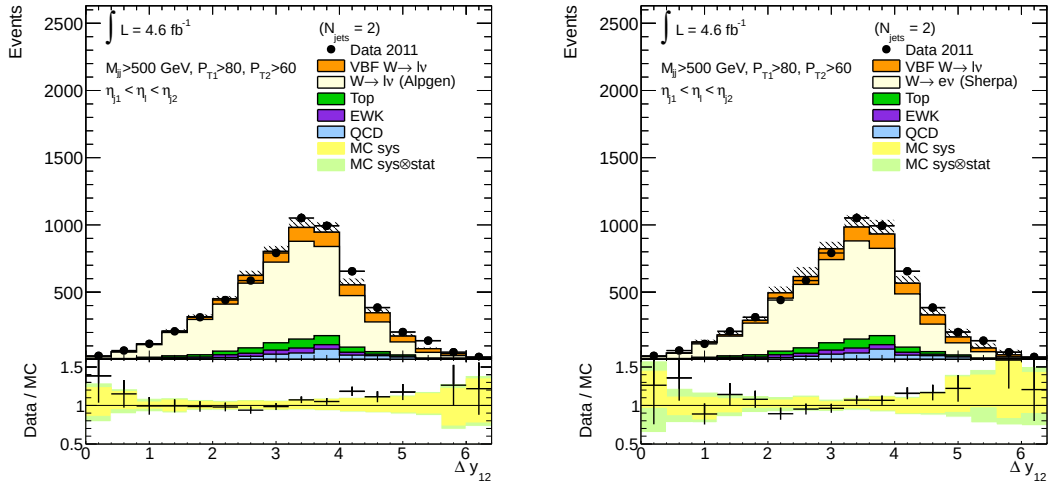
(c) Combined \Delta y(j_1, j_2) (ALPGEN W + \text{QCD jets} ) (d) Combined \Delta y(j_1, j_2) (SHERPA W + \text{QCD jets} )
