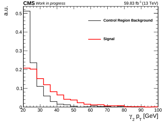
(d) p_T(\gamma_2) for m_\Phi = 50 GeV.
