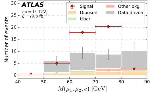
(d) Signal sample: M_N = 30 GeV, c\tau = 10 \mu\text{m} .
