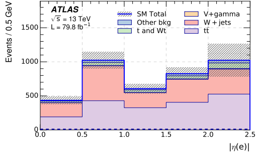
(d) Electron MR with N_{b\text{-jets}} \geq 1 .
