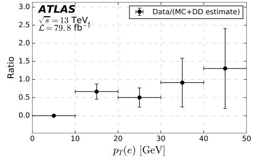
(b) \mu_2 : FixedCutLoose isolation. e : Loose isolation.
