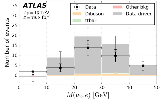
(d) \mu_2 : Loosened FixedCutLoose isolation. e : Loose isolation.
