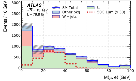
(b) M_N = 50 GeV.
