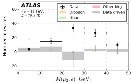
(e) \mu_2 : Loose isolation. e : Gradient isolation.
