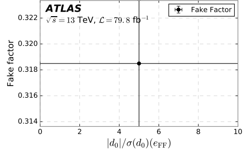
(d) Applied binning for Fig. 128c.
