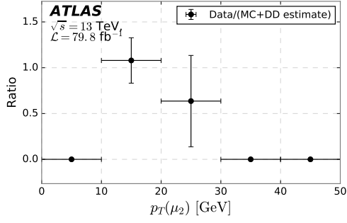
(a) \mu_2 : FixedCutLoose isolation. e : Gradient isolation.
