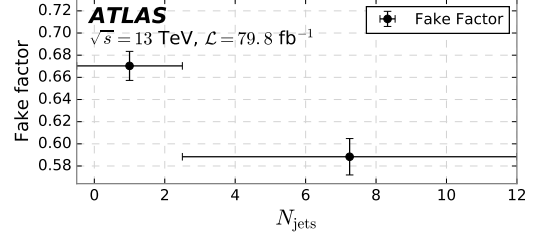
(d) Applied binning for Fig. 124c.
