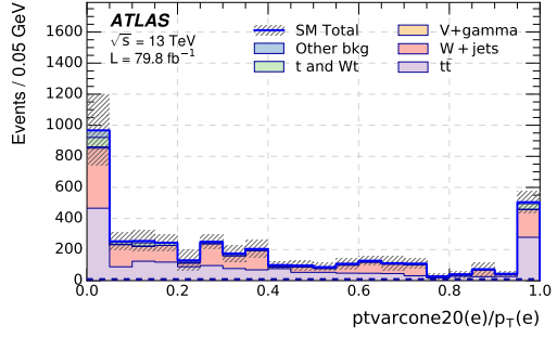
(d) Electron MR with N_{b-jets} \geq 1 .
