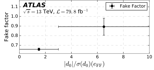
(d) Applied binning for Fig. 125c.
