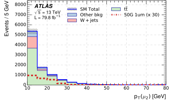
(b) M_N = 50 GeV.
