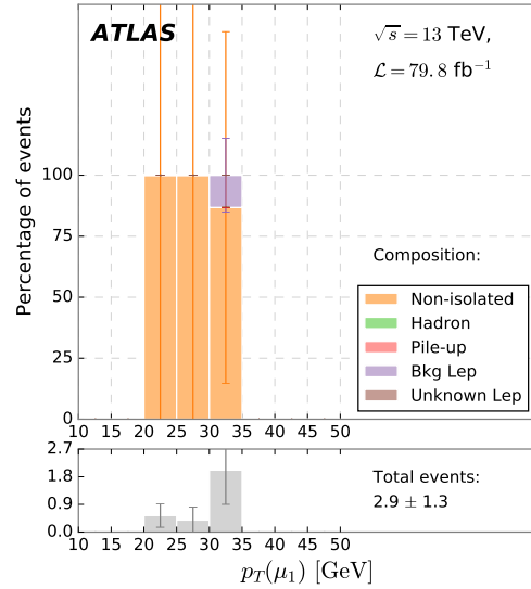
(d) Fake \mu_1 , real \mu_2 and real e .
