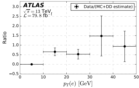
(c) \mu_2 : Loosened FixedCutLoose isolation. e : Gradient isolation.
