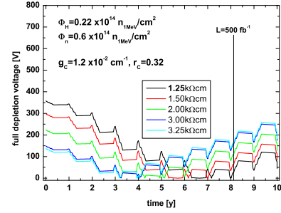
(d) Low hadron fluence and values from Table 6.3
