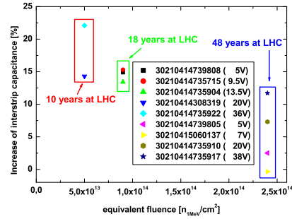
(d) Increase of interstrip capacitance values after proton irradiation
