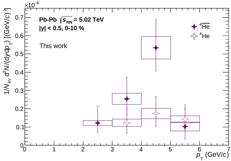
(b) (Anti) ^4He .
