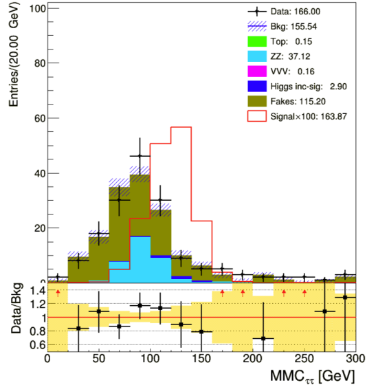
(d) Z \rightarrow ll & H \rightarrow \tau_{\text{had}}\tau_{\text{had}} (Ditau MMC)
