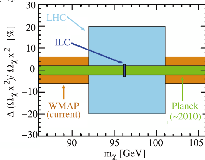
Слика 1.1.4 Релативна грешка мерења густине тамне материје у функцији масе неутрина (као LSP) у садашњим (WMAP) и будућим експериментима (LHC, ILC, Planck).
