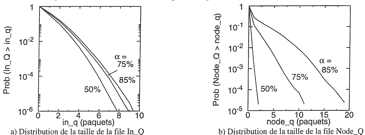
Figure 6-5: File d'attente In\_Q et Node\_Q .
