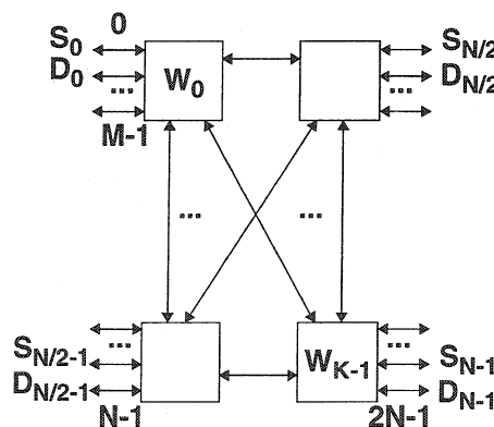
Réseau en étoile
