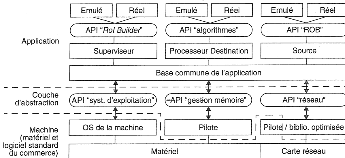
Figure 9-2: .Structure du logiciel.
