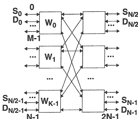
Omega, Banyan..., à deux étages
