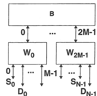
Dorsale + commutateurs d'accès
