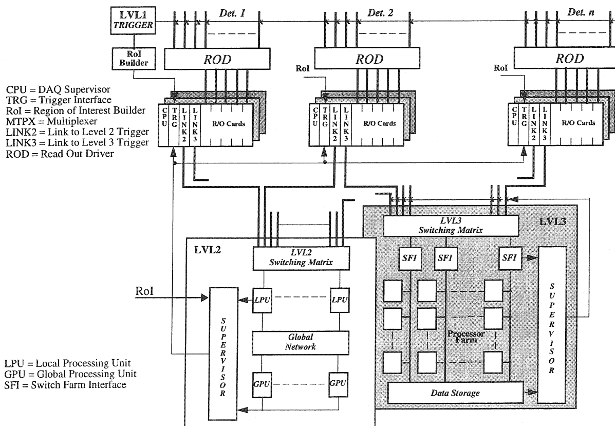
Figure 2-1: Architecture du T/DAQ d'ATLAS d'après le Technical Proposal .
