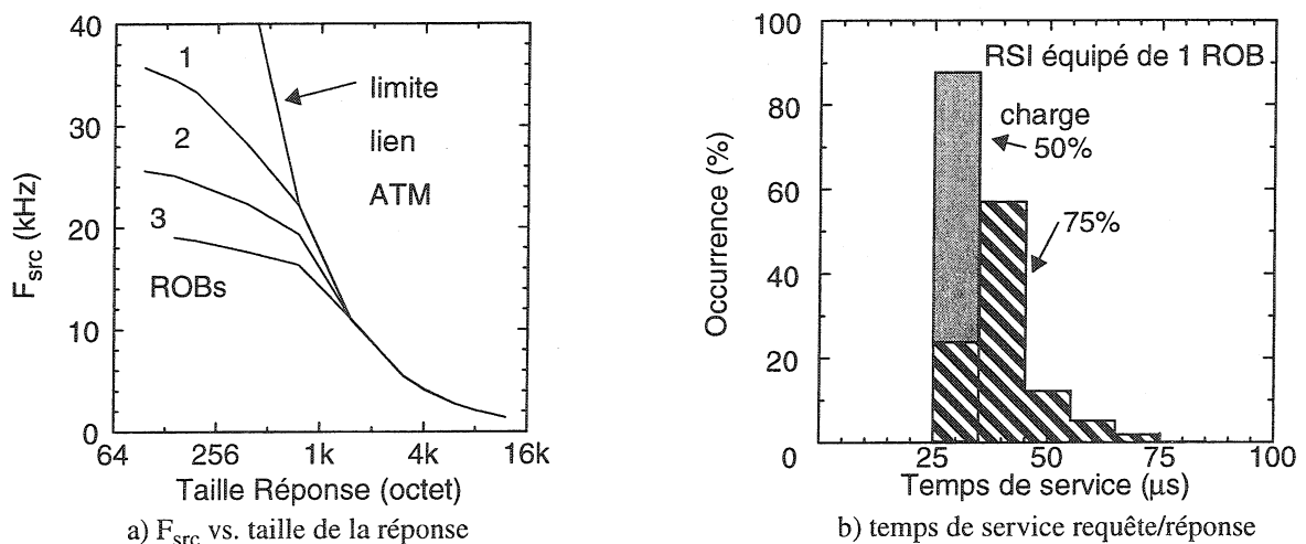
Figure 9-6: Fréquence de service du RSI/ROBs.
