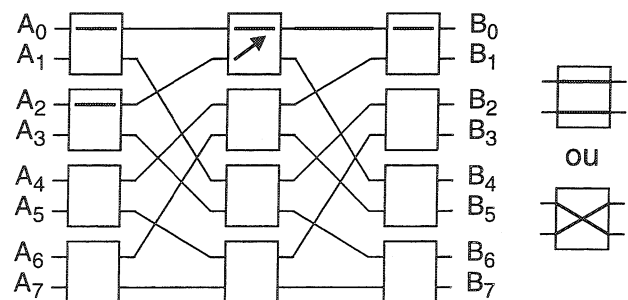
b) Réseau Omega
