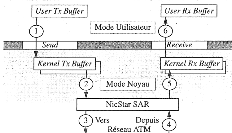
Figure 7-2: Fonctionnement du pilote de carte réseau ATM.
