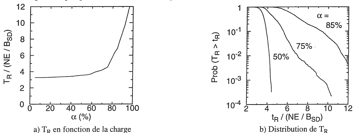
Figure 6-4: Temps de ré-assemblage.
