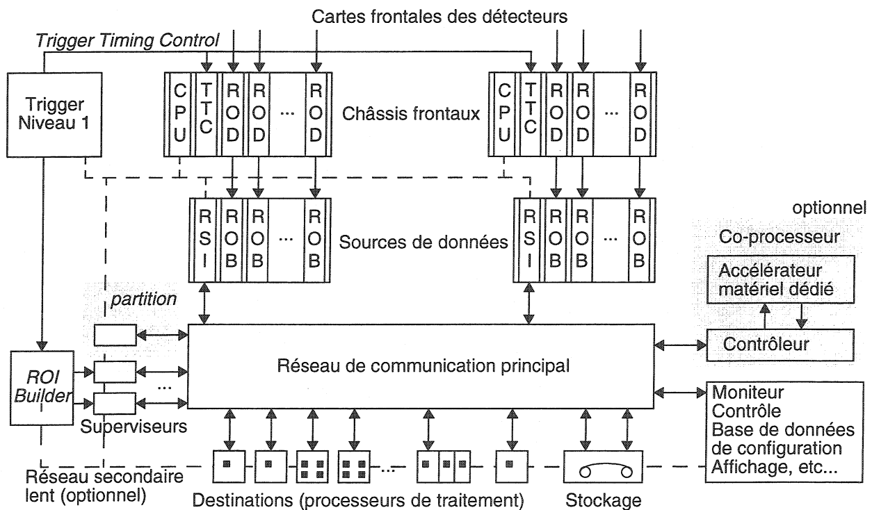
Figure 4-2: Schéma de principe de l'architecture proposée.
