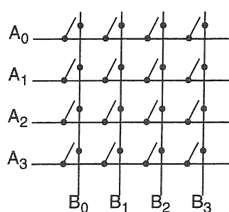
a) Réseau crossbar
