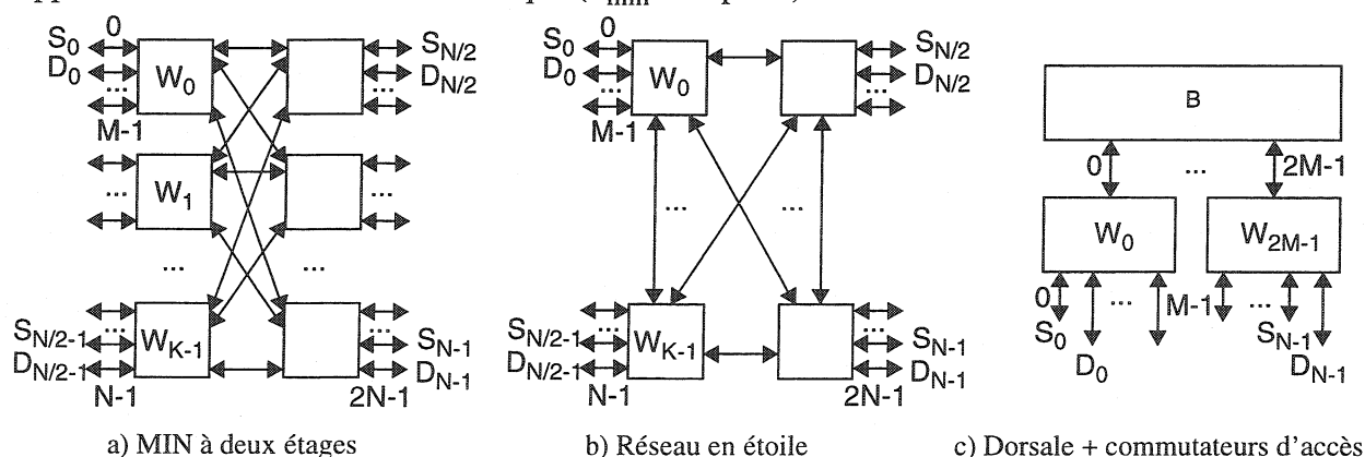
Figure 6-9: Assemblage de commutateurs.
