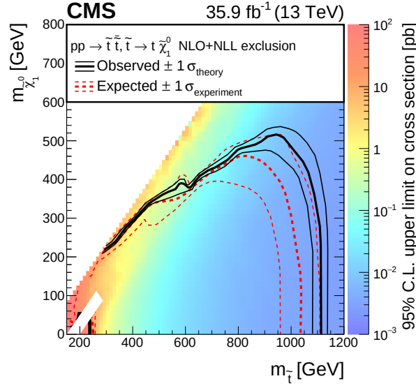
Figure A.11: Les limites d'exclusion à 95% CL sur le modèle T2tt correspondant à une luminosité intégrée de 35.9 fb -1 . L'interprétation est fournie dans le plan de la masse du stop par rapport à la masse du neutralino. Le code de couleur indique la limite supérieure de 95 % CL sur la section efficace en supposant un rapport de branchement de 100% pour \tilde{t}_1 \rightarrow t\tilde{\chi}_1^0 . Les contours rouge et noir représentent respectivement les limites d'exclusion attendues et observées. La zone sous la courbe épaisse noire indique la région exclue des points de signal.
