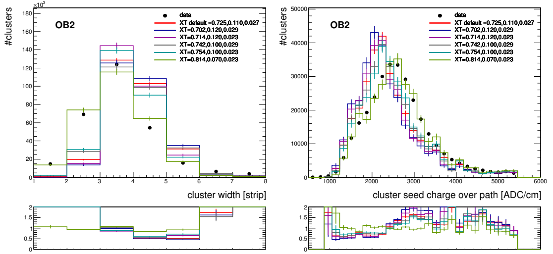
Figure A.7: Distributions de la largeur des amas (à gauche) et de la charge portée par la piste collectant le plus de signal dans l'amas (à droite) pour la géométrie OB2. Les données de collision sont représentées par les points noirs, différentes valeurs de la diaphonie XT sont utilisées dans la simulation (chaque set correspondant à une couleur différente). Le premier des trois nombres XT correspond à la fraction de charge induite sur la piste principale, les deuxième et troisième nombres représentent les fractions de charge induites sur les premiers et seconds voisins, respectivement. Les distributions simulées sont renormalisées au nombre d'amas dans les données. Les graphiques inférieurs représentent le rapport des distributions des données par la simulation.
