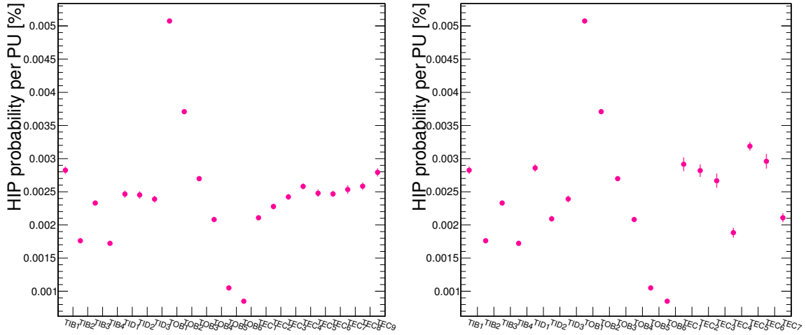
Figure A.4: Probabilité moyenne d’avoir un événement HIP par unité du pileup (PU) pour les couches du TIB et du TOB (aussi bien sur la figure de gauche que de droite) et pour les roues (à gauche) ou les anneaux (à droite) des partitions TID et TEC du trajectographe de silicium. Ces probabilités ont été calculées à partir du run 281604 enregistré en 2016 (2 e étude des HIP).
