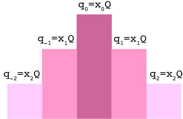
Figure A.6: Un schéma de partage de charge entre pistes voisines.
