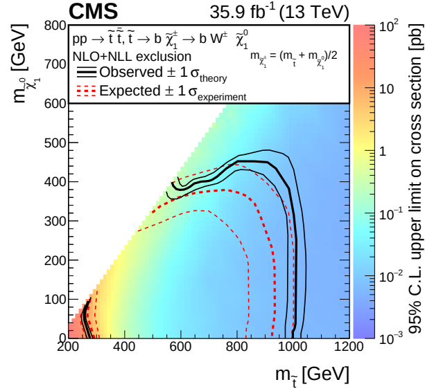
Figure A.12: Les limites d'exclusion à 95% CL sur le modèle T2bW correspondant à une luminosité intégrée de 35.9 \text{ fb}^{-1} . L'interprétation est fournie dans le plan de la masse du stop vs la masse du neutralino. Le code couleur indique la limite supérieure de 95% CL sur la section efficace en supposant un rapport de branchement de 100% pour \tilde{t}_1 \rightarrow b\tilde{\chi}_1^\pm . Les contours rouge et noir représentent respectivement les limites d'exclusion attendues et observées. La zone sous la courbe épaisse noire indique la région exclue des points de signal.
