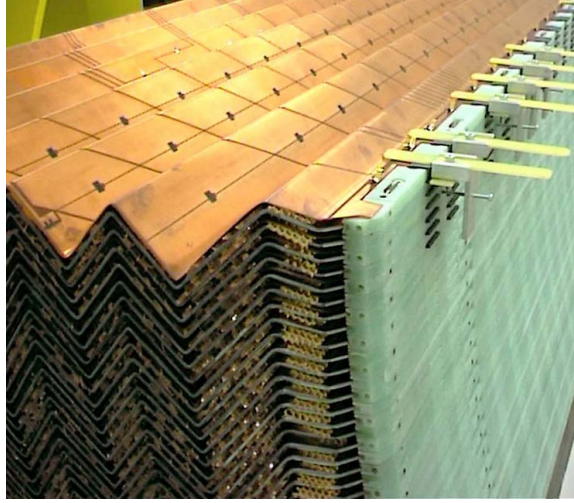
FIG. 5.9 – Photographie d’une portion de module permettant de visualiser l’empilement des électrodes positionnées à l’aide d’espaces en nid d’abeille et les connecteurs de lecture du signal du compartiment avant.
