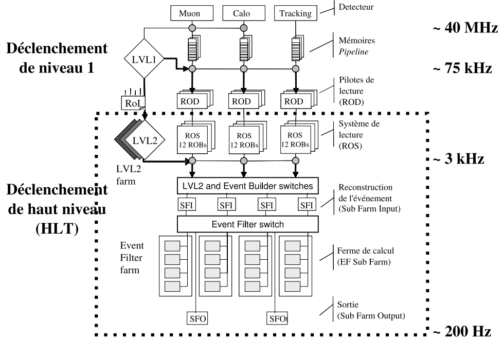
FIG. 4.6 – Schéma du système d'acquisition et de déclenchement [37]
