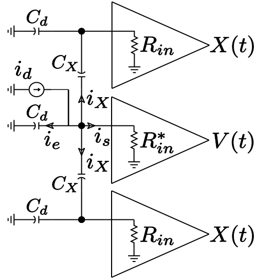
FIG. 9.6 – Schéma électrique équivalent de la diaphonie dans le compartiment avant utilisé pour le calcul du signal de diaphonie d'une cellule fuyante génèreuse.
