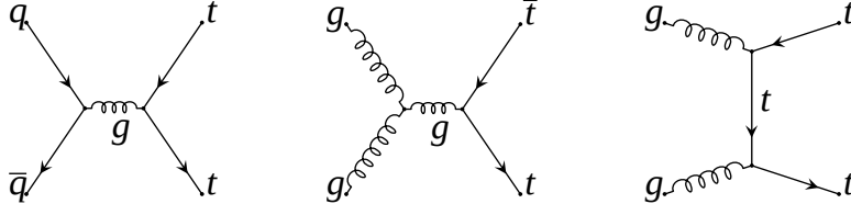
FIG. 10.1 – Diagrammes de production d'une paire t\bar{t} à l'ordre dominant par annihilation quark-antiquark ou fusion de gluons.
