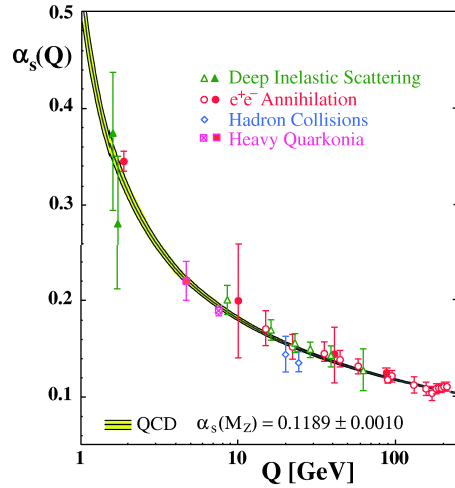
FIG. 2.3 – Mesure de la variation de la constante de couplage fort à différentes échelles d'énergie [13].
