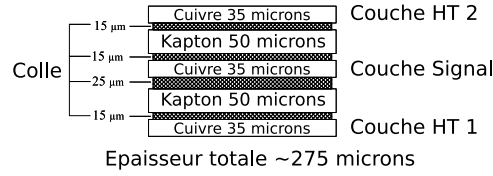
FIG. 5.3 – Détail sur la composition d'une électrode avec les deux couches haute tension (HT) et la couche centrale de lecture, séparées par l'isolant en kapton.
