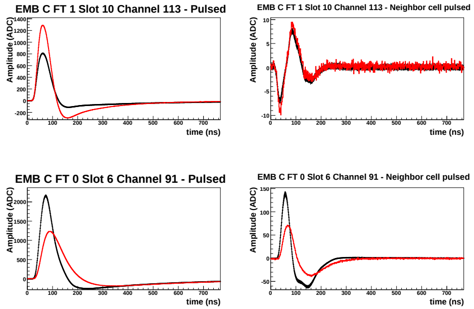
FIG. 9.4 – Illustration de voies distordues à cause d'un défaut dans la chaîne d'étalonnage ( haut ) ou de lecture ( bas ). Le signal étudié est tracé en rouge, le signal attendu en noir. Les signaux de gauche sont mesurés lorsque la cellule est injectée, ceux de droite représentent le signal de diaphonie qui apparaît lorsqu'une cellule voisine est injectée.
