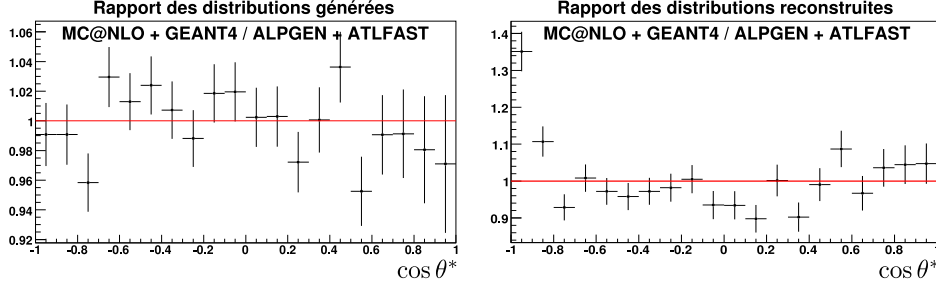
FIG. 12.4 – Comparaison des distributions en \cos \theta^* obtenues pour les échantillons “MC@NLO + GEANT4” et “ALPGEN + ATLFAST”. Gauche : rapport des distributions générées. Droites : rapport des distributions reconstruites (contenant au moins un lepton chargé et quatre jets reconstruits).
