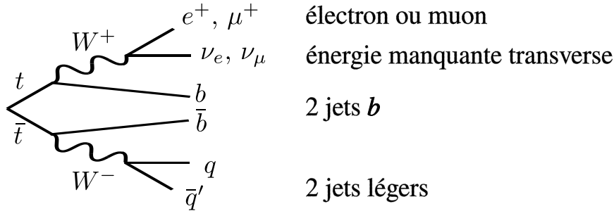
FIG. 11.1 – Topologie d'un processus de signal.
