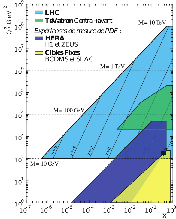
FIG. 3.3 – Régions en x et Q^2 accessibles pour différentes expériences [22]. M et y désignent respectivement la masse invariante et la rapidité (voir section 3.1.2) du système partonique.
