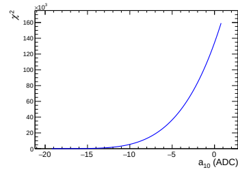
(d) \chi^2 for different a_{10} values
