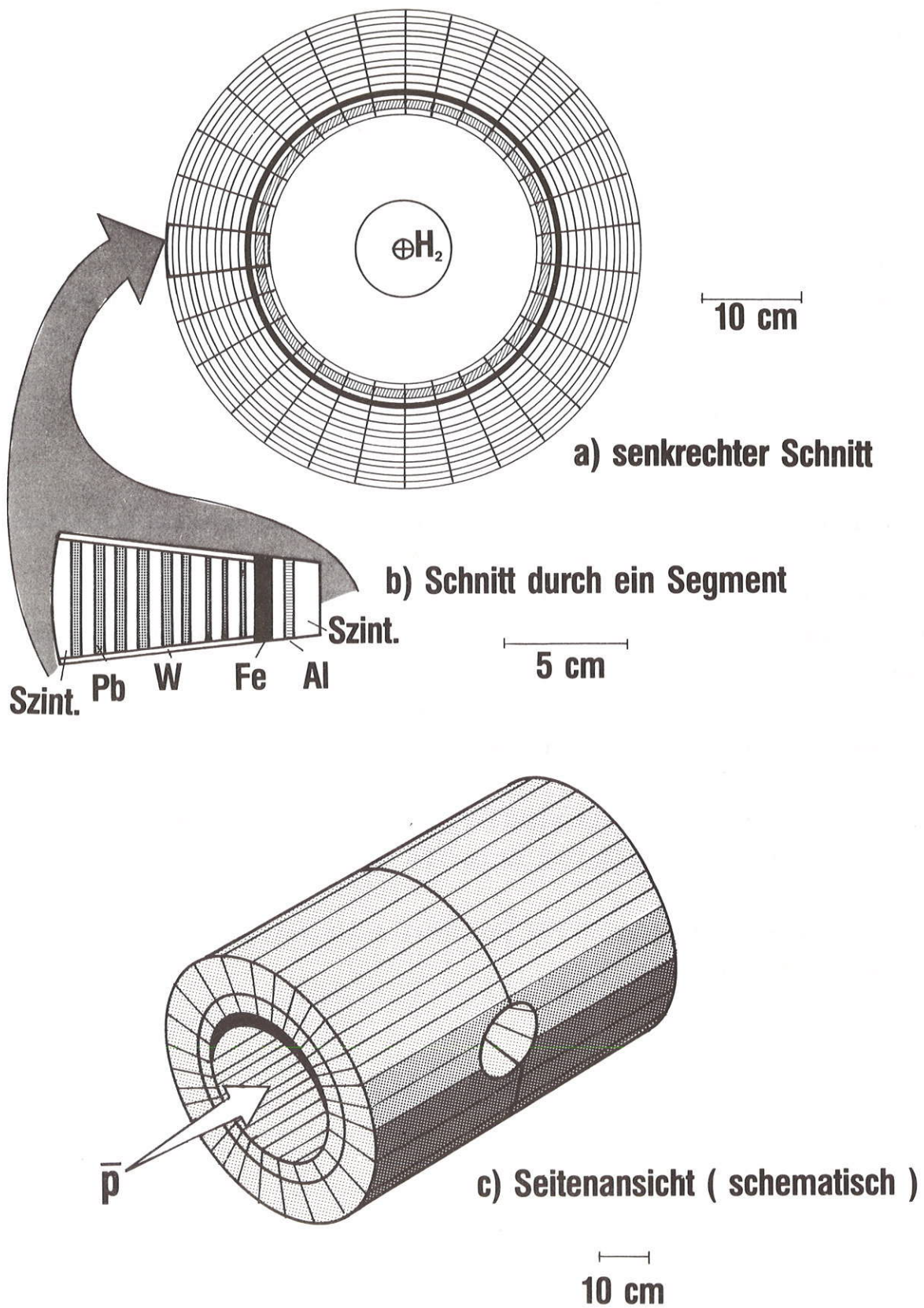
Abbildung 13 : Der Annihilationszähler
