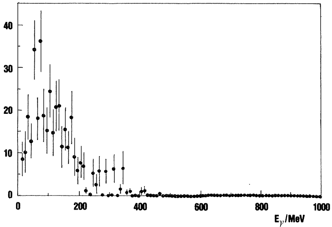
Abbildung 26 : Die \gamma -Spektren des modularen NAJ-Sektors für den Annihilationstrigger 4 geladene Teilchen und 3 \pi^0 's oben : gemessenes \gamma -Spektrum unten : Monte-Carlo \gamma -Spektrum
