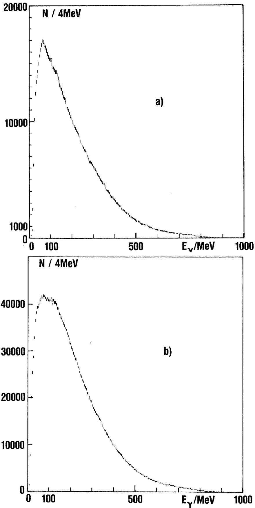
Abbildung 23 : Die totalen inklusiven \gamma -Spektren des modularen NAJ-Sektors, a. Experiment 1979, b. Experiment 1980
