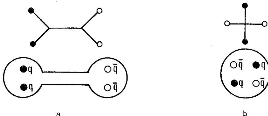
Abbildung 3 : Naives Modell der Quarkstruktur von Baryonium, die Struktur 3a sollte bevorzugt sein
