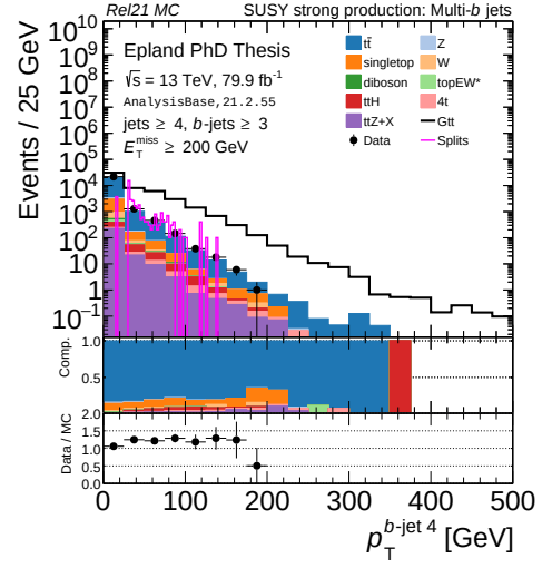
(b) p_T^{b\text{-jet } 4}
