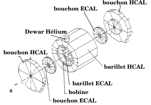
Figure 3.10: Les calorimètres électromagnétique (ECAL) et hadronique (HCAL).
