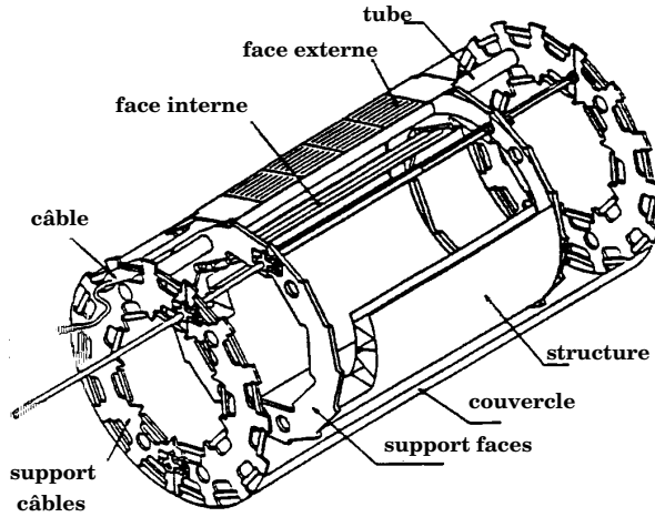
Figure 3.5: Schéma du détecteur de vertex.
