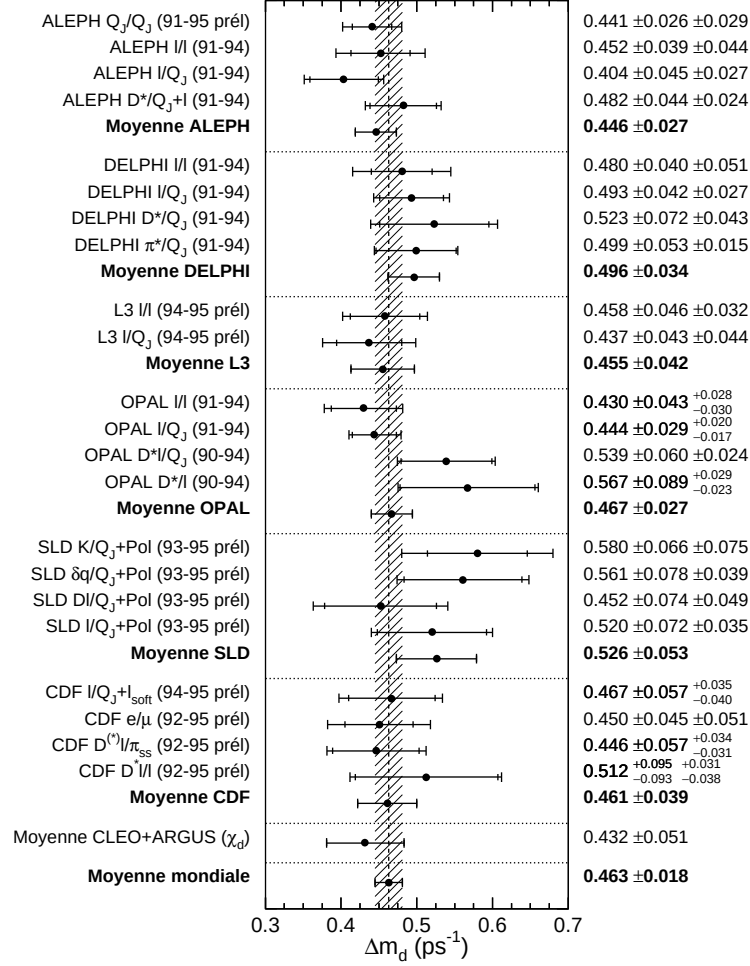
Figure 2.13: Mesures individuelles et combinées de \Delta m_d . Sont indiqués de gauche à droite, le nom de l'expérience, la méthode ( Q_J désigne la charge du jet), les années correspondantes aux données utilisées, la valeur centrale de \Delta m_d ajustée, suivie de ses erreurs statistique et systématique. De nombreux résultats sont préliminaires (prél).
