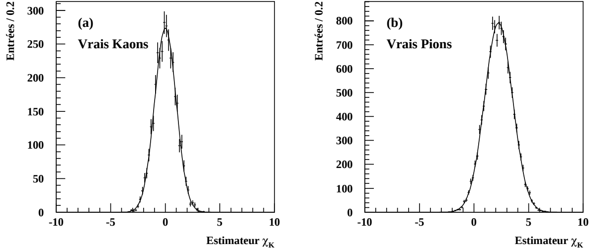
Figure 3.13: Distribution de l'estimateur d'ionisation \chi_K , dans une simulation, pour (a) des vrais kaons et (b) des vrai pions.
