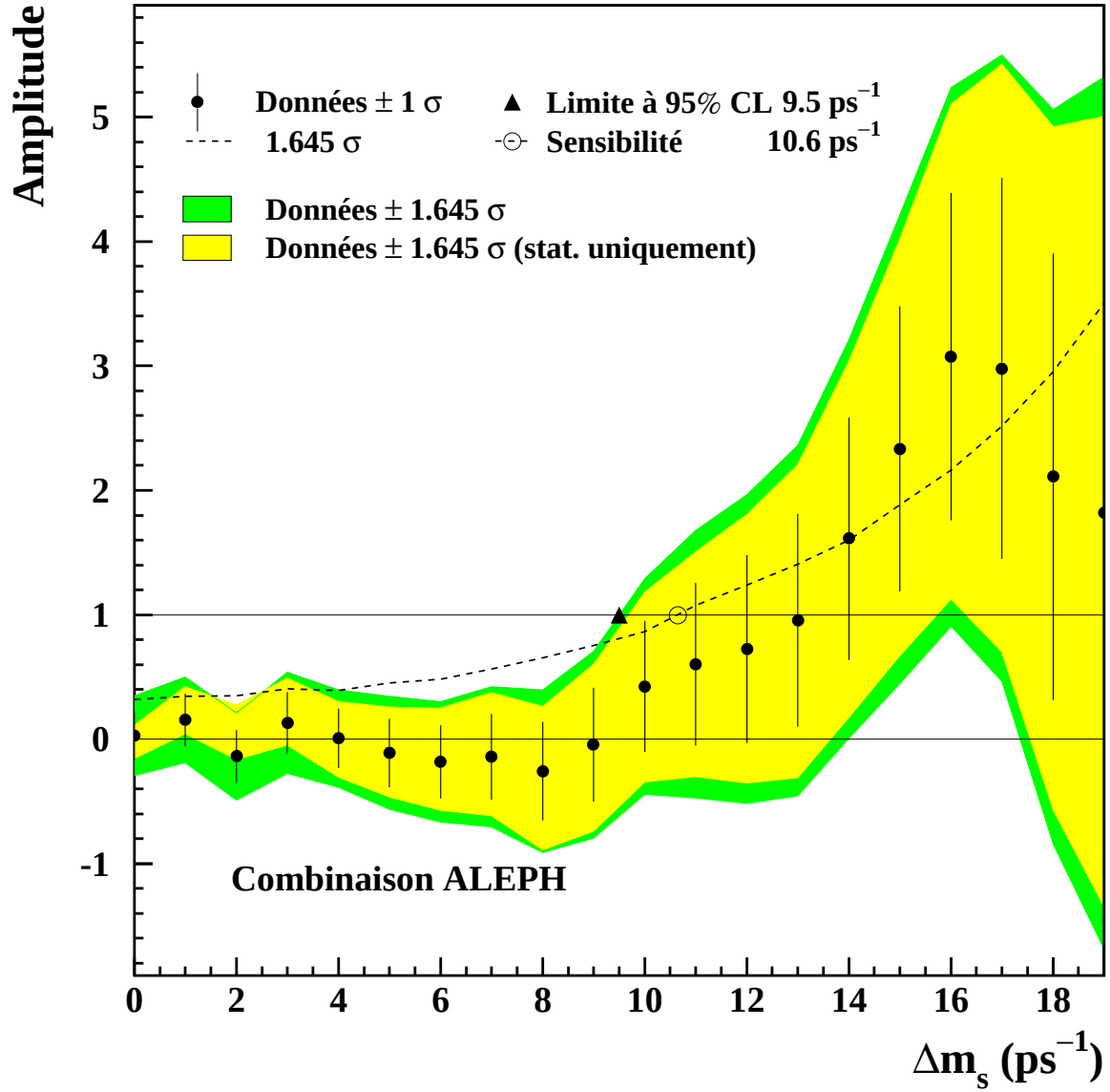
Figure 6.16: Amplitude d'oscillation des B_s^0 mesurée en fonction de \Delta m_s , dans les données, pour la combinaison de notre analyse avec les analyses ALEPH utilisant des D_s^- .
