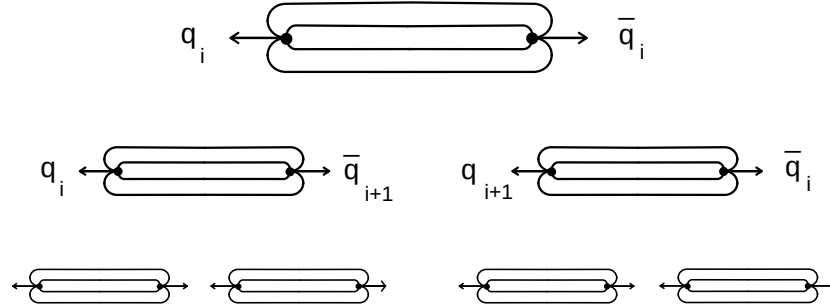
Figure 2.2: Représentation schématique de l'algorithme des cordes utilisé pour simuler la fragmentation.
