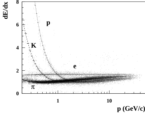
Figure 3.11: Perte d'énergie par ionisation en fonction de l'impulsion, pour différents types de particules. La normalisation est telle que les particules au minimum d'ionisation ont dE/dx=1 . Les courbes superposées sont les prédictions théoriques.
