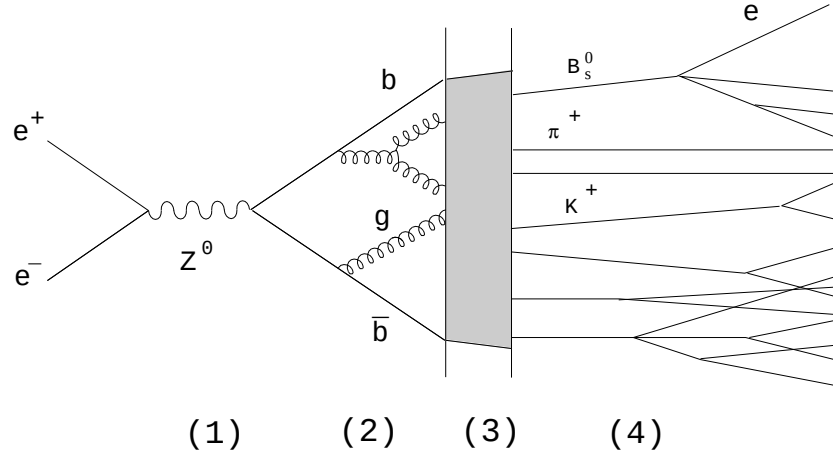
Figure 2.1: Schéma représentant le processus de production des hadrons beaux à partir d'une collision e^+e^- . (1) création de la paire de quarks primaires, (2) rayonnement des partons (quarks et gluons), (3) fragmentation des partons en hadrons, (4) désintégration des hadrons.
