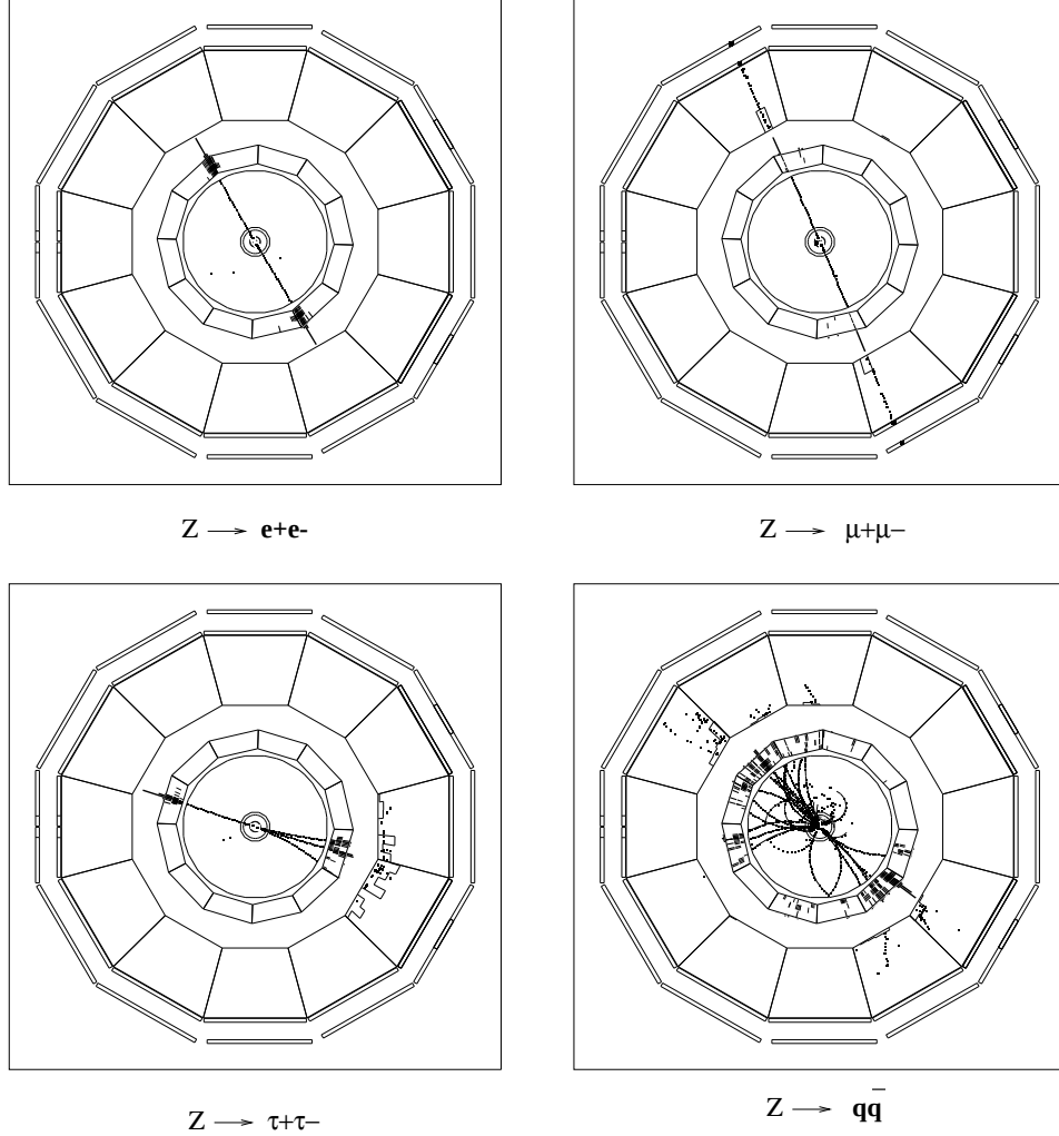
Figure 4.1: Les désintégrations du boson Z^0 observées par le détecteur ALEPH (vue transversale).
