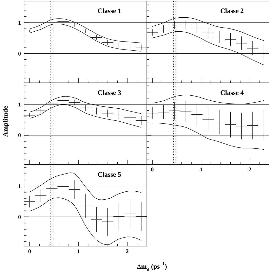
Figure 6.15: Amplitude d'oscillation des B_d^0 mesurée en fonction de \Delta m_d dans les cinq classes d'étiquetages , dans les données. Les lignes pointillées verticales correspondent à la valeur ajustée de \Delta m_d dans tout l'échantillon, par la méthode du maximum de vraisemblance : \Delta m_d = 0.457 \pm 0.024 \text{ ps}^{-1} . Les barres d'erreur représentent l'incertitude statistique à 1\sigma et les courbes en trait plein les contours d'exclusion à 95% CL (sans les incertitudes systématiques).
