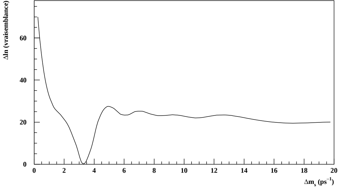
Figure 6.3: \Delta \ln \mathcal{L} en fonction de \Delta m_s , dans le Monte-Carlo (voir le texte). La valeur engendrée de \Delta m_s est 3.33 \text{ ps}^{-1} .
