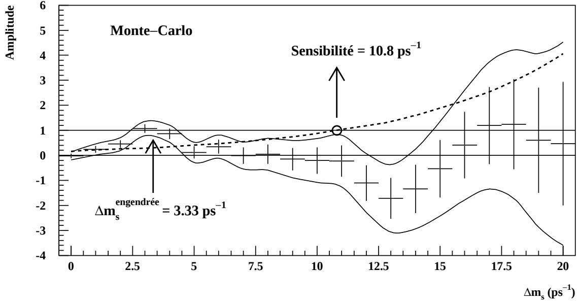
Figure 6.7: Amplitude d'oscillation des B_s^0 mesurée en fonction de \Delta m_s , dans le Monte-Carlo. Les barres d'erreur représentent l'incertitude totale à 1\sigma et les courbes en trait plein les contours d'exclusion à 95% CL (sans les incertitudes systématiques). La courbe discontinue correspond à 1.645\sigma . La valeur engendrée est \Delta m_s = 3.33 \text{ ps}^{-1} .
