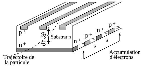
Figure 3.6: Détail de fonctionnement du VDET.
