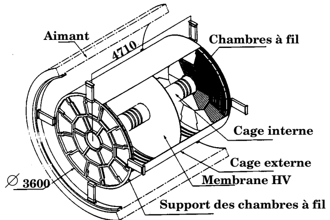
Figure 3.8: La chambre à projection temporelle.
