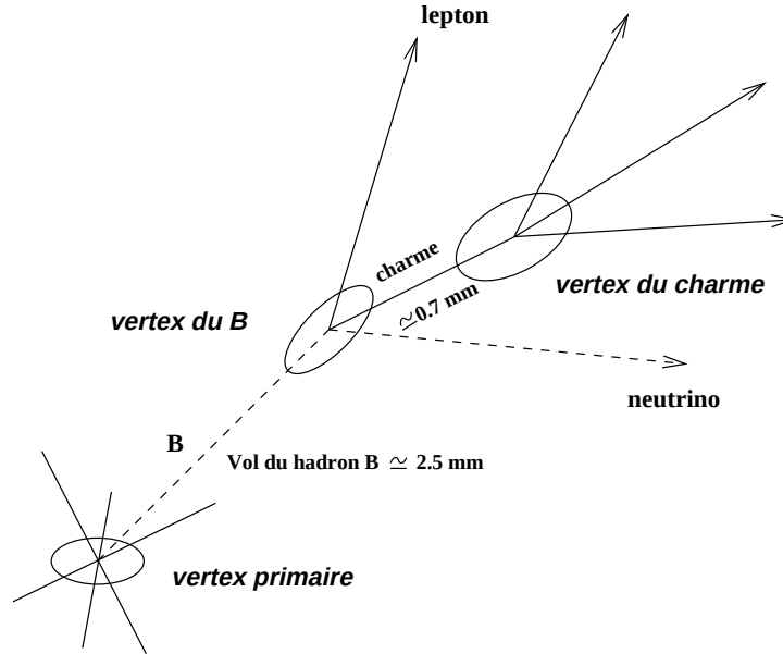
Figure 4.3: Représentation schématique d'une désintégration semi-leptonique typique d'un hadron B .
