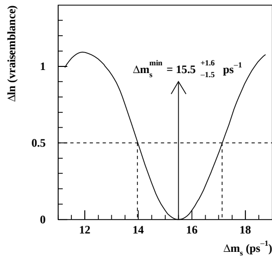
Figure 6.5: \Delta \ln \mathcal{L} en fonction de \Delta m_s , agrandissement de la figure 6.4, dans la région du minimum global. La valeur préférée de \Delta m_s est 15.5^{+1.6}_{-1.5} \text{ ps}^{-1} , mais la profondeur du minimum n'est que de 1.16 unités, soit 1.5\sigma .
