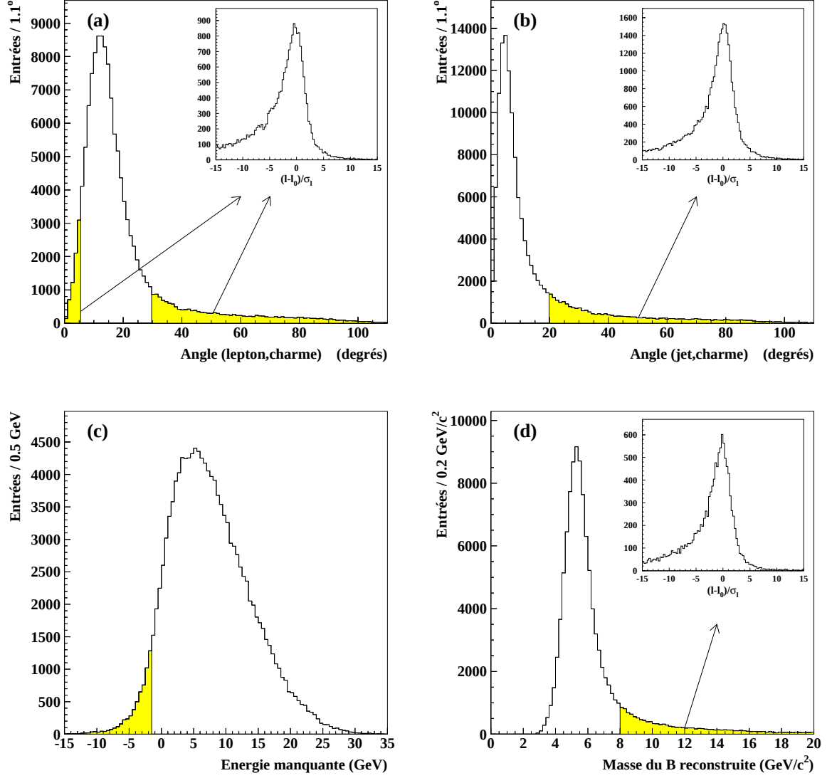
Figure 4.11: Dans la simulation, exemples de grandeurs physiques permettant d'éliminer les événements douteux. Les portions grisées correspondent aux coupures effectuées. Les histogrammes insérés montrent la résolution normalisée sur la longueur de vol des événements rejetés (l'échelle verticale est en nombre d'entrées par 0.3).
