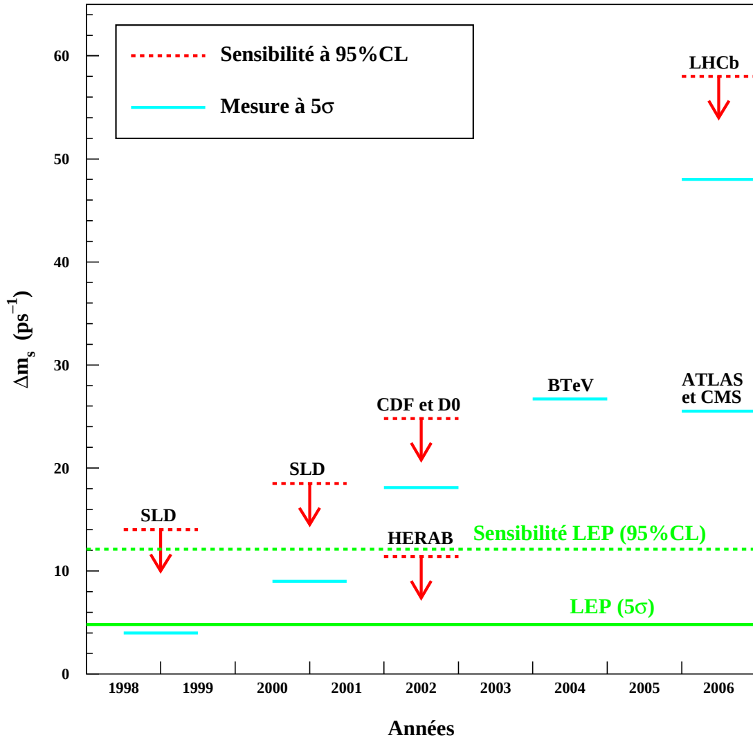
Figure 6.19: Pronostics sur les futures mesures de \Delta m_s . Les chiffres fournis par les différentes expériences mentionnées ne sont pas toujours rigoureusement comparables. Les lignes en trait plein correspondent à une mesure à 5\sigma et les traits discontinus, à une à la sensibilité à 95% CL. Les lignes “LEP (5σ)” et “sensibilité LEP (95 %CL)” correspondent aux résultats présentés dans ce mémoire (§6.5.1).
