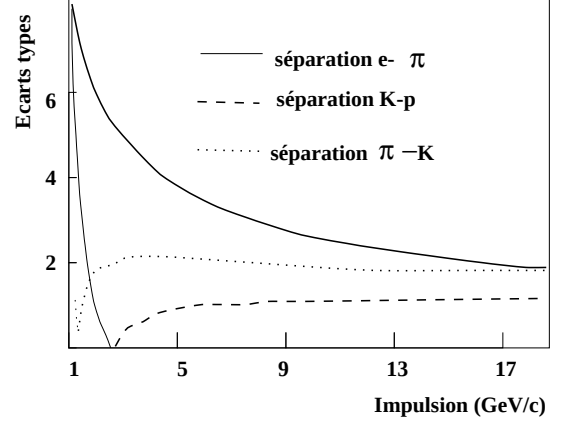
Figure 3.12: Différences attendues de dE/dx , en nombre d'écart types, pour plusieurs couples de particules en fonction de leur impulsion.
