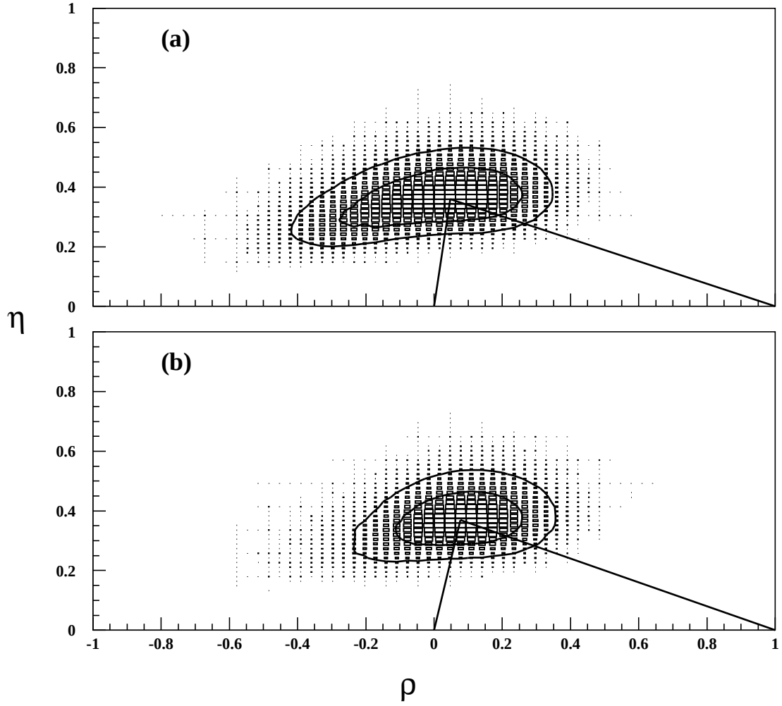
Figure 1.5: Densité de probabilité de (\rho, \eta) , en supposant les erreurs théoriques gaussiennes, (a) sans utiliser l'information sur \Delta m_s et (b) avec la contrainte \Delta m_s > 9.5 \text{ ps}^{-1} à 95% CL. Les contours dessinés correspondent à 68% et 95% de niveau de confiance.
