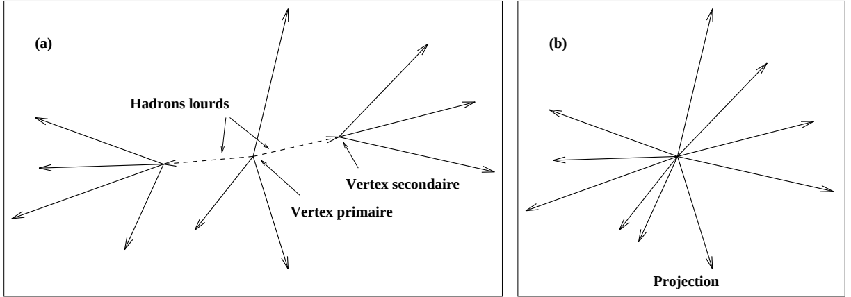
Figure 4.4: Schéma de principe de la recherche du vertex primaire. (a) Exemple d'événement avec désintégrations de hadrons lourds. (b) Après projection le long de la direction des hadrons lourds, toutes les particules semblent provenir du même point.
