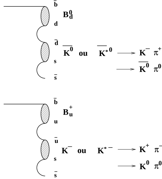
Figure 2.10: Processus pouvant créer un kaon de fragmentation, sans qu'un méson B_s^0 ne soit présent dans l'événement.
