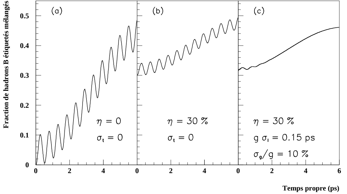
Figure 2.14: Visibilité des oscillations en fonction des paramètres clés de l'étude du mélange (voir le texte).
