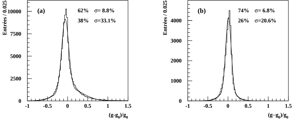
Figure 4.9: Résolution relative sur le terme de poussée, en utilisant l’algorithme de jet nucléé; (a) après la présélection, (b) après l’élimination des événements douteux (§4.4). Les histogrammes sont ajustés par la somme de deux gaussiennes dont les fractions et les écarts types sont indiqués.
