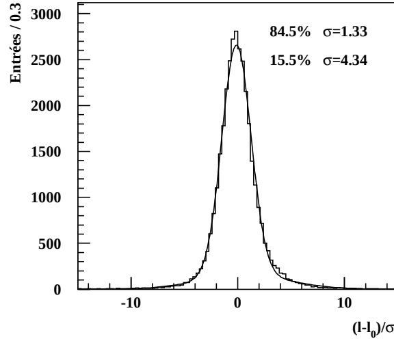
Figure 4.10: Résolution normalisée sur la longueur de vol, après toutes les coupures (à comparer avec fig. 4.6). L’histogramme est ajusté par la somme de deux gaussiennes dont les fractions et les écarts types sont indiqués.
