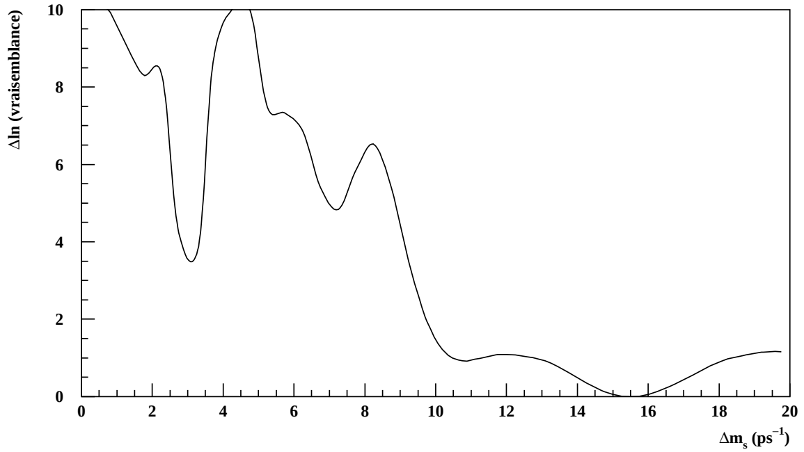
Figure 6.4: \Delta \ln \mathcal{L} en fonction de \Delta m_s , dans les données (voir le texte).
