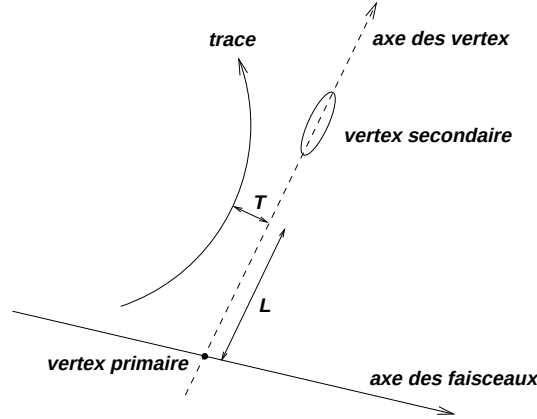
Figure 2.6: Définitions des quantités utilisées dans le calcul de la charge du dipôle, par l'expérience SLD.
