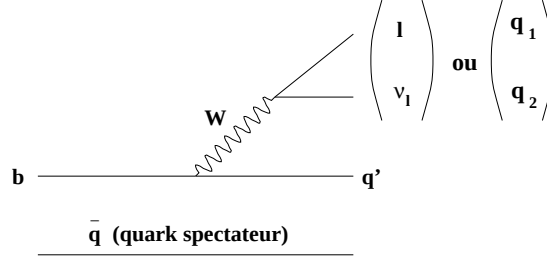
Figure 2.4: Désintégration d'un méson B ( \sim b\bar{q} ) par processus spectateur.
