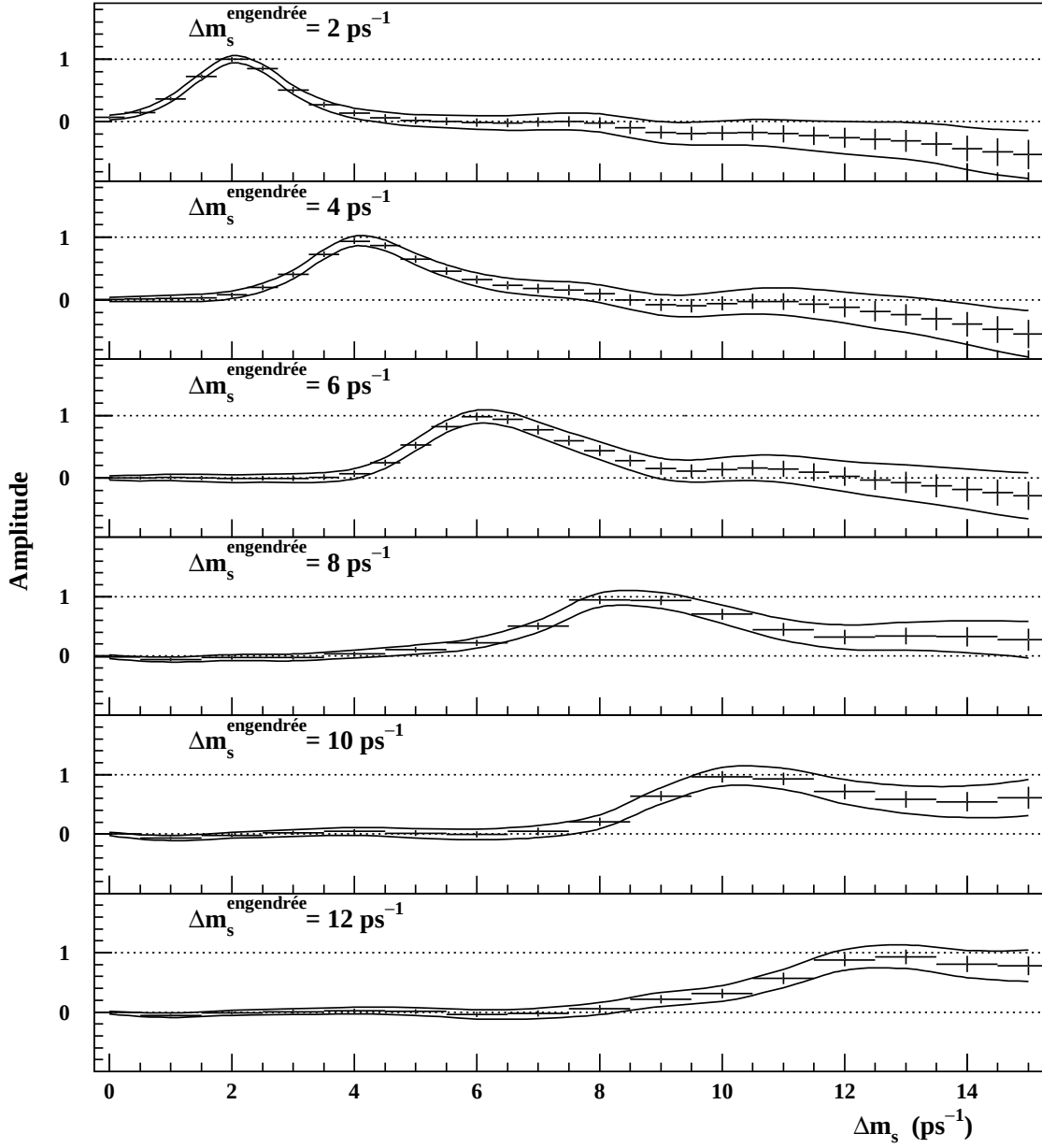
Figure 6.10: Amplitude d'oscillation des B_s^0 mesurée en fonction de \Delta m_s , dans des échantillons Monte-Carlo simplifiés, engendrés avec \Delta m_s^{\text{engendrée}}=2, 4, 6, 8, 10 , et 12 \text{ ps}^{-1} . Les barres d'erreur représentent l'incertitude statistique à 1\sigma et les courbes en trait plein les contours d'exclusion à 95% CL.
