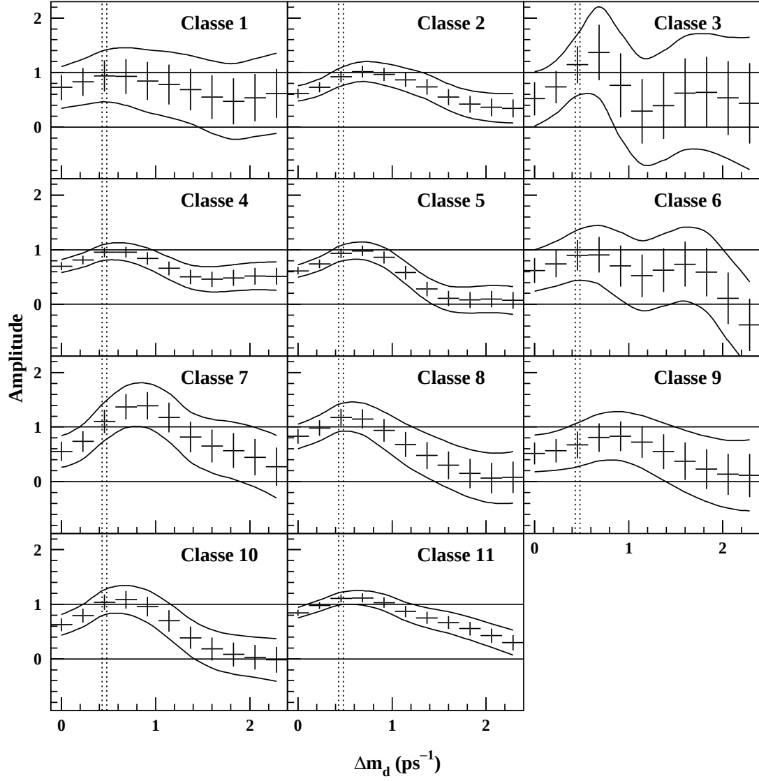
Figure 6.14: Amplitude d'oscillation des B_d^0 mesurée en fonction de \Delta m_d dans les onze classes de puretés , dans les données. Les lignes pointillées verticales correspondent à la valeur ajustée de \Delta m_d dans tout l'échantillon, par la méthode du maximum de vraisemblance : \Delta m_d = 0.457 \pm 0.024 ps -1 . Les barres d'erreur représentent l'incertitude statistique à 1\sigma et les courbes en trait plein les contours d'exclusion à 95% CL (sans les incertitudes systématiques).
