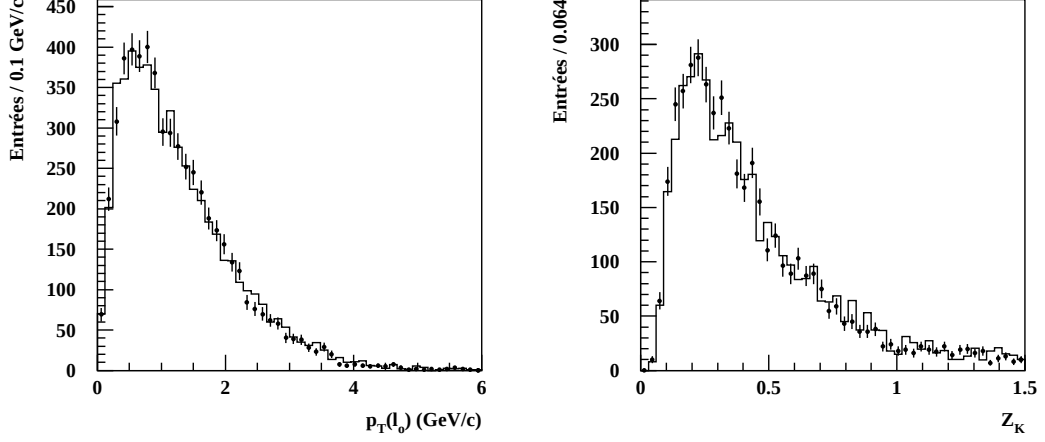
Figure 5.7: Distributions des variables discriminantes p_T(l_o) et Z_K dans les données (points) et le Monte-Carlo (histogrammes).
