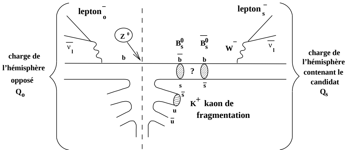
Figure 5.5: Informations utilisées pour étiqueter les saveurs initiale et finale de mésons B_s^0 .
