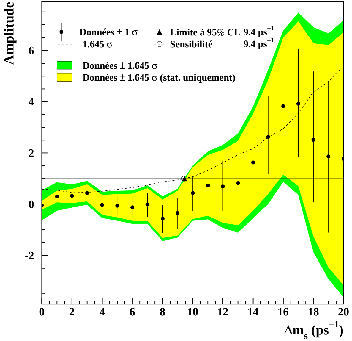
Figure 6.8: Amplitude d'oscillation des B_s^0 mesurée en fonction de \Delta m_s , dans les données. Les barres d'erreur représentent l'incertitude totale à 1\sigma et les bandes grisées montrent les contours d'exclusion à 95% CL avec et sans les incertitudes systématiques.
