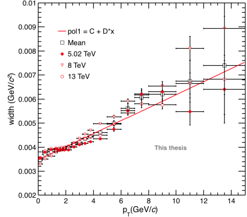
(b) K_S^0 width parameter vs. p_T .
