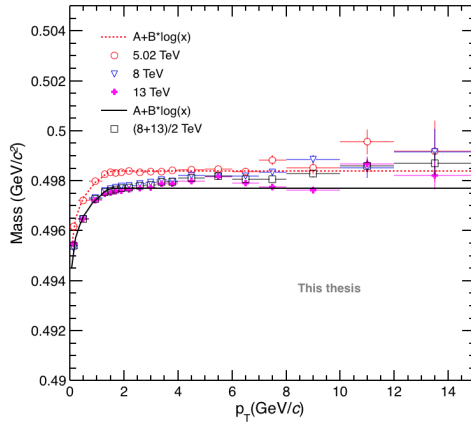
(a) K_S^0 mass parameter vs. p_T .
