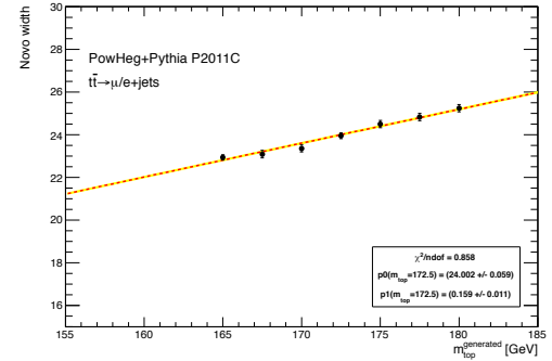
(d) \sigma_{bkg} (background width) fit parameter dependence.
