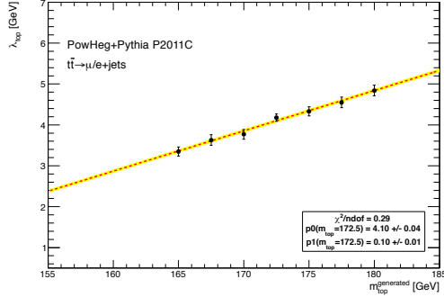
(a) \lambda fit parameter dependence.
