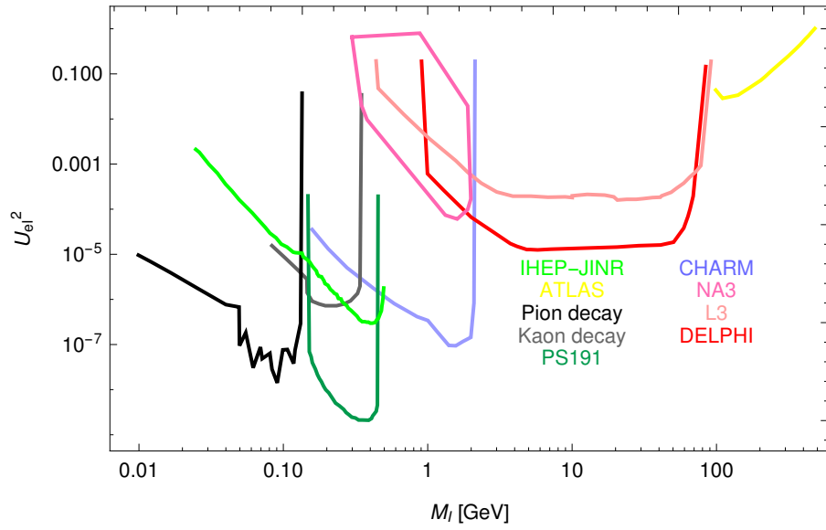
(a) Sensibilité à U_e^2
