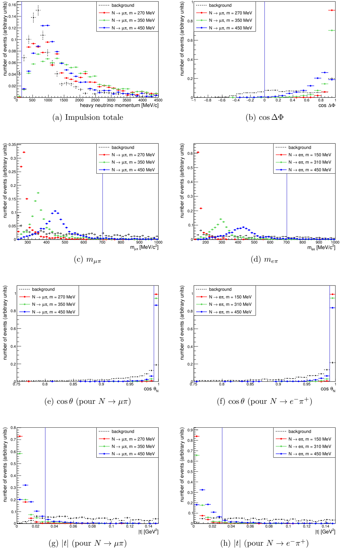
FIGURE 5.11 – Distributions de l'impulsion reconstruite du neutrino lourd, de l'angle entre les deux traces, de la masse invariante, de l'angle polaire et de |t| pour différents échantillons de signal, comparées avec les prédictions pour le bruit de fond restant après les coupures d'identification. Les coupures sont représentées par des lignes bleues verticales et les distributions sont normalisées à l'unité.
