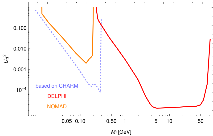
(c) Sensibilité à U_\tau^2
