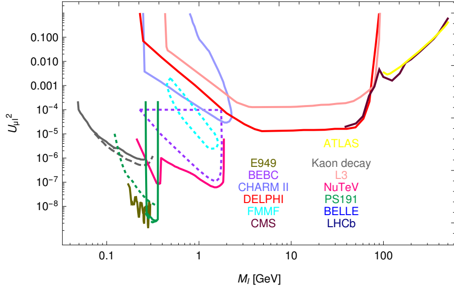
(b) Sensibilité à U_\mu^2
