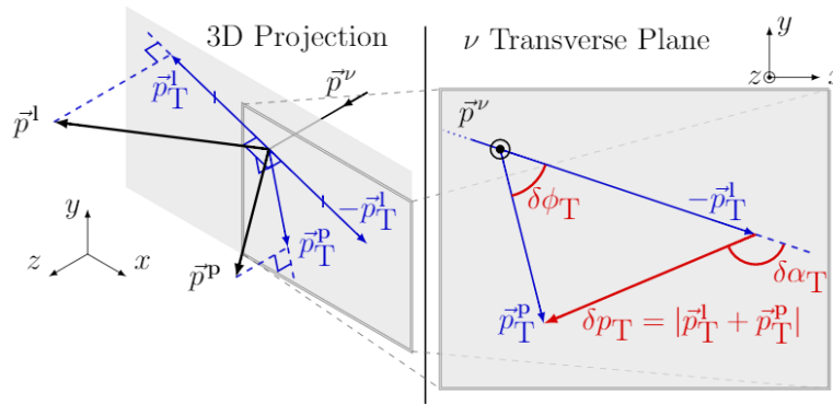
FIGURE 4.3 – Définition des variables cinématiques transverses à partir de la cinématique du muon et du proton. Figure provenant de [91].
