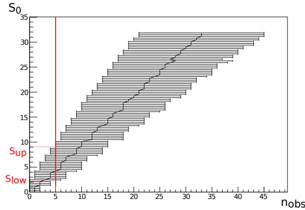
FIGURE 6.2 – Exemple de ceinture de confiance construite avec la méthode de Feldman-Cousins et la fonction de vraisemblance 6.7. Les valeurs numériques utilisées sont : B^0 = 0.67 , \delta B = 0.24 ( \sigma(\eta_B) = 36\% ), \sigma(\eta_S) = 16\% , CL = 90\% . La ligne rouge correspond à une observation de 5 événements dans ces conditions et permet alors de définir un intervalle de confiance à 90% [S_{\text{low}}, S_{\text{up}}] .
