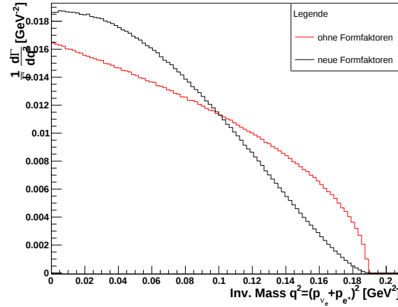
Abbildung 3.7: q^2 -Verteilung des Verzweigungsverhältnisses bei B_c^+ \rightarrow B_s(2) + e^+ + \nu_e
