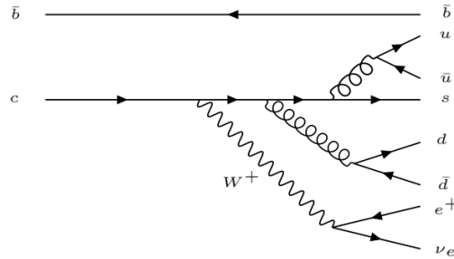
Abbildung 4.1: Beispiel für Feynman Diagramm mit Gluonabstrahlung. Hadronisation kann nun zum Beispiel die Endprodukte \pi^- , B^+ , D_s^- , e^+ , \nu_e ergeben
