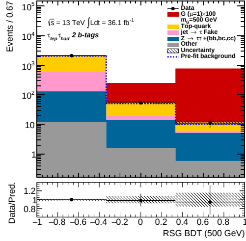
(d) RSG ( m_G = 500 GeV)
