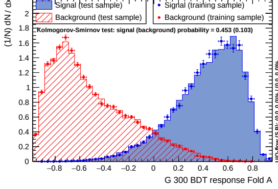
(a) RSG ( m_G = 300 GeV) Fold 1
