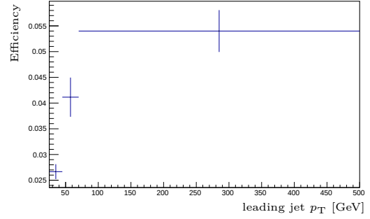
(d) 70 % WP: Efficiency in the case of a muon.
