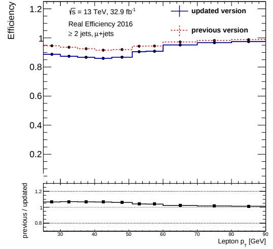
(d) Real efficiency for the \mu + \text{jets} channel.
