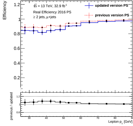
(d) Real efficiency for the \mu + \text{jets} channel.
