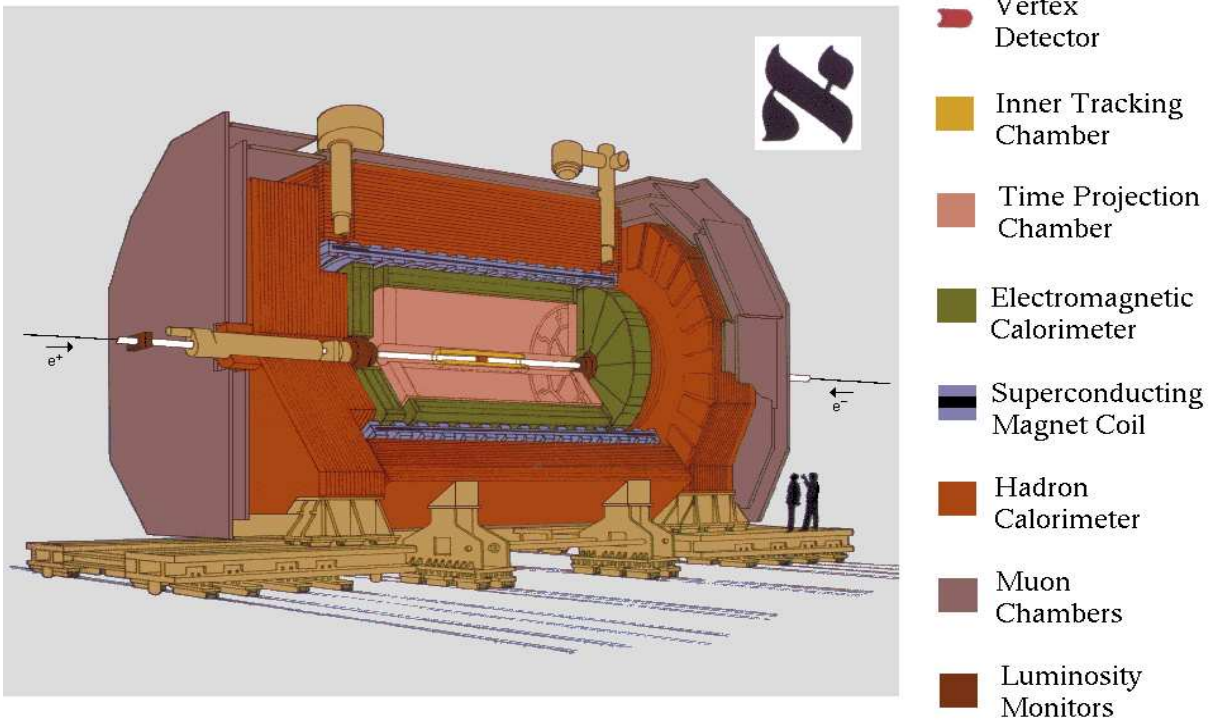
Abbildung 4.3: Querschnitt des ALEPH-Detektors. Man beachte den Größenvergleich mit zwei Menschen am rechten Bildrand.
