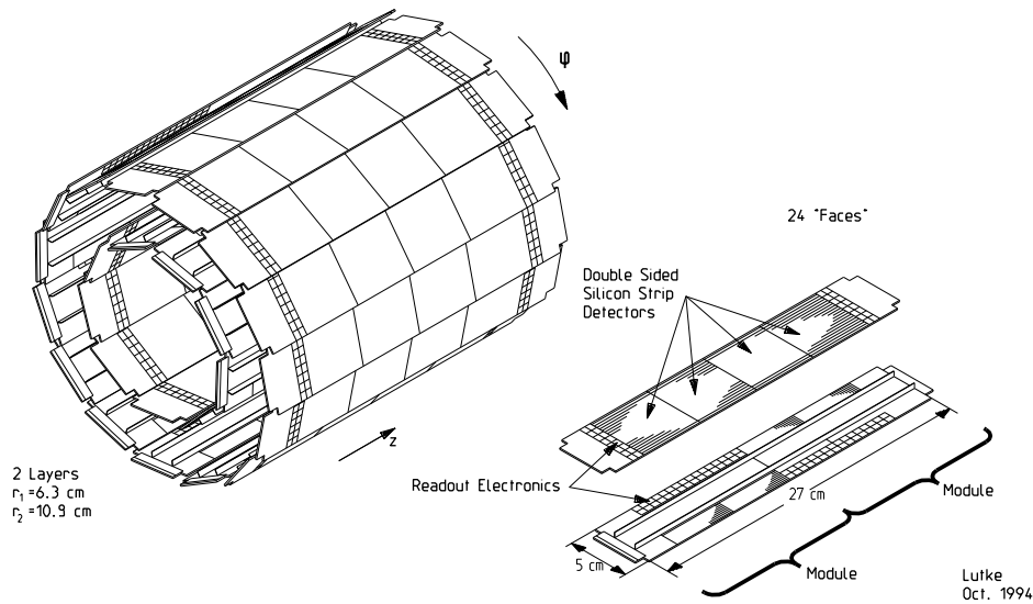
Abbildung 4.4: Der Silizium-Vertexdetektor
