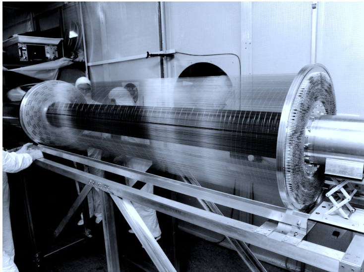
Abbildung 4.5: Gesamtansicht der ITC vor dem Einbau in eine Kohlefaserhülle.
