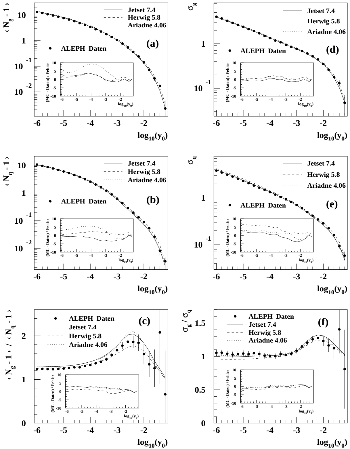
Abbildung 6.1: Mittelwert und Standardabweichung der Subjet-Multiplizitätsverteilung von Gluon- und Quarkjets als Funktion des Subjet-Auflöseparameters y_0 . Die Meßergebnisse für den E_{jet} -integrierten Fall werden mit den Hadronniveaue-Vorhersagen unterschiedlicher MC-Modelle verglichen. In den Unterbildern ist jeweils die Differenz zwischen Modellvorhersage und Daten normiert auf den Gesamtfehler dargestellt.
