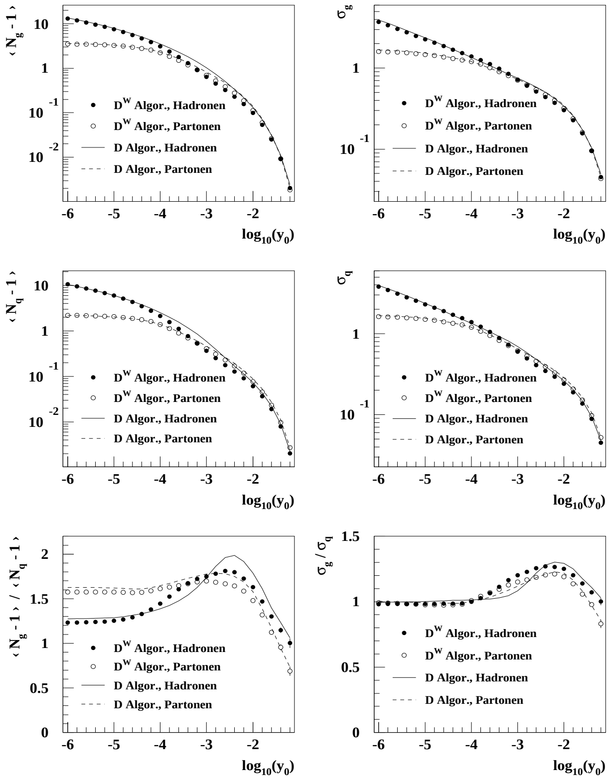
Abbildung B.2: Mittelwert und Breite der Subjet-Multiplizitätsverteilung von Gluon- und Quarkjets als Funktion des Subjet-Auflöseparameters y_0 . Die Meßgrößen auf Parton- und Hadronenniveau für den ‘verbesserten’ Durham-Algorithmus ( D^W ) sind mit denen für den Standard-Durham-Algorithmus (D) verglichen. Diese Bilder beinhalten alle zur Verfügung stehenden Jetenergien.
