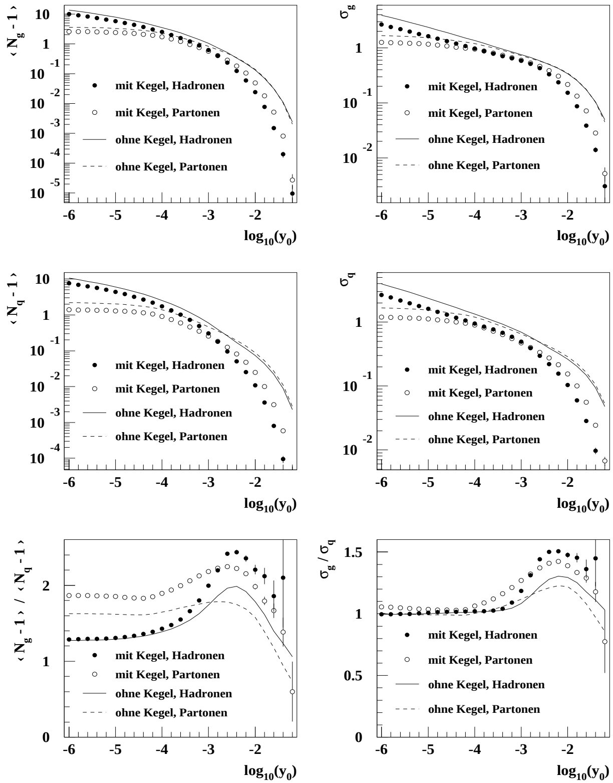
Abbildung C.1: Mittelwert und Breite der Subjet-Multiplizitätsverteilung von Gluon- und Quarkjets als Funktion des Subjet-Auflöseparameters y_0 . Die Meßgrößen auf Parton- und Hadronniveau sind für den Standard-Durham-Algorithmus mit und ohne Verwendung von Akzeptanzkegeln um die Jetachsen verglichen. Diese Bilder beinhalten alle zur Verfügung stehenden Jetenergien.
