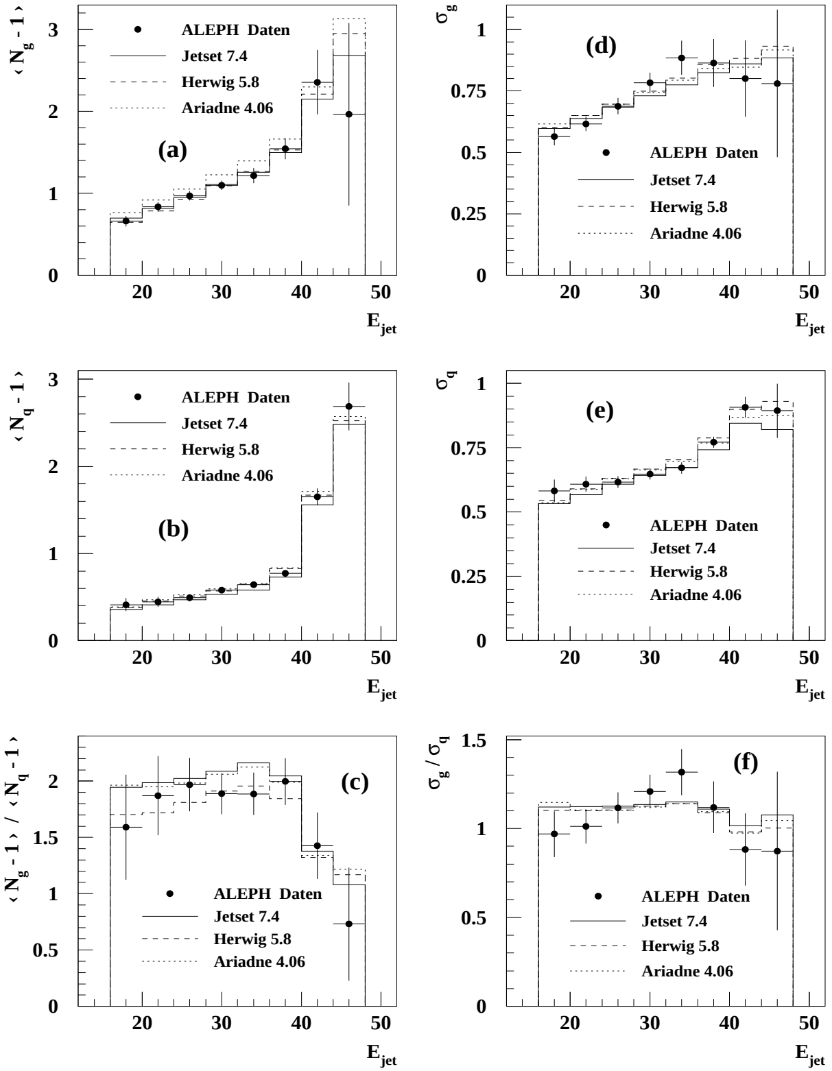
Abbildung 6.5: Mittelwert und Standardabweichung der Subjet-Multiplizitätsverteilung von Gluon- und Quarkjets als Funktion der Jetenergie E_{jet} . Die Meßergebnisse für y_0 = 10^{-3.0} ( \hat{=} k_t \approx 2.9 GeV) werden mit den Hadronniveau-Vorhersagen unterschiedlicher MC-Modelle verglichen.
