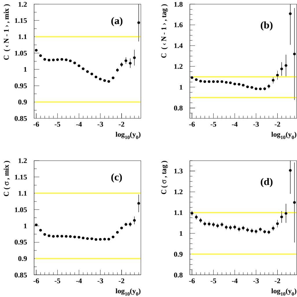
Abbildung 5.5: Detektorkorrekturfaktoren als Funktion von y_0 für den E_{jet} -integrierten Fall: (a) für \langle N-1 \rangle in der gemischten Jetmenge, (b) für \langle N-1 \rangle in der gluonenangereicherten Jetmenge, (c) für \sigma in der gemischten Jetmenge, (d) für \sigma in der gluonenangereicherten Jetmenge. Die horizontalen Linien kennzeichnen Korrekturen von \pm 10\% . Die Fehlerbalken stellen die statistische Unsicherheit dar.
