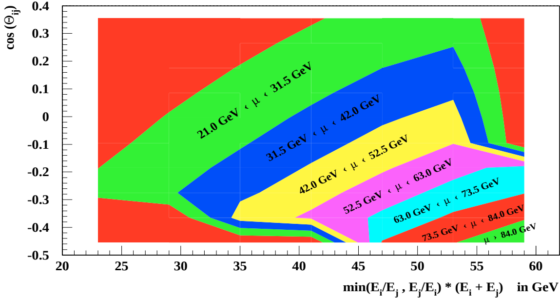
Abbildung D.2: Diese Abbildung zeigt die verschiedenen Ereignisklassen, die zu unterschiedlichen Intervallen der Größe \mu gehören. Auf der x-Achse ist der Energieterm des minimalen k_t im Ereignis für den Durham-Algorithmus mit veränderter Distanzgröße aufgetragen, während auf der y-Achse der Winkelterm \cos \theta_{ij} dargestellt ist. Jedes 3-Jet-Ereignis wird durch einen Punkt in dieser Ebene gekennzeichnet. Die verschiedenen Grautöne zeigen unterschiedliche Intervalle von \mu an 1 . Die Bereiche in der oberen und unteren linken und der oberen rechten Ecke, für die kein Intervall von \mu eingetragen ist, sind für die verwendete Ereignisselektion nicht zugänglich.
