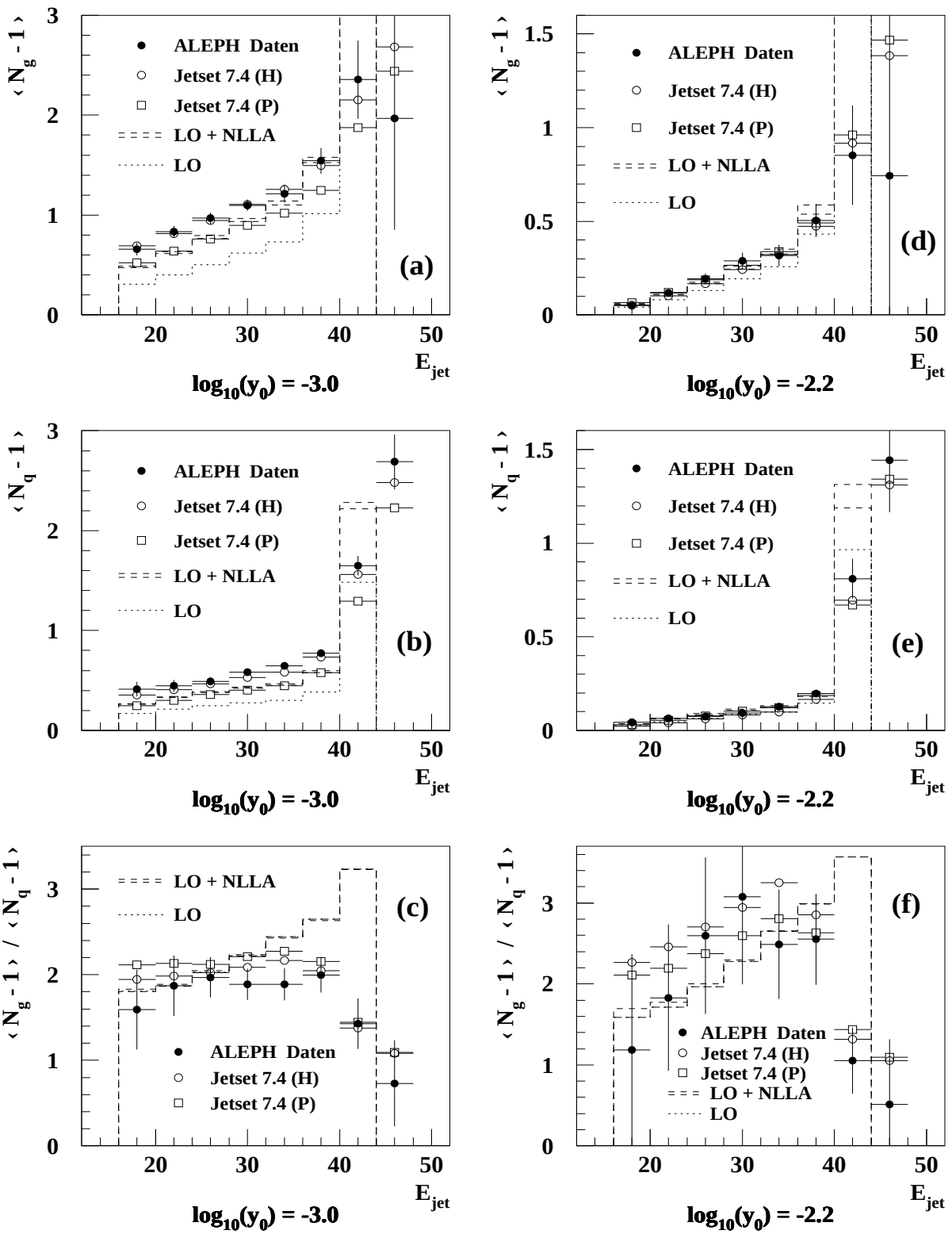
Abbildung 6.9: Die mittlere Subjet-Multiplizität von Gluon- und Quarkjets als Funktion der Jetenergie E_{jet} für y_0 = 10^{-3.0} ( \hat{=} k_t \approx 2.9 GeV) und y_0 = 10^{-2.2} ( \hat{=} k_t \approx 7.2 GeV). Die Meßergebnisse werden mit perturbativen QCD-Vorhersagen (gepunktetes Histogramm für LO und zwei gestichelte Histogramme für LO+NLLA) und dem Hadron- und Partonniveau des Modells Jetset 7.4 verglichen. Die Abweichung der beiden gestichelten Histogramme voneinander ist ein Maß für die theoretische Unsicherheit der LO+NLLA-Vorhersage.
