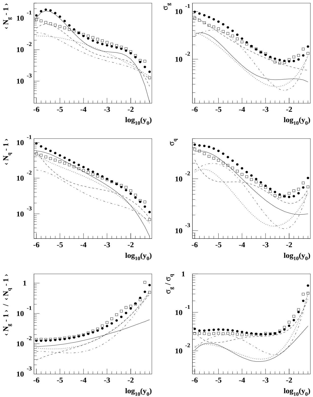
Abbildung 5.6: Die verschiedenen absoluten Beiträge zum gesamten systematischen Fehler der Meßgrößen für den E_{jet} -integrierten Fall als Funktion des Subjet-Auflöseparameters y_0 . Die durchgezogene Linie stellt den Einfluß der Generatorabhängigkeit der Detektorkorrekturfaktoren, die gestrichelte Linie den Einfluß des Schnittes E_{neutral}^{min} , die gepunktete Linie den Einfluß des Schnittes \theta_{jet}^{min} und die strich-punktierte Linie den Einfluß des Schnittes P_{jet}^{cut} dar (siehe Text). Die vollen Punkte geben den gesamten systematischen Fehler wieder und die offenen Quadrate kennzeichnen den absoluten statistischen Fehler.
