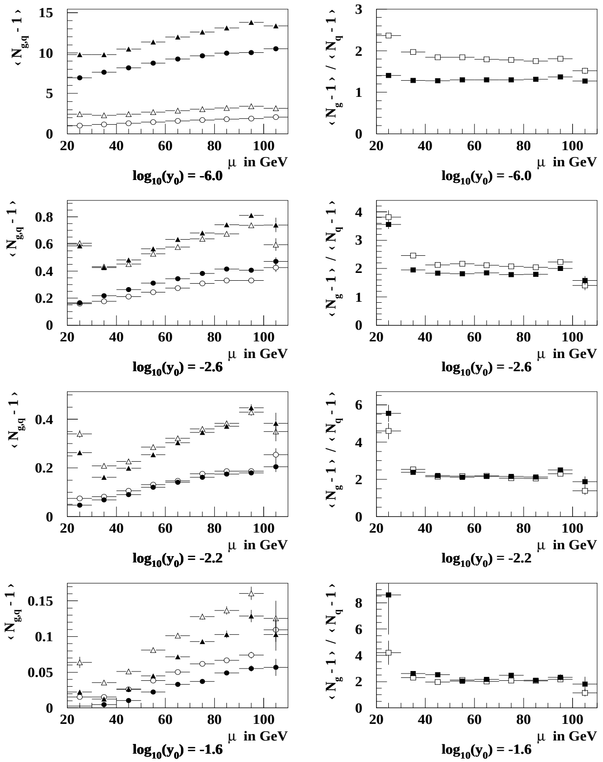
Abbildung D.3: Mittelwert der Subjet-Multiplizitätsverteilung von Gluon- und Quarkjets als Funktion der Größe \mu = k_t^{min}/2 für einzelne Werte von y_0 . Die Meßgrößen auf Hadronniveau (volle Symbole) und Partonniveau (offene Symbole) sind für den Durham-Algorithmus mit veränderter Distanzgröße und Verwendung von Akzeptanzkegeln um die Jetachsen dargestellt. Gluonjets sind durch Dreiecke, Quarkjets durch Kreise und das Verhältnis \frac{Gluon}{Quark} ist durch Quadrate gekennzeichnet.
