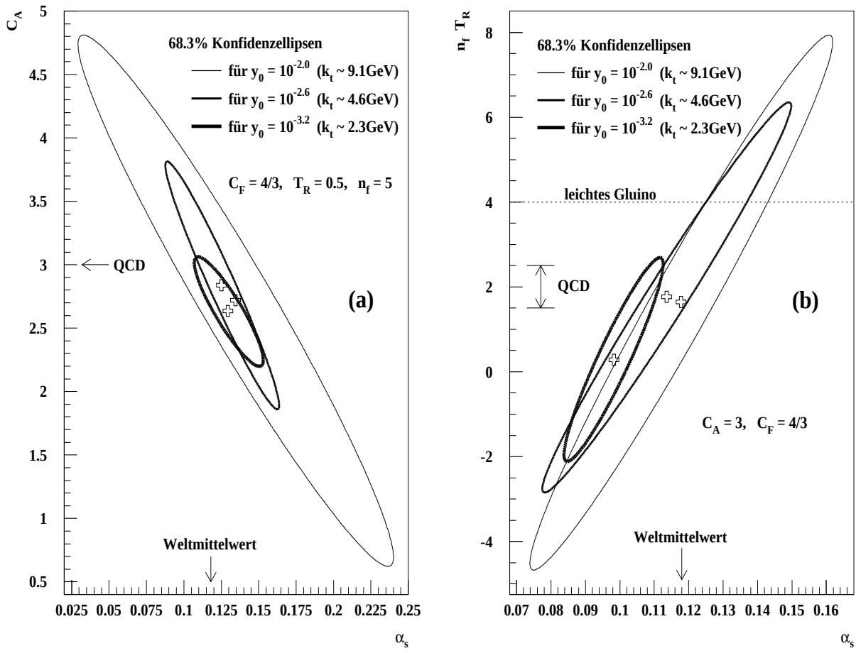
Abbildung 7.1: Die 68.3% Konfidenzellipsen der gemeinsamen Anpassung von (a) C_A und \alpha_s und (b) n_f T_R und \alpha_s für drei verschiedene Werte des Subjet-Auflöseparameters y_0 : y_0 = 10^{-3.2} , y_0 = 10^{-2.6} und y_0 = 10^{-2.0} . Die zugehörigen Werte der transversalen Energie ( k_t \approx \sqrt{y_0} \cdot E_{CM} ) sind ebenfalls angegeben. Die Konfidenzellipsen berücksichtigen die statistischen und systematischen Unsicherheiten.
