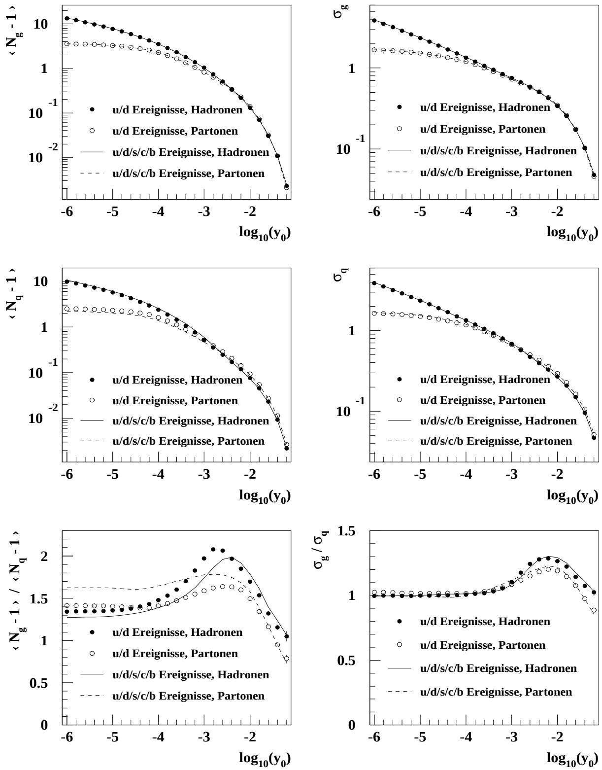
Abbildung A.1: Mittelwert und Breite der Subjet-Multiplizitätsverteilung von Gluon- und Quarkjets als Funktion des Subjet-Auflöseparameters y_0 . Die Meßgrößen auf Parton- und Hadronniveau für Z^0 \rightarrow u\bar{u} und Z^0 \rightarrow d\bar{d} Ereignisse sind mit denen für Ereignisse in der natürlichen Quarkmischung auf der Z^0 -Resonanz verglichen. Diese Bilder beinhalten alle zur Verfügung stehenden Jetenergien.
