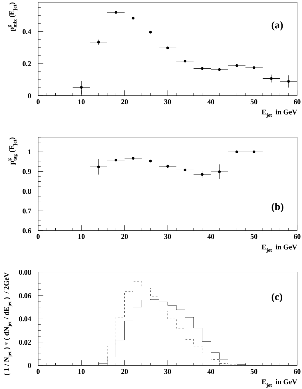
Abbildung 5.4: Die Gluonjetreinheit ist als Funktion der Jetenergie (a) für die gemischte Jetmenge und (b) für die gluonenangereicherte Jetmenge dargestellt. Beide Bilder wurden unter Verwendung simulierter Ereignisse (siehe Abschnitt 5.3) erstellt; die Fehlerbalken zeigen die statistische Unsicherheit der Bestimmung. In Abbildung (c) ist die Jetenergieverteilung der gemischten Menge (durchgezogenes Histogramm) und der gluonenangereicherten Jetmenge (gestricheltes Histogramm) wiedergegeben. Beide Verteilungen wurden aus ALEPH-Daten bestimmt und auf Fläche 1 normiert.
