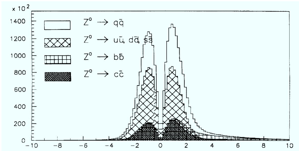
Abbildung 5.1: Verteilung der Stoßparametersignifikanz S = D/\sigma_D für verschiedene Ereignistypen [55]. Die Histogramme wurden unter Verwendung des Jetset-MC-Modells gewonnen. Der b\bar{b} -Anteil ist deutlich im positiven Ausläufer der S -Verteilung zu erkennen.
