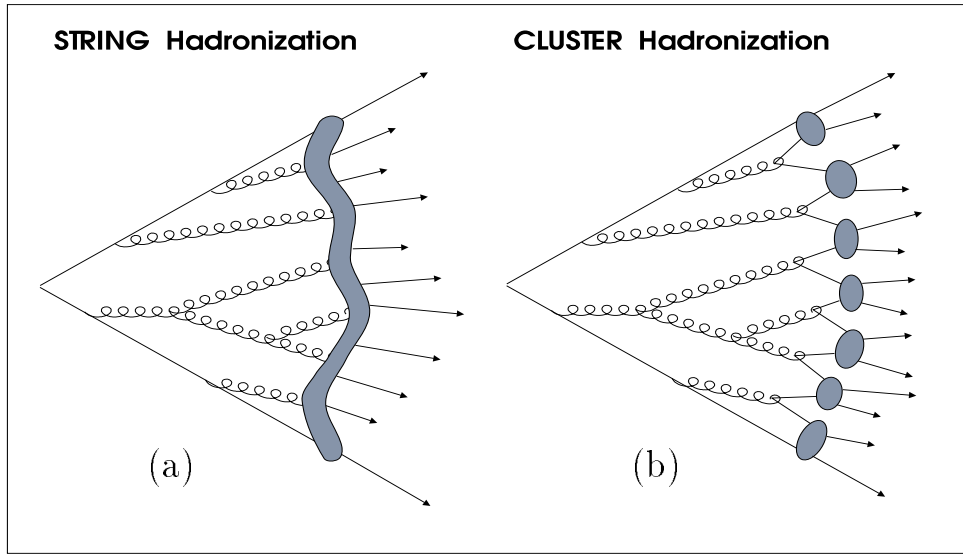
Abbildung 2.3: Unterschiedliche Hadronisierungsmodelle [18]: a) das Stringmodell, b) das Clustermodell.
