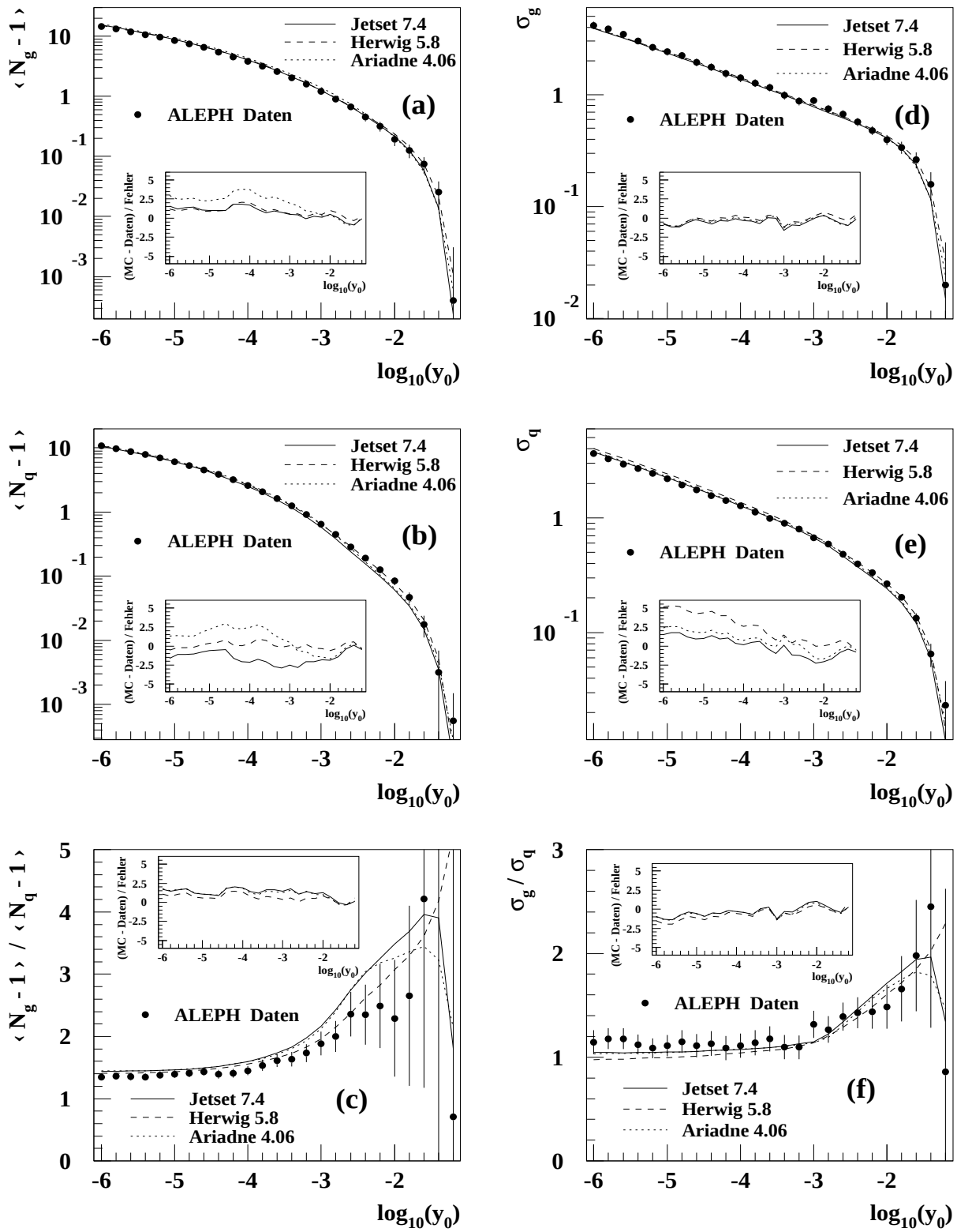
Abbildung 6.3: Mittelwert und Standardabweichung der Subjet-Multiplizitätsverteilung von Gluon- und Quarkjets als Funktion des Subjet-Auflöseparameters y_0 . Die Meßergebnisse für das Jetenergieintervall 32 \text{ GeV} \leq E_{jet} \leq 36 \text{ GeV} werden mit den Hadronniveaue Vorhersagen unterschiedlicher MC-Modelle verglichen. In den Unterbildern ist jeweils die Differenz zwischen Modellvorhersage und Daten normiert auf den Gesamtfehler dargestellt.
