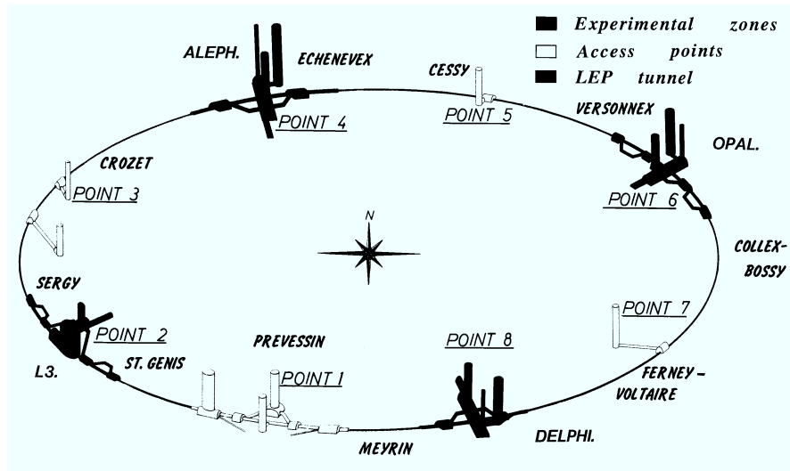
Abbildung 4.2: Der LEP-Speicherring und seine Installationen [46].
