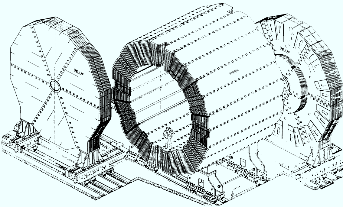
Abbildung 4.8: Perspektivische Sicht des HCAL. Man beachte den Größenvergleich mit dem Menschen im Inneren des Detektors.
