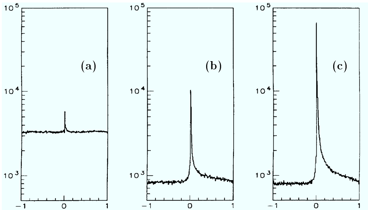
Abbildung 5.2: P_T -Häufigkeitsverteilung für verschiedene Ereignistypen [55]: (a) für Z^0 \rightarrow u\bar{u}, d\bar{d}, s\bar{s} , (b) für Z^0 \rightarrow c\bar{c} und (c) für Z^0 \rightarrow b\bar{b} . Die Verteilungen wurden unter Verwendung des Jetset-MC-Modells gewonnen.
