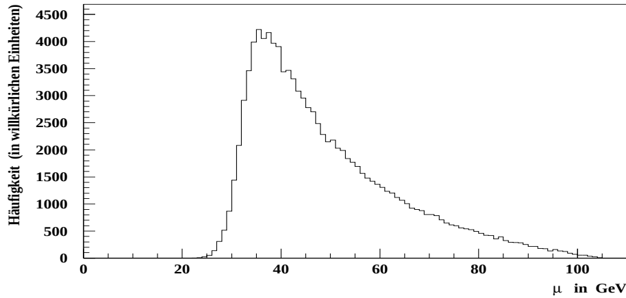
Abbildung D.1: Verteilung der Größe \mu = k_t^{min}/2 auf Hadronniveau für den Durham-Algorithmus mit veränderter Distanzgröße ( 2 \cdot 10^6 Ereignisse).
