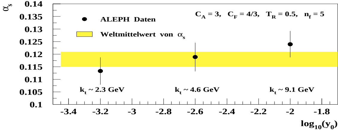
Abbildung 7.2: Die Ergebnisse der Anpassung der Kopplungsstärke \alpha_s für drei verschiedene Werte von y_0 : 10^{-3.2} , 10^{-2.6} und 10^{-2.0} . Die zugehörigen Werte der transversalen Energie k_t sind ebenfalls angegeben. Das graue Band zeigt den Weltmittelwert von \alpha_s mit seinem Fehler. Die Fehler der Meßpunkte schließen statistische und systematische Unsicherheiten ein.
