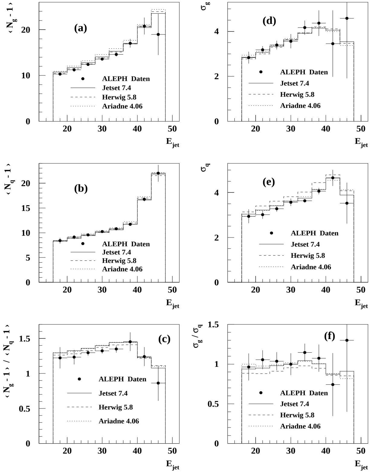
Abbildung 6.4: Mittelwert und Standardabweichung der Subjet-Multiplizitätsverteilung von Gluon- und Quarkjets als Funktion der Jetenergie E_{jet} . Die Meßergebnisse für y_0 = 10^{-6.0} ( \hat{=} k_t \approx 0.1 GeV) werden mit den Hadronniveau-Vorhersagen unterschiedlicher MC-Modelle verglichen.
