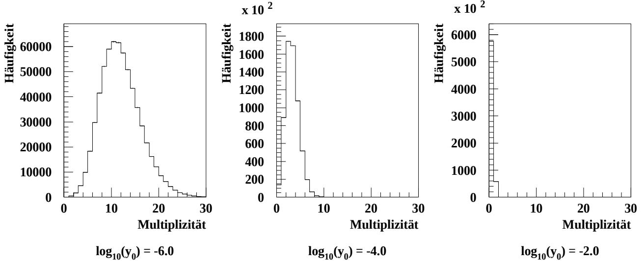
Abbildung 3.2: Subjet-Multiplizitätsverteilung (N - 1) für verschiedene Werte des Subjet-Auflösparameters y_0 . Dargestellt ist die Vorhersage des MC-Modells Jetset 7.4 für alle Jets in 3-Jet-Ereignissen, die mit einem Auflösparameter y_{cut} = y_1 = 0.1 selektiert wurden.
