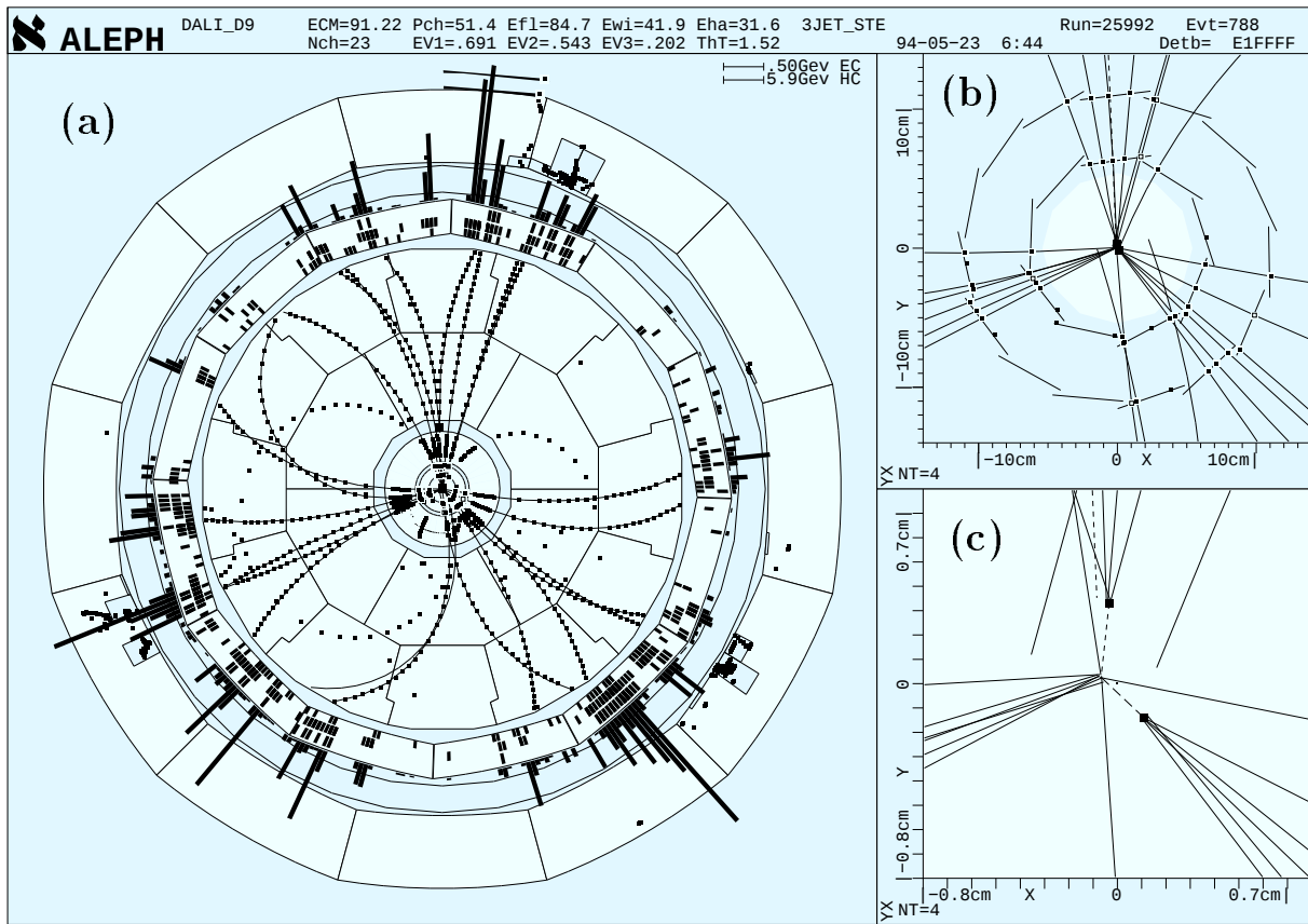
Abbildung 3.1: Ein Beispiel für ein 3-Jet-Ereignis aus den ALEPH-Daten. Alle drei Teilbilder zeigen die Projektion des Ereignisses in die Ebene senkrecht zur Strahlachse 1 . Bild (a) gibt die Gesamtansicht des Detektors wieder, wobei der Maßstab so verzerrt ist, daß die inneren Spurdetektoren größer dargestellt sind. Die beiden äußeren Ringe mit Balkendiagrammen zeigen das elektromagnetische und das hadronische Kalorimeter. In der Mitte des Bildes sind die zwei Lagen des Silizium-Vertexdetektors dargestellt. Dieser ist von einer zylindrischen Drahtkammer (ITC) umgeben, die bis zu acht Messungen pro Spur durchführen kann. Daran schließt sich ein großes Driftvolumen (TPC) an, das sich bis zum elektromagnetischen Kalorimeter erstreckt und bis zu 21 Spurmeßpunkte liefert. Am oberen Bildrand zeigen sich außerhalb des hadronischen Kalorimeters noch zwei Meßpunkte in den Myonkammern. Bild (b) stellt eine Vergrößerung der Messungen des Vertexdetektors dar. Eine weitere Vergrößerung des zentralen Bereichs um den nominellen Wechselwirkungspunkt ist in Bild (c) wiedergegeben. In allen drei Bildern ist klar die mercedessternartige Struktur des Ereignisses zu erkennen ( y_{ij}^{min} \approx 0.259 ). Für zwei der Jets im Ereignis konnte ein deutliches Signal für schwere Hadronen mit langer Lebensdauer nachgewiesen werden. Deren wahrscheinliche Zerfallsvertices sind in Bild (c) durch zwei kleine Quadrate dargestellt. Die auf diese Weise gekennzeichneten Jets stellen Quarkjetkandidaten dar, während der dritte Jet mit hoher Wahrscheinlichkeit durch ein energiereiches Gluon initiiert wurde. Die gestrichelte Linie, die in Bild (c) beginnt und sich in Bild (b) fortsetzt, kennzeichnet die Flugrichtung eines weiteren neutralen Teilchens, das erst im Übergang zwischen ITC und TPC eine Wechselwirkung zeigt (Quadrat in Bild (a)); weiter außen sind dann zwei Spuren geladener Teilchen sichtbar. Hierbei könnte es sich um ein Photon handeln, das in der Innenwand der TPC ein e^+e^- -Paar erzeugt.
