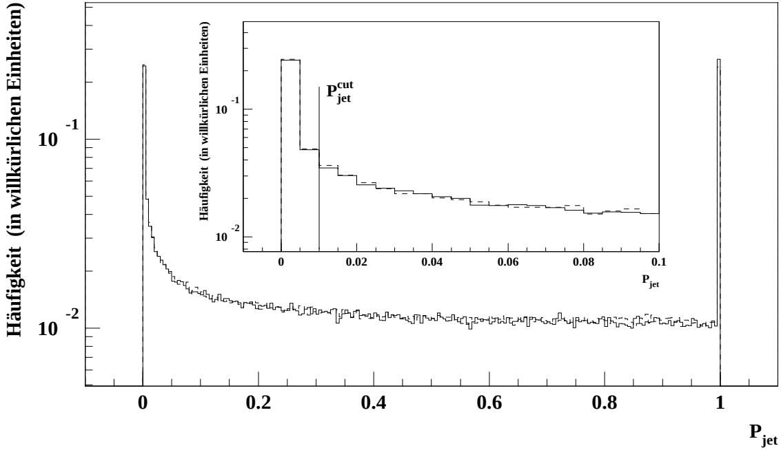
Abbildung 5.3: P_{jet} -Häufigkeitsverteilung für ALEPH-Daten (durchgezogene Linie) und simulierte ALEPH-Ereignisse (gestrichelte Linie, siehe Abschnitt 5.3). Die Verteilungen sind auf die gleiche Anzahl akzeptierter 3-Jet-Ereignisse normiert. In dem Unterbild ist ein Ausschnitt der Verteilungen vergrößert dargestellt. Dort ist auch der Schnitt zur Selektion von Gluonjetkandidaten angedeutet (siehe Abschnitt 5.2.2).
