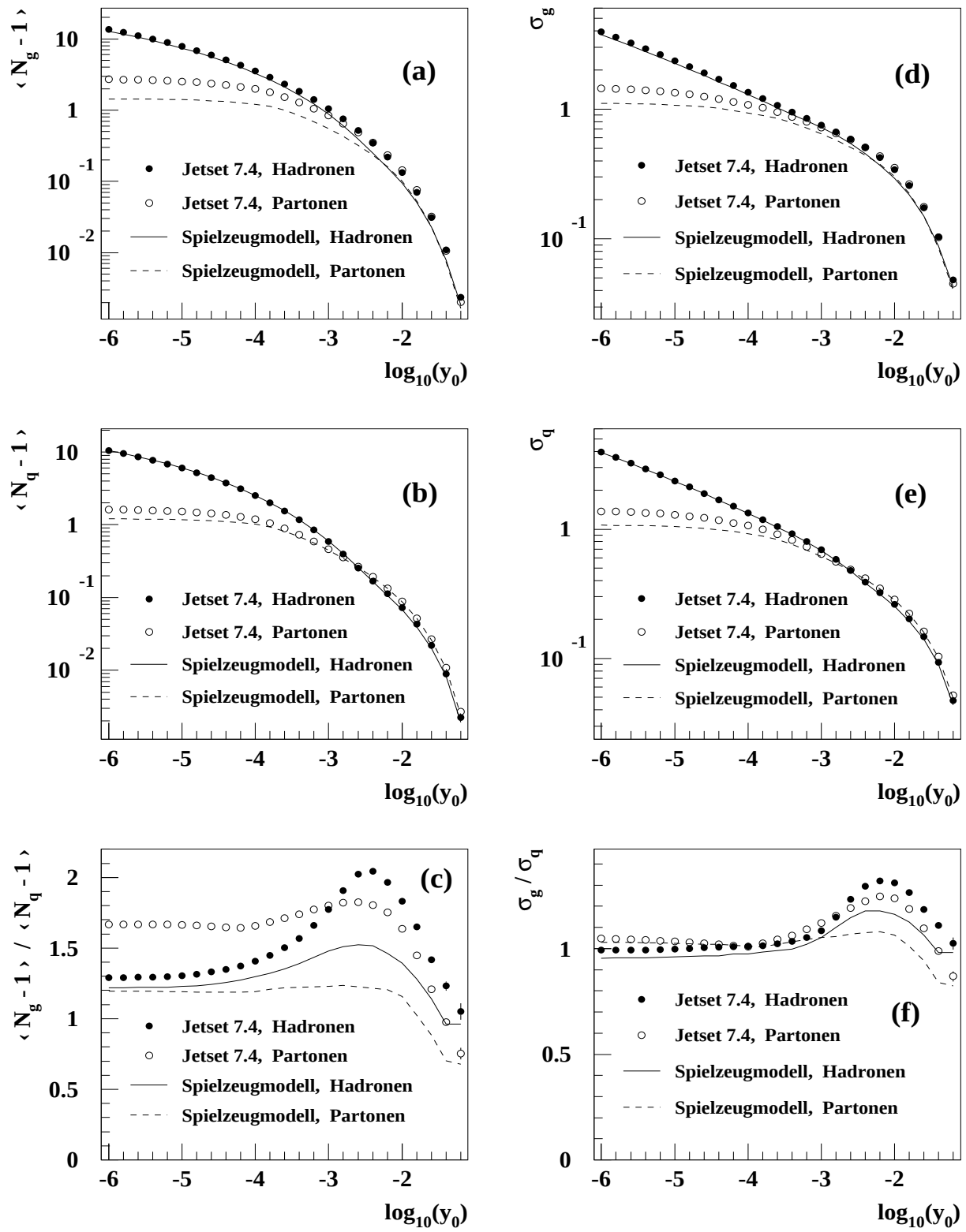
Abbildung 3.3: Mittelwert und Breite der Subjet-Multiplizitätsverteilung von Gluon- und Quarkjets als Funktion des Subjet-Auflöseparameters y_0 . Die Vorhersagen für die Meßgrößen auf Hadron- und Partonniveau werden für das MC-Modell Jetset 7.4 und ein Spielzeugmodell (gleiche effektive Kopplung der Vertices g \rightarrow gg und q \rightarrow qg , siehe Text) miteinander verglichen. Diese Bilder beinhalten alle zur Verfügung stehenden Jetenergien.
