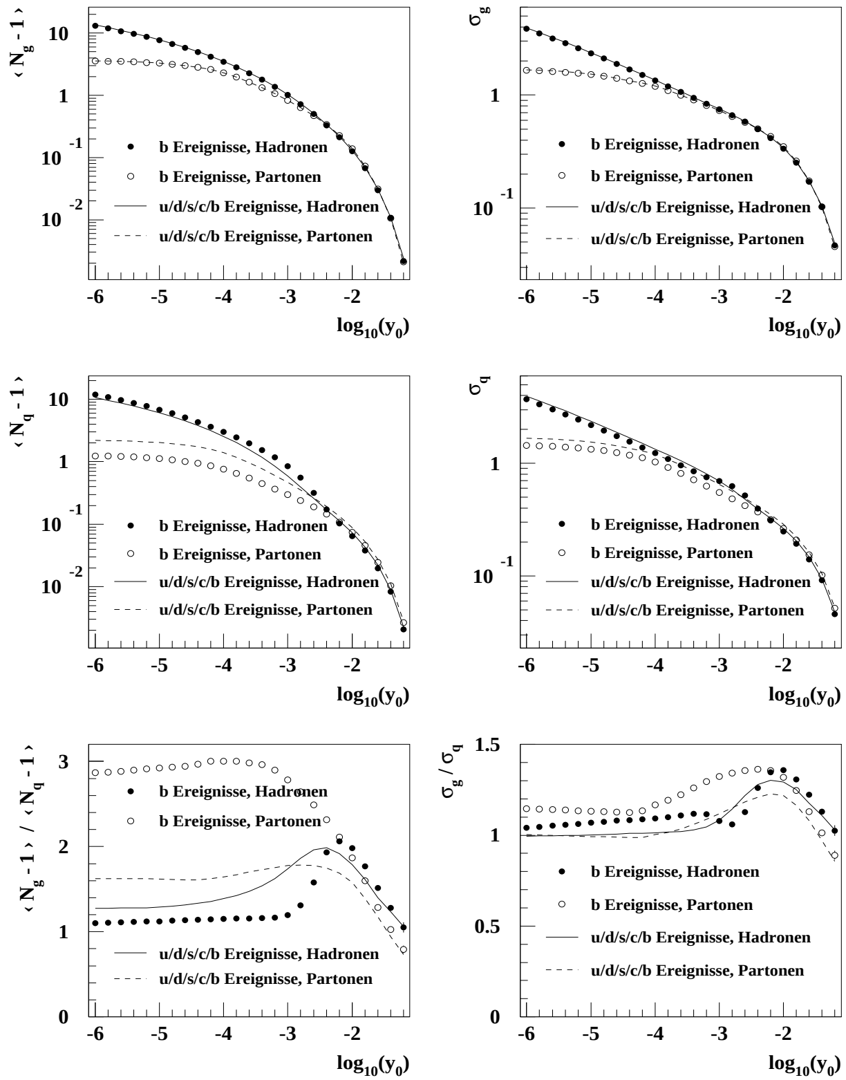
Abbildung A.2: Mittelwert und Breite der Subjet-Multiplizitätsverteilung von Gluon- und Quarkjets als Funktion des Subjet-Auflöseparameters y_0 . Die Meßgrößen auf Parton- und Hadronenniveau für Z^0 \rightarrow b\bar{b} Ereignisse sind mit denen für Ereignisse in der natürlichen Quarkmischung auf der Z^0 -Resonanz verglichen. Diese Bilder beinhalten alle zur Verfügung stehenden Jetenergien.
