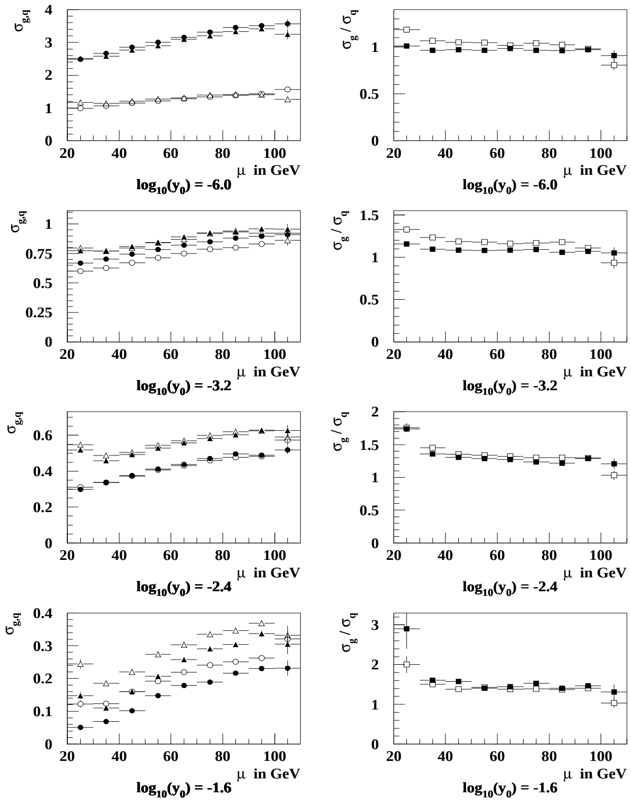
Abbildung D.4: Breite der Subjet-Multiplizitätsverteilung von Gluon- und Quarkjets als Funktion der Größe \mu = k_t^{min}/2 für einzelne Werte von y_0 . Die Meßgrößen auf Hadronebene (volle Symbole) und Partonebene (offene Symbole) sind für den Durham-Algorithmus mit veränderter Distanzgröße und Verwendung von Akzeptanzkegeln um die Jetachsen dargestellt. Gluonjets sind durch Dreiecke, Quarkjets durch Kreise und das Verhältnis \frac{Gluon}{Quark} ist durch Quadrate gekennzeichnet.
