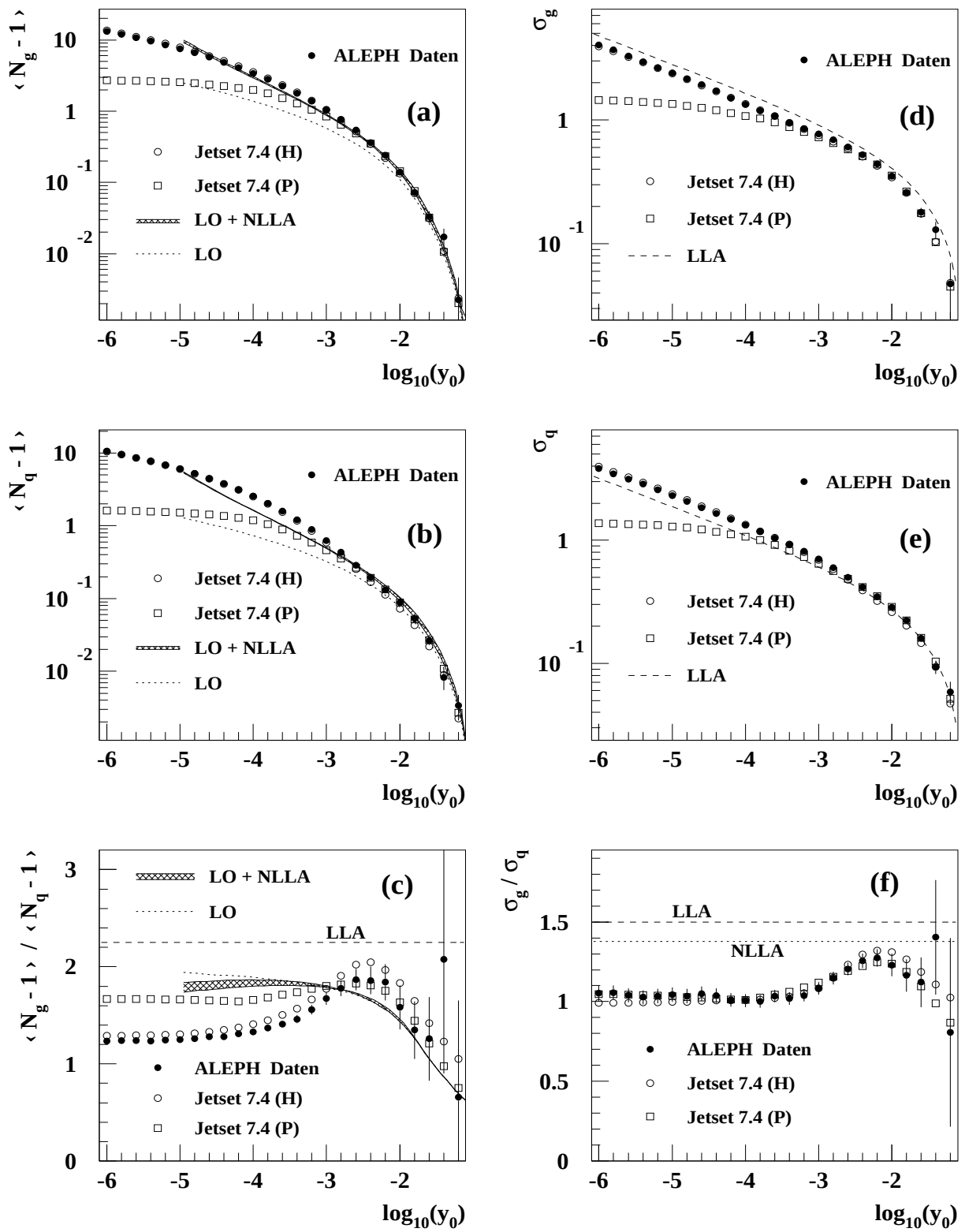
Abbildung 6.7: Mittelwert und Standardabweichung der Subjet-Multiplizitätsverteilung von Gluon- und Quarkjets als Funktion des Subjet-Auflöseparameters y_0 . Die Meßergebnisse für den E_{jet} -integrierten Fall werden mit perturbativen QCD-Vorhersagen (siehe Text) und dem Hadron- und Partonniveau des Modells Jetset 7.4 verglichen. Wenn die offenen Kreise (Hadronen in Jetset) in einigen Bildern nicht sichtbar sind, so liegen sie direkt unter den vollen Kreisen (ALEPH-Daten).
