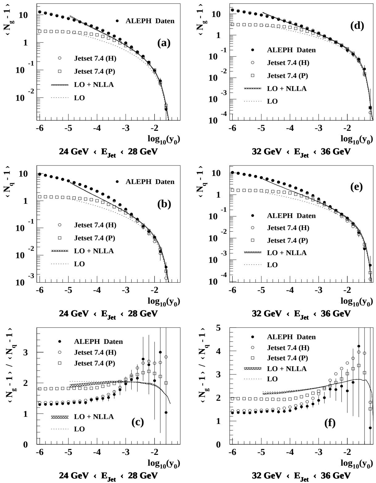
Abbildung 6.8: Die mittlere Subjet-Multiplizität von Gluon- und Quarkjets als Funktion des Subjet-Auflöseparameters y_0 . Die Meßergebnisse für die Jetenergieintervalle 24 \text{ GeV} \leq E_{\text{jet}} \leq 28 \text{ GeV} und 32 \text{ GeV} \leq E_{\text{jet}} \leq 36 \text{ GeV} werden mit perturbativen QCD-Vorhersagen (siehe Text) und dem Hadron- und Partonniveau des Modells Jetset 7.4 verglichen. Wenn die offenen Kreise (Hadronen in Jetset) in einigen Bildern nicht sichtbar sind, so liegen sie direkt unter den vollen Kreisen (ALEPH-Daten).
