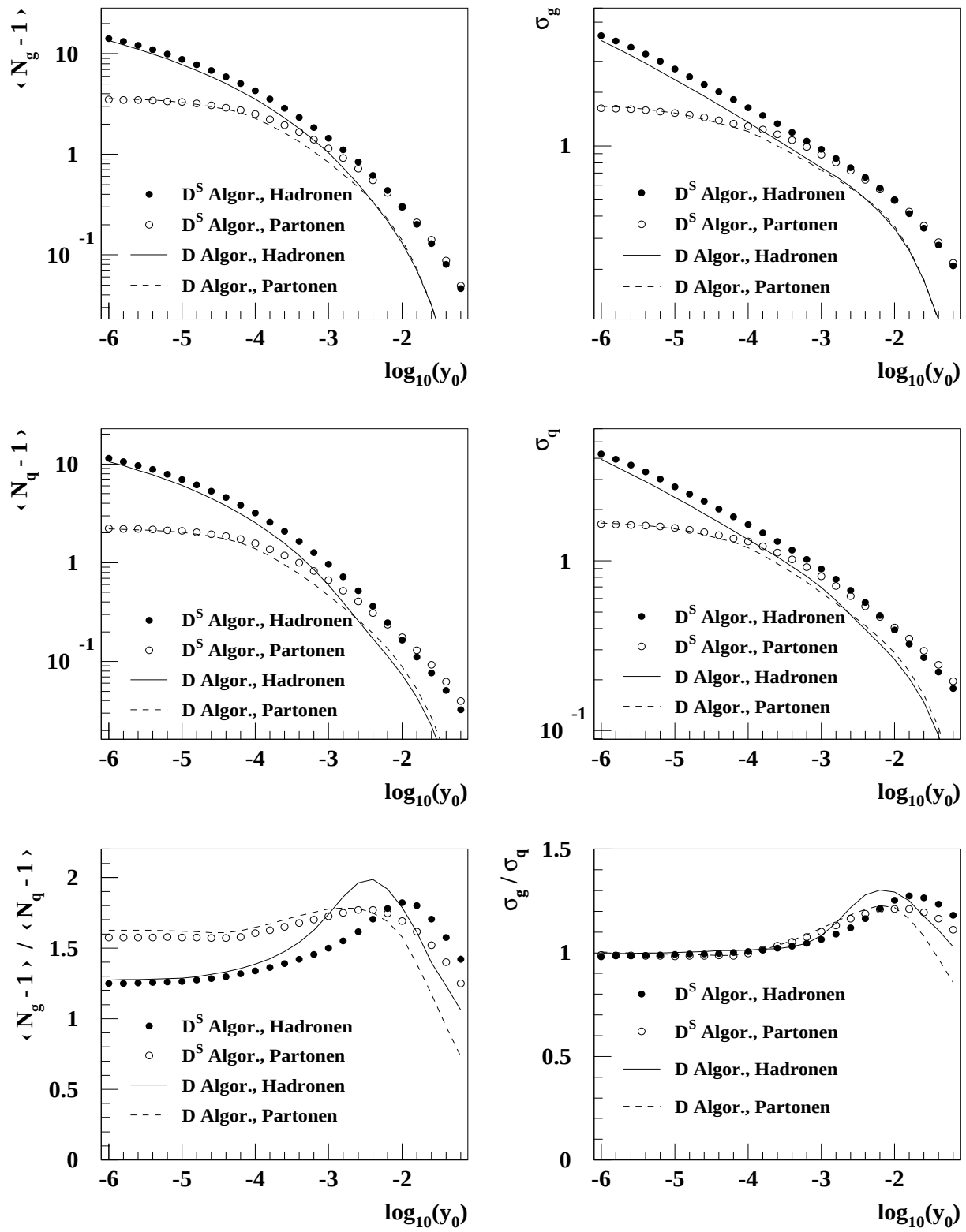
Abbildung B.1: Mittelwert und Breite der Subjet-Multiplizitätsverteilung von Gluon- und Quarkjets als Funktion des Subjet-Auflöseparameters y_0 . Die Meßgrößen auf Parton- und Hadronniveau für den Durham-Algorithmus mit veränderter Distanzgröße ( D^S ) sind mit denen für den Standard-Durham-Algorithmus ( D ) verglichen. Diese Bilder beinhalten alle zur Verfügung stehenden Jetenergien.
