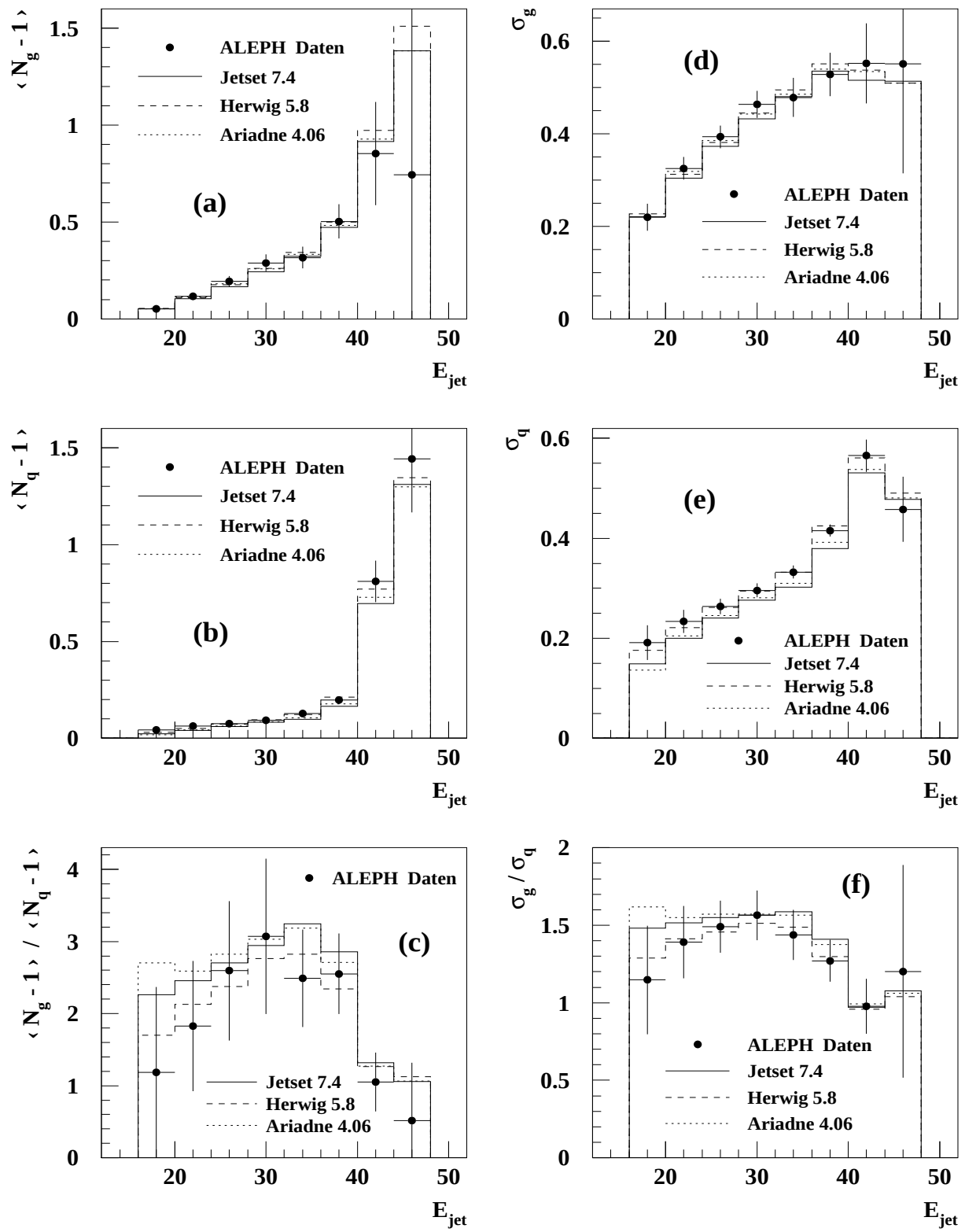
Abbildung 6.6: Mittelwert und Standardabweichung der Subjet-Multiplizitätsverteilung von Gluon- und Quarkjets als Funktion der Jetenergie E_{\text{jet}} . Die Meßergebnisse für y_0 = 10^{-2.2} ( \hat{=} k_t \approx 7.2 \text{ GeV} ) werden mit den Hadronniveau-Vorhersagen unterschiedlicher MC-Modelle verglichen.
