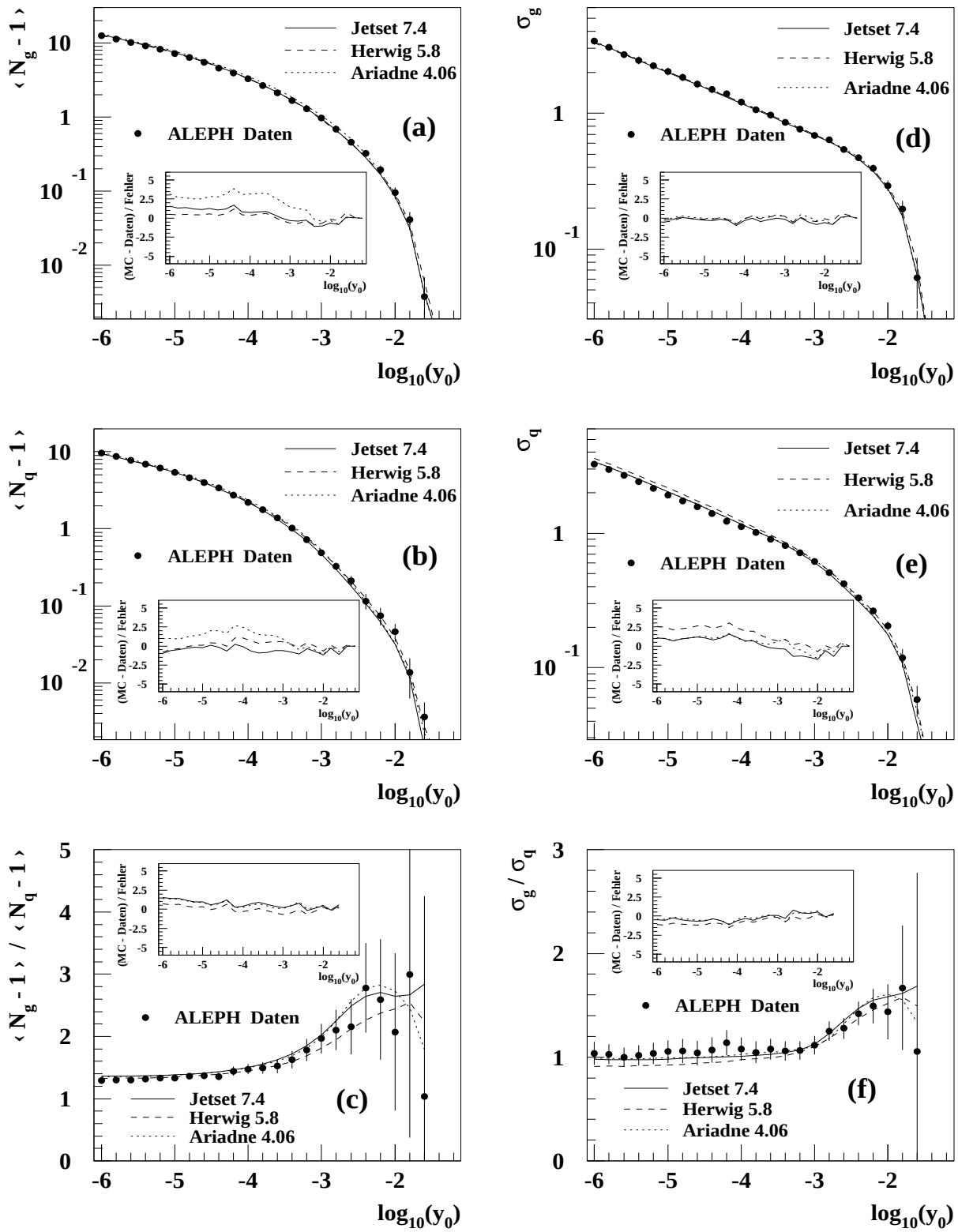
Abbildung 6.2: Mittelwert und Standardabweichung der Subjet-Multiplizitätsverteilung von Gluon- und Quarkjets als Funktion des Subjet-Auflöseparameters y_0 . Die Meßergebnisse für das Jetenergieintervall 24 \text{ GeV} \leq E_{jet} \leq 28 \text{ GeV} werden mit den Hadronniveaue Vorhersagen unterschiedlicher MC-Modelle verglichen. In den Unterbildern ist jeweils die Differenz zwischen Modellvorhersage und Daten normiert auf den Gesamtfehler dargestellt.
