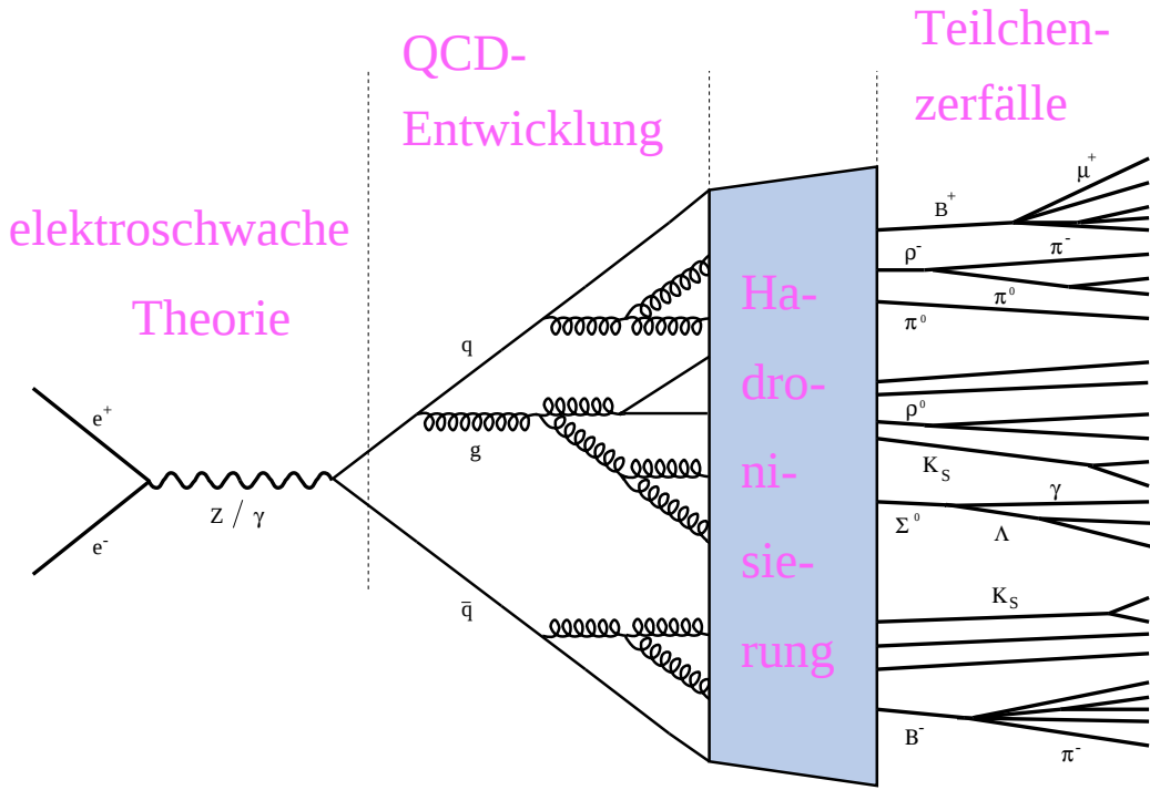
Abbildung 2.2: Schematische Darstellung eines hadronischen Ereignisses in e^+e^- -Annihilationen.
