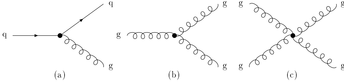
Abbildung 2.1: Die fundamentalen Vertices der QCD: (a) Quark-Gluon Vertex, (b) Triple-Gluon Vertex, (c) Vier-Gluon Vertex
