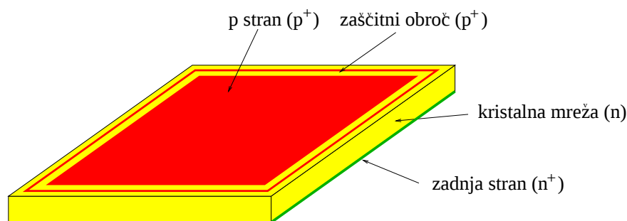
Slika 9.1: Shematični prikaz diod, uporabljenih v tem delu. Prikazana je tudi struktura p strani z zaščitnim obročem. Zaradi visoke koncentracije primesi je p stran označena kot p^+ .
