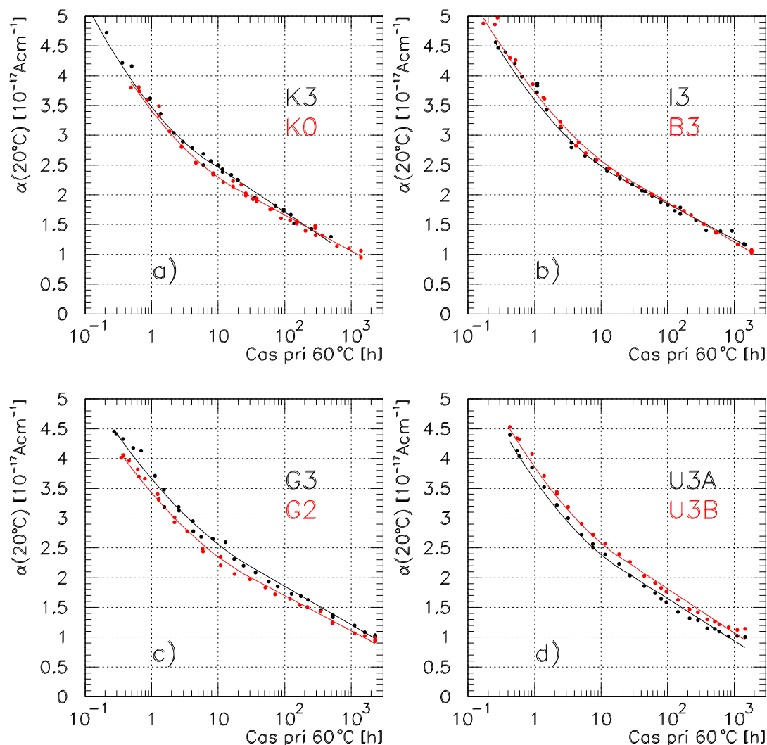
Slika 9.9: Časovni razvoj počasnih komponent zapornega toka. V tabeli so navedeni pogoji obsevanja in rezultati prilagajanja po enačbi 9.28. Vrednosti parametra \alpha so normalizirane na 20°C.
