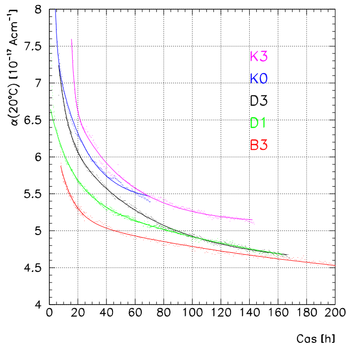
Slika 9.8: Hitro okrevanje zapornega toka. Vrednosti parametra \alpha so normalizirane na 20°C po enačbi j(T_2) = j(T_1) \left(\frac{T_2}{T_1}\right)^2 e^{-\frac{E'_g}{2k_B}(T_2^{-1} - T_1^{-1})} . Za E'_g je bila uporabljena vrednost 1.2 eV [14]. Opozoriti velja, da se na sliki ordinatna os ne začne pri ničli.
