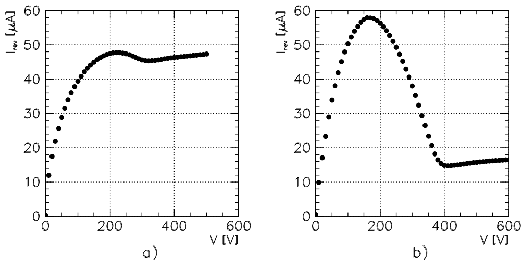
Slika 9.4: Primer I/V meritve diode a) v začetni fazi (po 5 dneh pri 5°C) in b) v pozni fazi (po 5 dneh 60°C) okrevanja zapornega toka. Generacijski tok je določen kot vrednost zapornega toka v minimumu za hrbtom.
