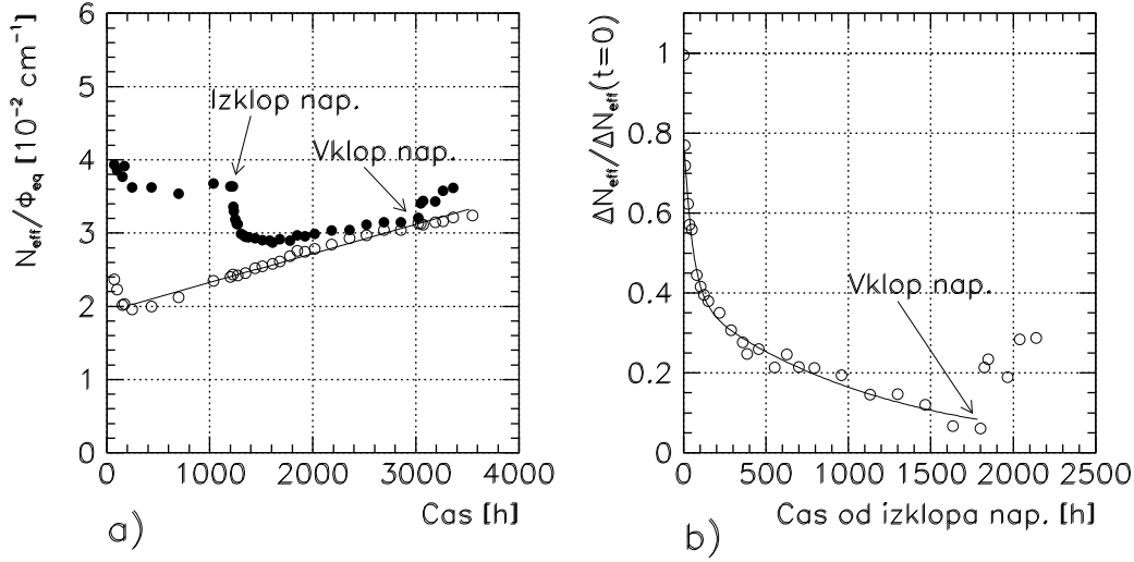
Slika 9.14: a) Časovni razvoj N_{eff} za diodo z (polni krogci) in brez (prazni krogci) napajalne napetosti. Razen napajalne napetosti sta bili diodi obsevane in hranjeni pod enakimi pogoji pri temperaturi 20°C. b) Časovni razvoj razlike v N_{eff} po izklopu napajalne napetosti. Razlika je normalizirana na vrednost tik pred izklopom. Upadanje razlike lahko lepo popišemo z dvema eksponentnima funkcijama (polna črta). Po ponovnem vklopu napajalne napetosti (približno 1800 ur po izklopu) opazimo ponovno naraščanje N_{eff} .
