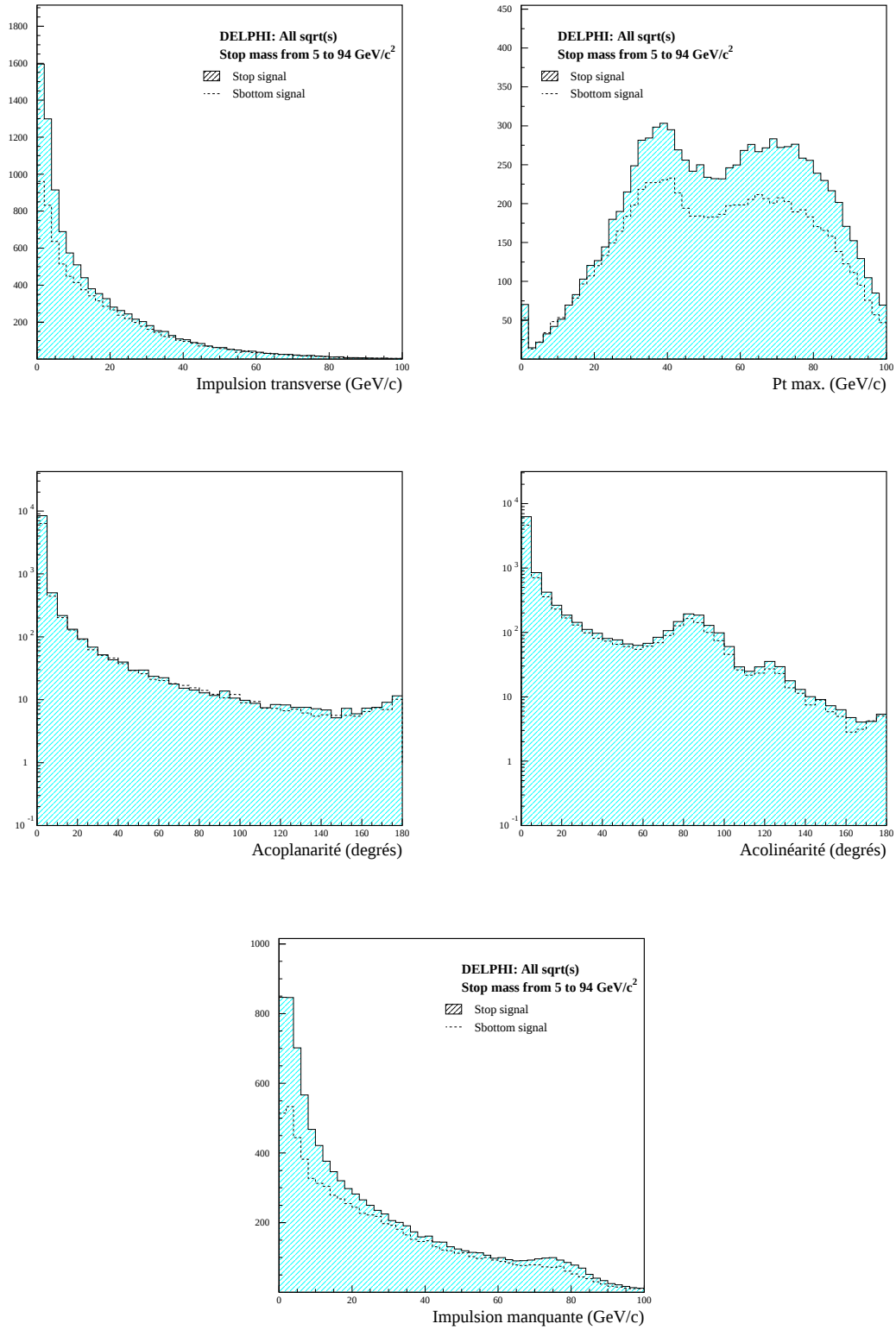
FIG. 5.6 – Quelques distributions caractéristiques des événements s -hadrons générés avec SUSYGEN. Les signaux stop et sbottom montrés correspondent à une masse entre 5 et 94 \text{GeV}/c^2 .
