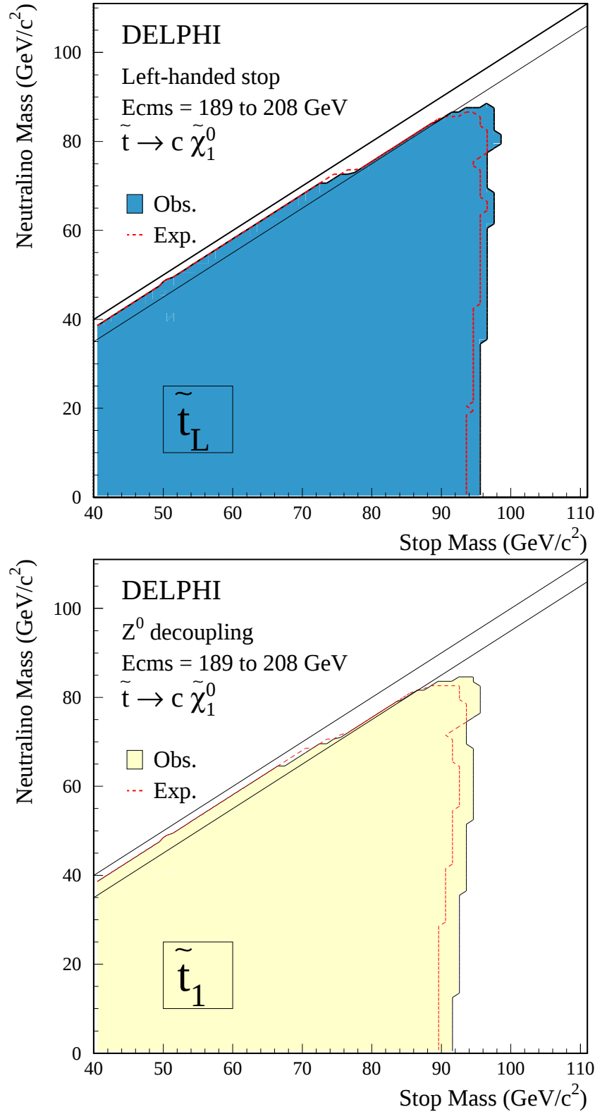
FIG. C.1 – Régions exclues à 95% CL dans le plan (M_{\tilde{t}_1}, M_{\tilde{\chi}_1^0}) par les analyses effectuées dans DELPHI pour rechercher le stop dans le canal c\tilde{\chi}_1^0 pour l'état purement gauche (diagramme du haut) et pour l'état au découplage du Z^0 (diagramme du bas). Les résultats de l'analyse du cas dégénéré (sujet du chapitre 7 de cette thèse) sont combinés avec ceux de l'analyse du cas non dégénéré [44].
