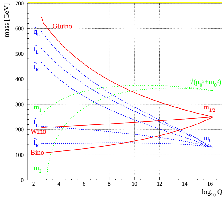
FIG. 1.8 – Evolution des paramètres de masse dans mSUGRA [21].
