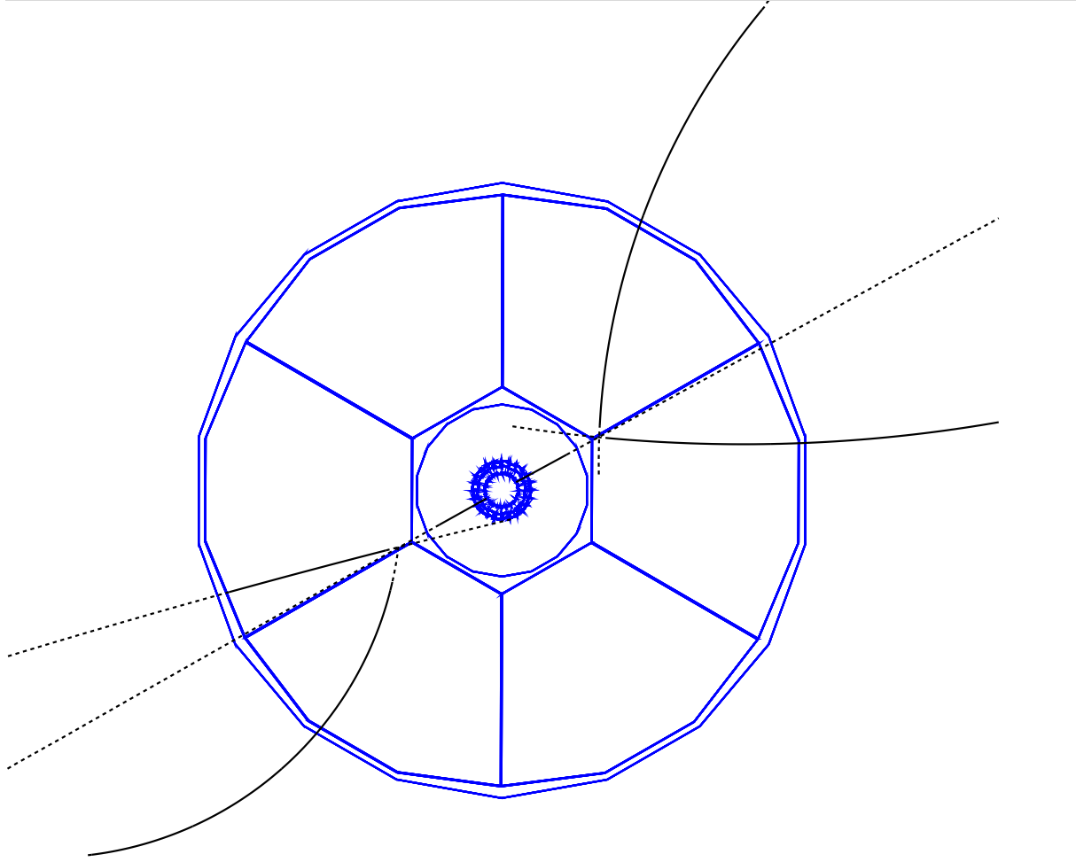
FIG. 5.11 – Simulation de la trace primaire d'un événement stop se désintégrant en \pi^+\pi^- dans la TPC. Les pointillés indiquent l'extrapolation des traces de l'événement.
