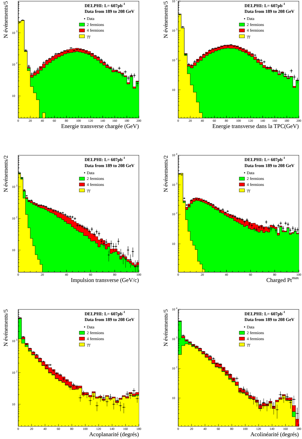
FIG. 9.2 – Comparaison entre données et simulation des processus standards au niveau de la présélection.
