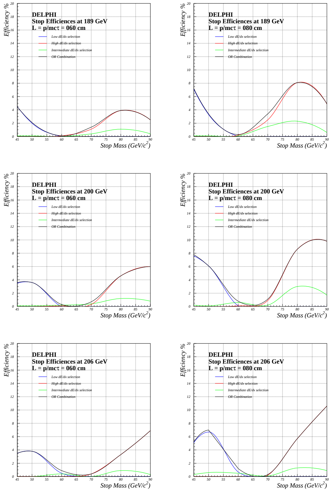
FIG. 9.7 – Courbes d'efficacité de détection de stop de durées de vie intermédiaires obtenues par l'application de l'analyse de recherche de s -hadrons pour \sqrt{s} = 189, 200 et 206 GeV et un parcours moyen \hat{L} = 60 et 80 cm.
