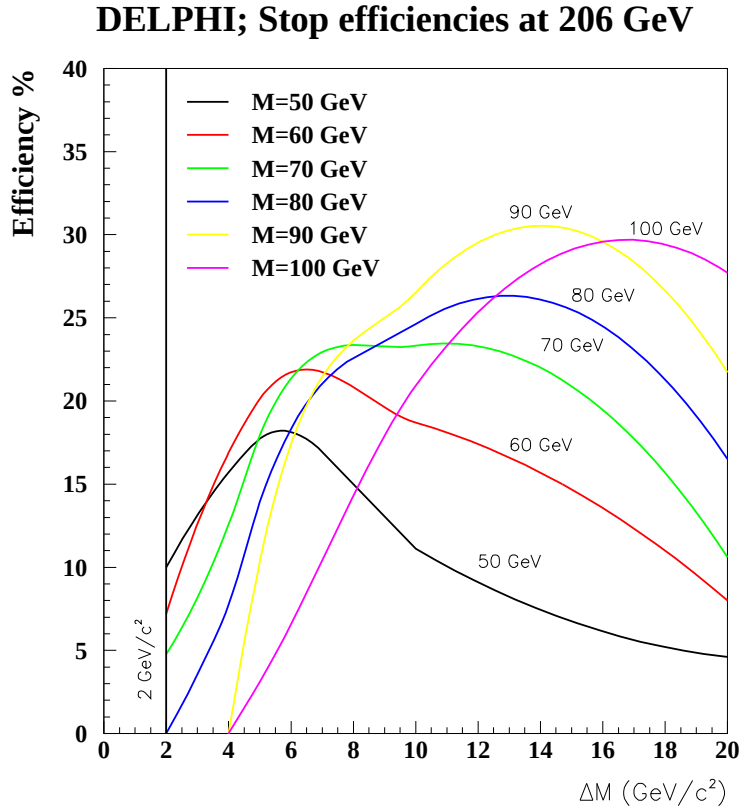
FIG. 7.7 – Efficacité de détection du signal pour différentes hypothèses de masses de stop en fonction de \Delta M = M_{\tilde{t}_1} - M_{\tilde{\chi}_1^0} , à \sqrt{s}=189 et 206 GeV.
