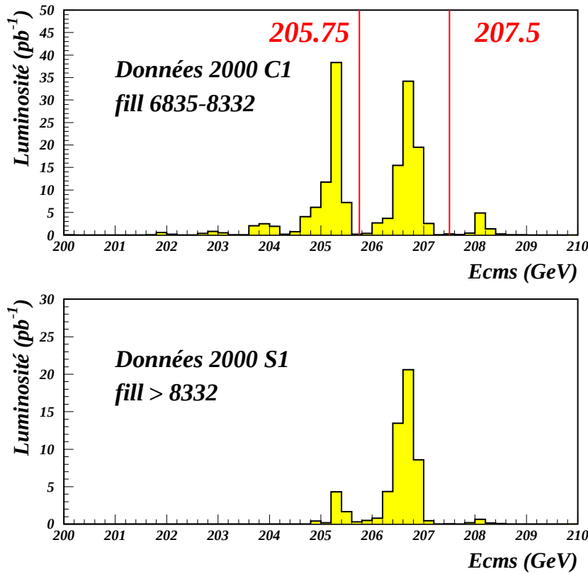
FIG. 5.1 – Luminosité intégrée en \text{pb}^{-1} en fonction de l'énergie dans le centre de masse pour les données de l'an 2000. Les histogrammes du haut et du bas montrent les distributions des données collectées avec (C1) et sans (S1) le secteur 6 de la TPC.
