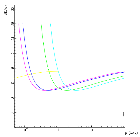
FIG. 8.10 – Candidat présentant un dE/dx anormalement bas.
