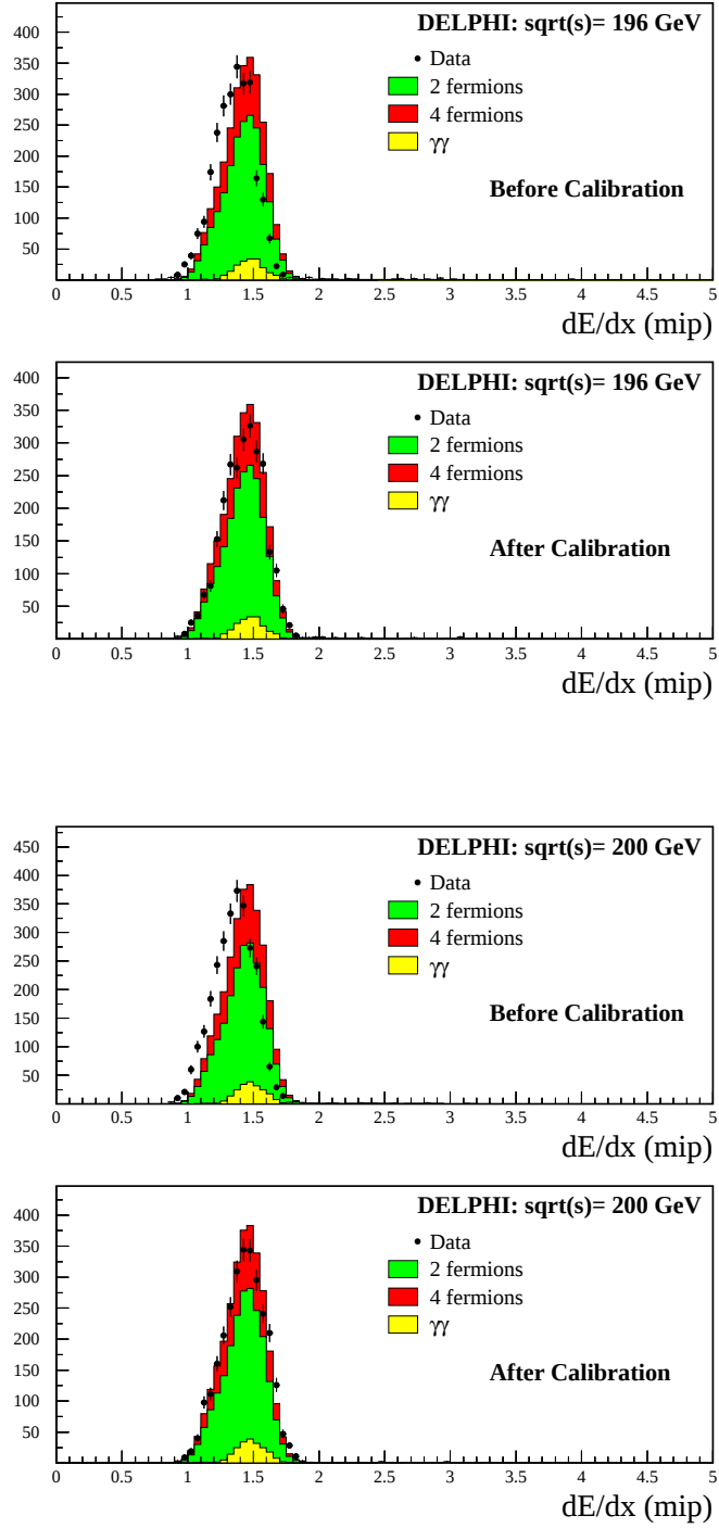
FIG. 4.4 – Calibration du dE/dx (à 196 GeV et 200 GeV)
