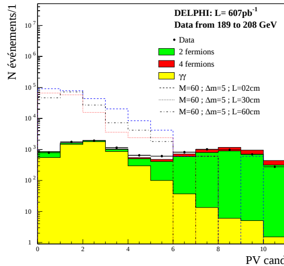
FIG. 9.3 – Comparaison entre données et simulation des processus standards pour le nombre de traces primaires PV . Des signaux de stop de 60 GeV/c 2 de masse et de \Delta m = 5 GeV/c 2 sont également montrés pour un parcours moyen \hat{L} = 2, 30 et 60 cm.
