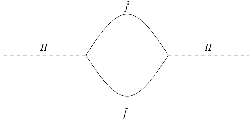
FIG. 1.6 – Contribution sfermionique à la correction radiative à une boucle sur la masse du boson de Higgs.
