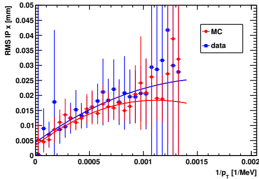
(e) 5 PVs
