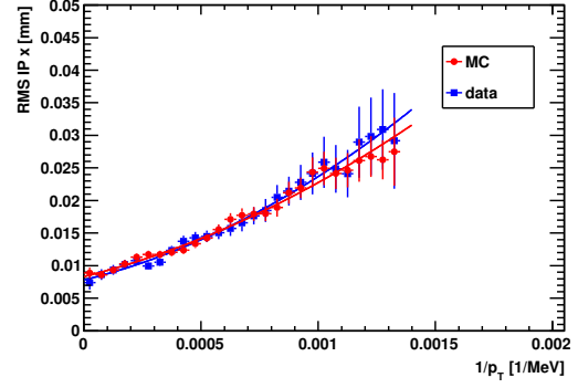
(b) 2 PVs
