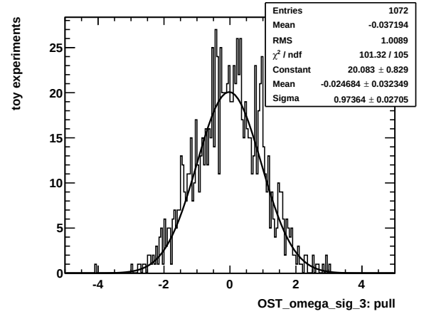
(d) Category 3
