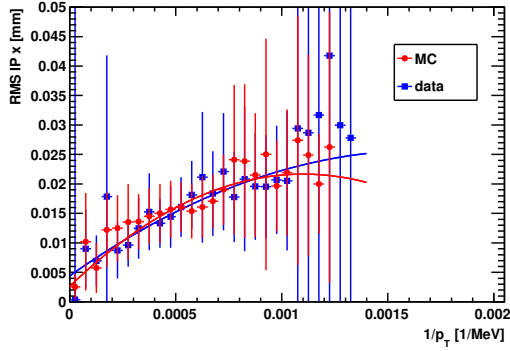
(e) 5 PVs
