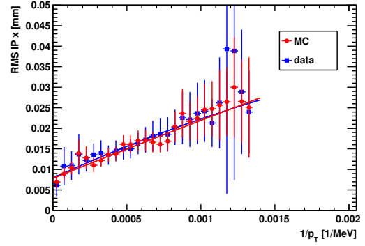
(d) 4 PVs
