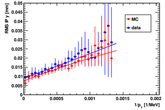
(d) 4 PVs
