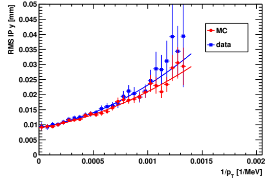
(b) 2 PVs
