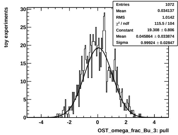
(d) Category 3
