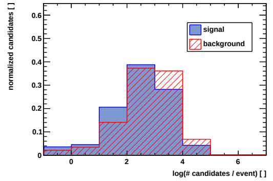
(d) \log(\#candidates/event)
