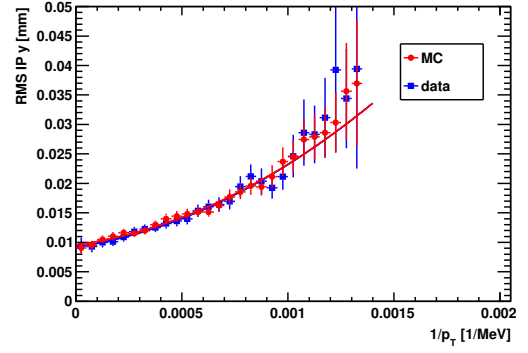
(b) 2 PVs
