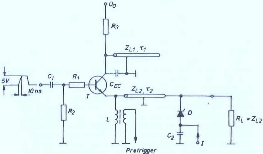
Abb. 5.1 Vereinfachte Schaltung des verwendeten Impuls- generators
