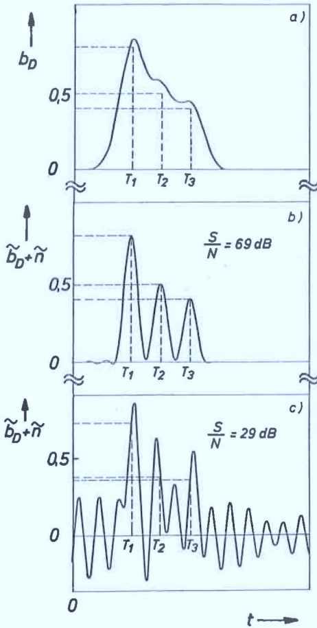
Abb. 4.3 Zahlenbeispiel für die Anwendung eines inversen Filters zur Verbesserung der Auflösung (Bandbreite \Delta f = 2,3 \text{ GHz} ) a.) Ungefilterte Echofunktion b.) Gefilterte Echofunktion für S/N = 69 \text{ dB} , Blackman - Fenster c.) Gefilterte Echofunktion für S/N = 29 \text{ dB} , andere Daten wie unter b.)
