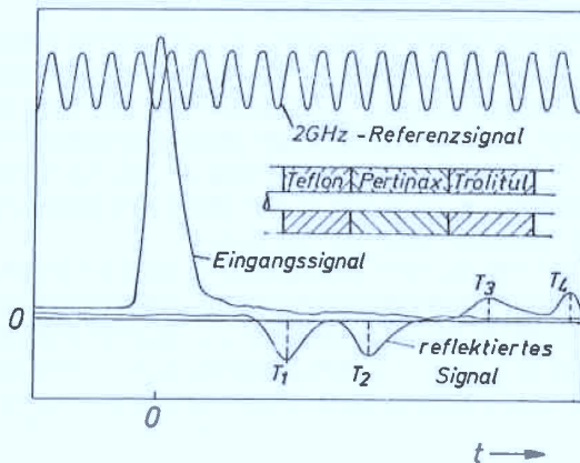
Abb. 5.15 TDR-Messung dielektrischer Einsätze in der Koaxialleitung
