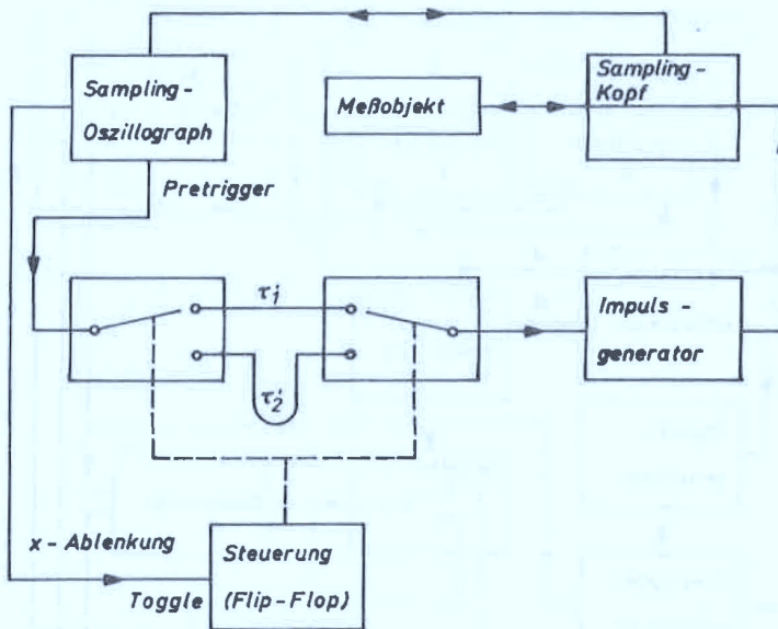
Abb. 5.11 Blockschaltbild zur Pretriggerumtastung
