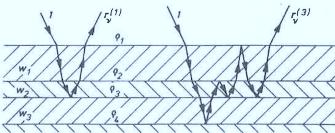
Abb. 2.2 Beispiele für Einzelübertragungswege
