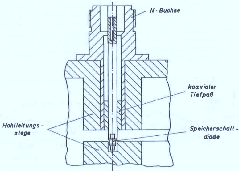
Abb. 5.8 Steghohlleitung mit integrierter Speicherschaltodiode
