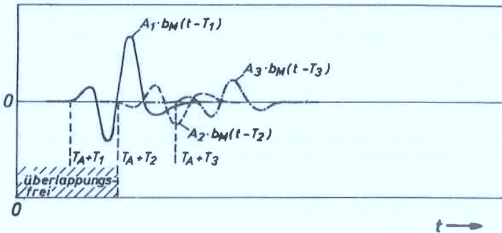
Abb. 4.4 Erläuterung des überlappungsfreien Gebietes
