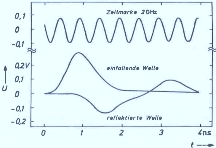
Abb. 5.13 Gleichzeitige Darstellung von Zeitmarke, Meß- und Referenzsignal [59] unter Verwendung des Meßaufbaus nach Abb. 5.12
