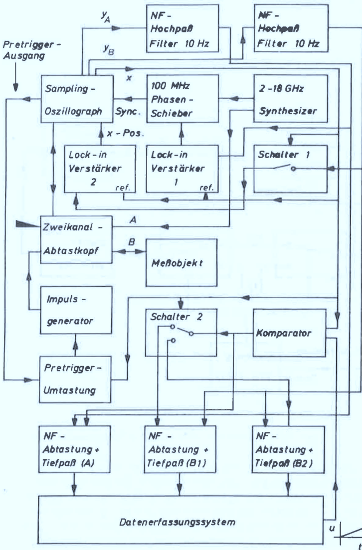
Abb. 5.12 Blockschaltbild des stabilisierten Zeitbereichsmeßplatzes
