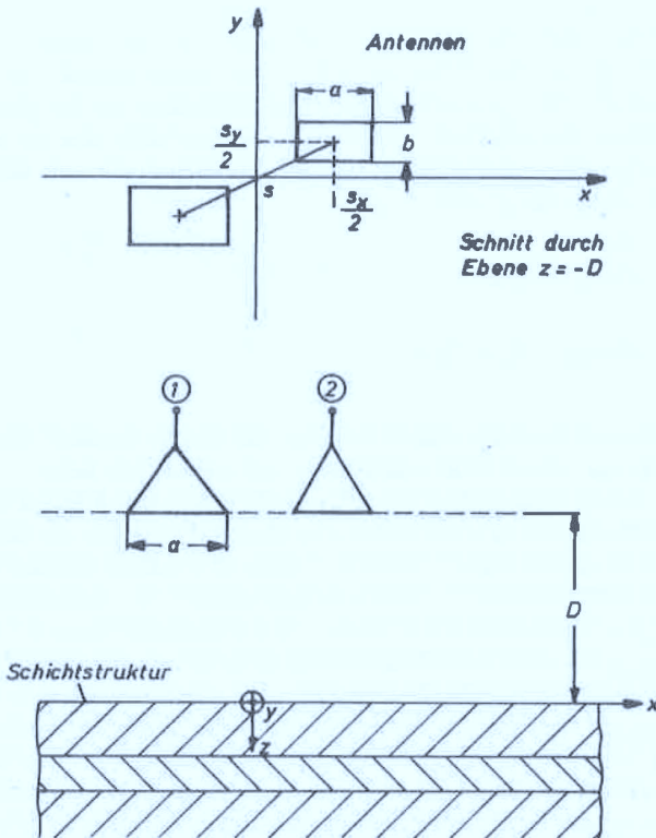
Abb. 3.2 Antennen - Schichtstruktur - Konfiguration
