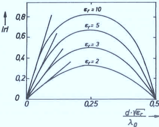
Abb. 2.4 Reflexionsfaktor r(\frac{d}{\lambda_0}\sqrt{\epsilon_r}) dünner, dielektrischer Schichten
