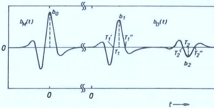
Abb. 4.2 Einfaches Auswerteverfahren für Echos ohne zeitliche Überlappung
