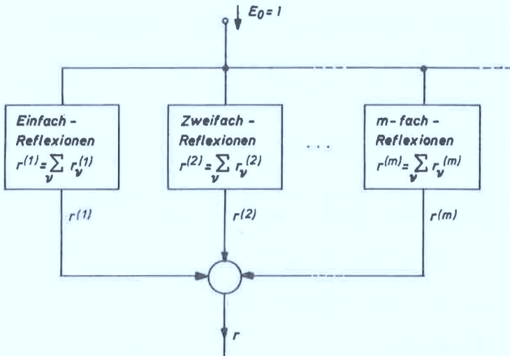
Abb. 2.3 Darstellung von r durch eine Bremmer-Reihe
