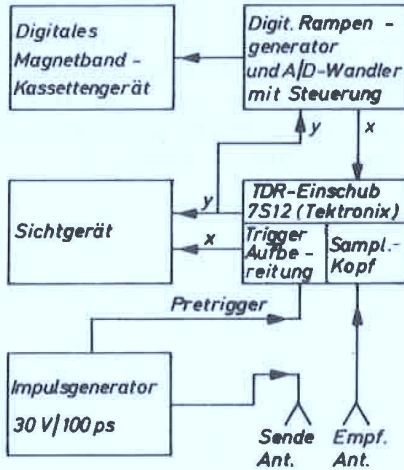
Abb. 5.14 Blockschaltbild des Kurzimpulsradargerätes
