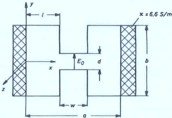
Abb. 5.5 Steghohlleitung mit Dämpfungseinsatz
