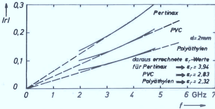
Abb. 6.1 Ermittlung der Dielektrizitätszahl dünner ( d \ll \lambda_0 / \sqrt{\epsilon_r} ) dielektrischer Schichten aus der Frequenzabhängigkeit des Reflexionsfaktors [67]
