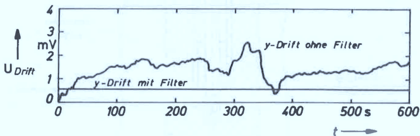
Abb. 5.9 Vertikaldrift des Samplingsystems mit und ohne NF-Hochpaßfilter ( f_{scan} = 100 Hz, f_g = 10 Hz)
