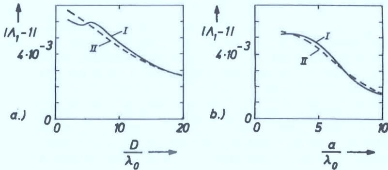
Abb. 3.4 Abweichung der normierten Reflexion an der ersten Grenzschicht gegenüber der Reflexion einer senkrecht einfallenden ebenen homogenen Welle (zweidimensionaler TE-Fall; f = 8 GHz; \epsilon_{r,1} = 2 ; s = 0 ) a.) a/\lambda_0 = 5 b.) D/\lambda_0 = 10,67 I: Numerische Auswertung von Gl. (3.36a), exakte Lösung II: Näherung nach Gl. (3.39), d_{\text{eff}} = 0
