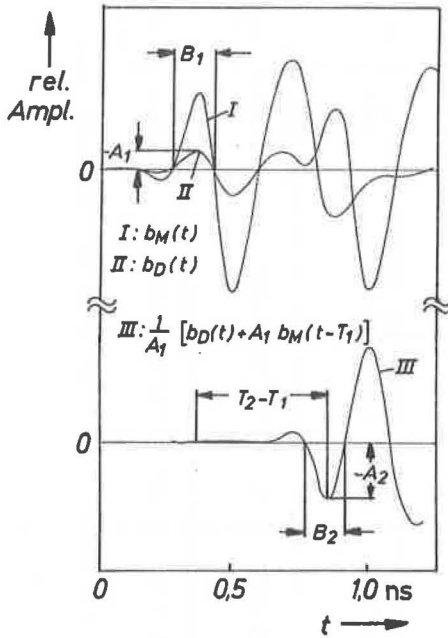
Abb. 5.17 Beispiel für die Empfangssignale von Schichtstrukturen
