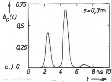
Abb. 3.7 Berechnete Einhüllende der Echofunktion für eine dielektrische Platte ( d_1 = 0,2 m; \epsilon_{r,1} = 2 ; \epsilon_{r,2} = 1 ) für verschiedene Werte des Antennenversatzes s ; zweidimensionaler Fall; Antenne ( a = 0,2 m) im Abstand D = 0,5 m; Gauimpuls mit f_0 = 6 GHz und einer 20 dB-Bandbreite von \Delta f = 3 GHz
