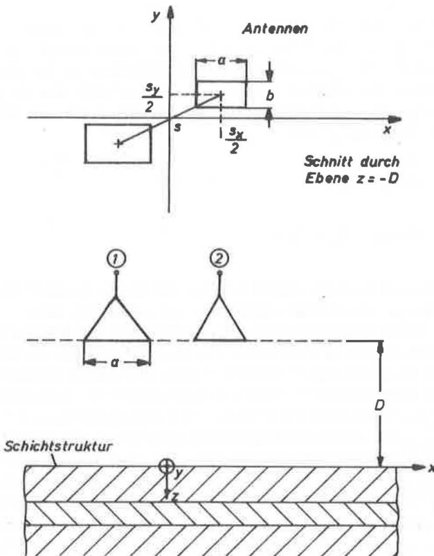
Abb. 3.2 Antennen - Schichtstruktur - Konfiguration
