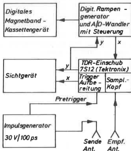
Abb. 5.14 Blockschaltbild des Kurzimpulsradargerätes
