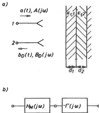
Abb. 4.1 Antennen - Schichtstruktur - Konfiguration (a) und zugehöriges Zweitorersatzschaltbild (b)
