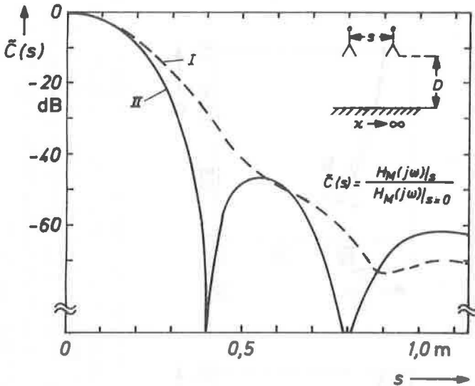
Abb. 3.6 Abhängigkeit der Übertragungsfunktion H_M(j\omega) zwischen zwei Antennen vom Versatz s ; Reflexion an einer Metallplatte im Abstand D = 0,5 m; (zweidimensionaler Fall, f = 6 GHz; a = 0,2 m) I. Numerische Auswertung von Gl. (3.40) II. Näherung über stationäre Phase
