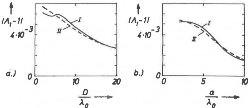
Abb. 3.4 Abweichung der normierten Reflexion an der ersten Grenzschicht gegenüber der Reflexion einer senkrecht einfallenden ebenen homogenen Welle (zweidimensionaler TE-Fall; f = 8 \text{ GHz} ; \epsilon_{r,1} = 2 ; s = 0 ) a.) a/\lambda_0 = 5 b.) D/\lambda_0 = 10,67 I: Numerische Auswertung von Gl. (3.36a), exakte Lösung II: Näherung nach Gl. (3.39), d_{\text{eff}} = 0
