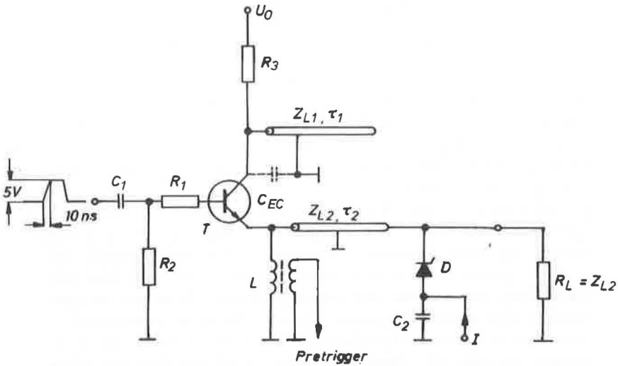
Abb. 5.1 Vereinfachte Schaltung des verwendeten Impuls- generators
