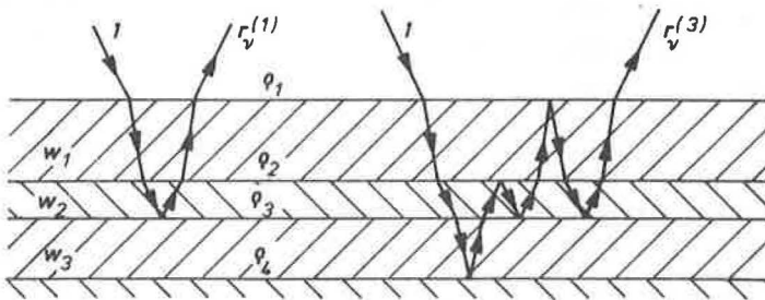
Abb. 2.2 Beispiele für Einzelübertragungswege
