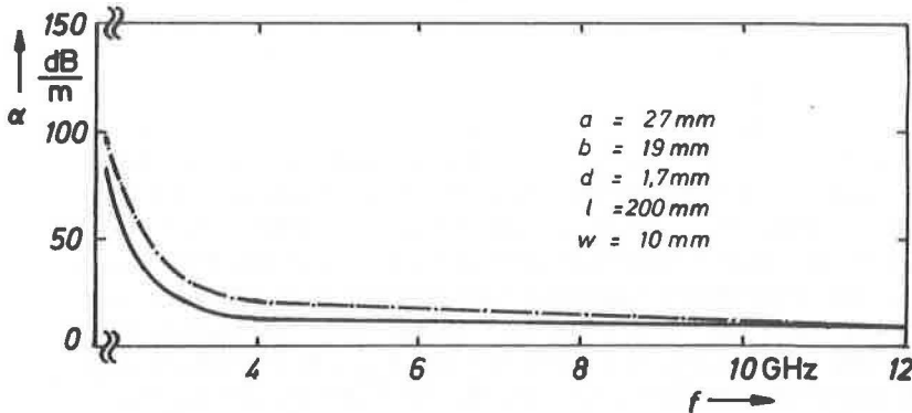
Abb. 5.6 Gemessener (---) und errechneter (—) Verlauf der Dämpfung einer Steghohlleitung nach Abb. 5.5 mit verlustbehafteten Seitenwänden
