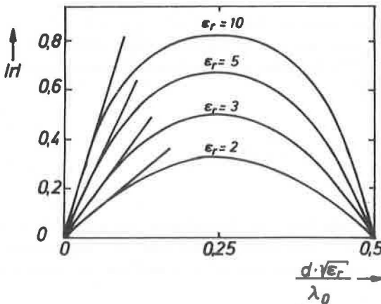
Abb. 2.4 Reflexionsfaktor r(\frac{d}{\lambda_0}\sqrt{\epsilon_r}) dünner, dielektrischer Schichten
