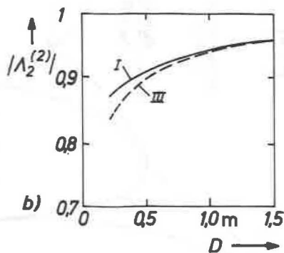
Abb. 3.5 Abweichung der normierten Reflexion an der zweiten Grenzschicht gegenüber der Reflexion einer senkrecht einfallenden ebenen homogenen Welle (zweidimensionaler TE-Fall; f = 6 GHz; a = 0,2 m; d_1 = 0,2 m; s = 0 ; \epsilon_{r,1} = 2 ; \epsilon_{r,2} = 1 ) a: Einfachreflexion, b: Zweifachreflexion, c: Dreifachreflexion I: Numerische Auswertung von Gl. (3.36a), II: Näherung nach Gl. (3.39) III: Näherung nach Gl. (3.38)
