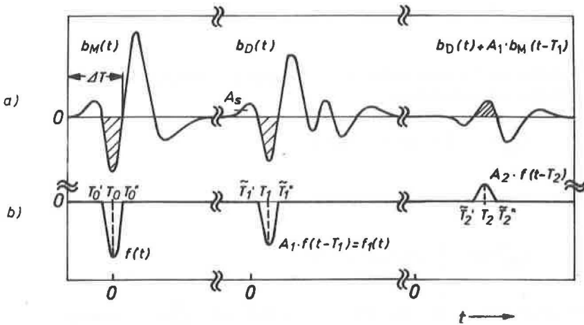
Abb. 4.5 Veranschaulichung des sukzessiven Subtraktionsverfahrens
