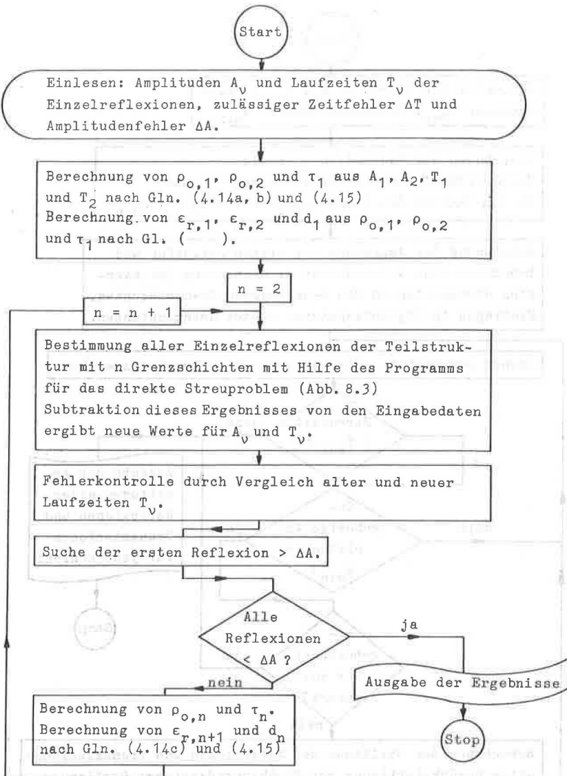
Abb. 8.4 Flußdiagramm zur Bestimmung der Dicken und Dielektrizitätszahlen aus den Amplituden und Laufzeiten der Einzelreflexionen (inverses Streuproblem)
