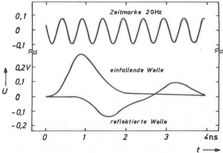
Abb. 5.13 Gleichzeitige Darstellung von Zeitmarke, Meß- und Referenzsignal [59] unter Verwendung des Meßaufbaus nach Abb. 5.12
