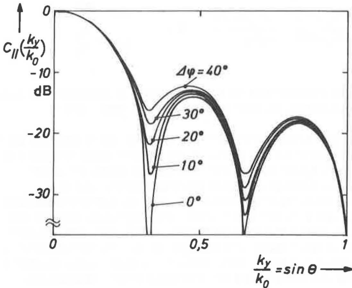
Abb. 8.1 Einfluß der Phasenbelegung auf das Richtdiagramm einer Hornantenne mit den Aperturabmessungen a = 0,2 m und b = 0,14 m (E-Ebene mit \phi = 90^\circ ; f = 6 GHz)
