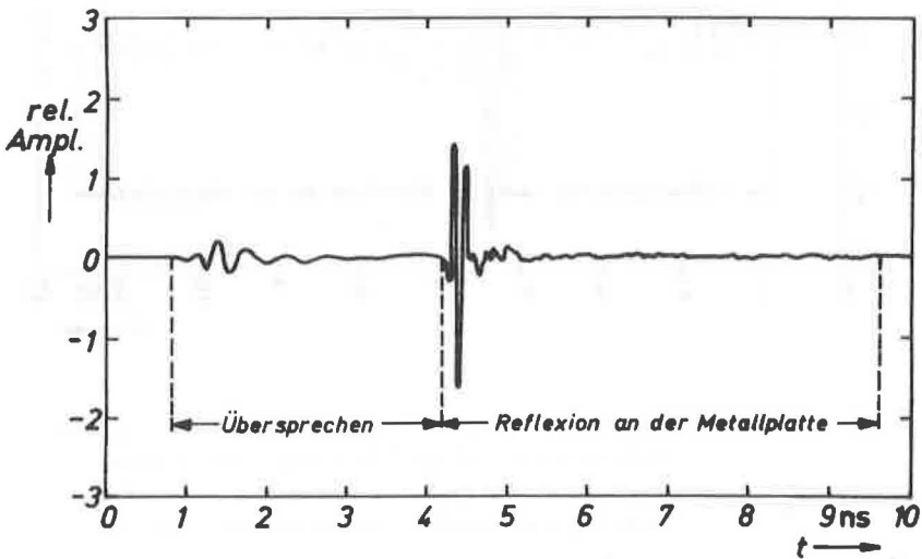
Abb. 5.4 Empfangener Impuls in einer Anordnung bestehend aus zwei Steghohlleitungshornantennen vor einer Metallplatte (Halbraum) unter Verwendung eines Hochpaßfilters
