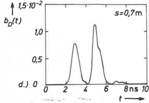
Abb. 3.7 Berechnete Einhüllende der Echofunktion für eine dielektrische Platte ( d_1 = 0,2 m; \epsilon_{r,1} = 2 ; \epsilon_{r,2} = 1 ) für verschiedene Werte des Antennenversatzes s ; zweidimensionaler Fall; Antenne ( a = 0,2 m) im Abstand D = 0,5 m; Gauimpuls mit f_0 = 6 GHz und einer 20 dB-Bandbreite von \Delta f = 3 GHz
