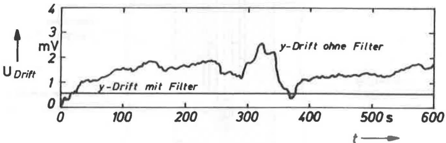
Abb. 5.9 Vertikaldrift des Samplingsystems mit und ohne NF-Hochpaßfilter ( f_{\text{scan}} = 100 Hz, f_g = 10 Hz)
