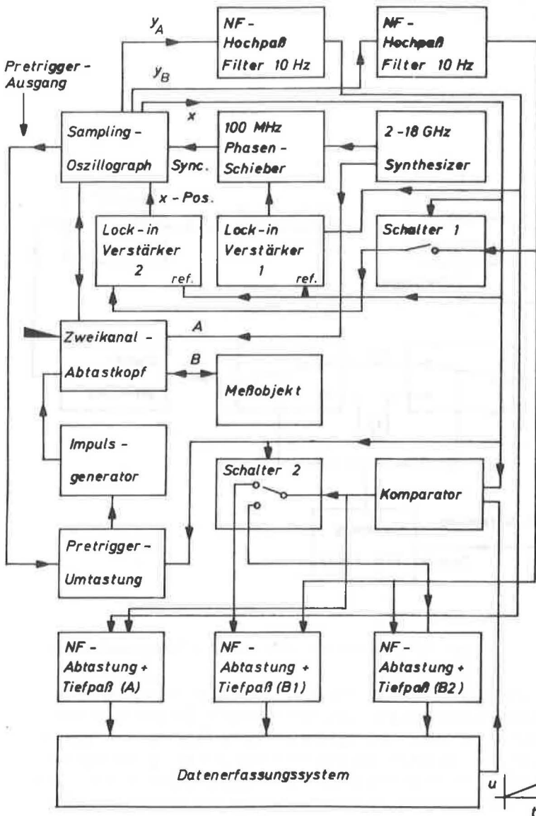
Abb. 5.12 Blockschaltbild des stabilisierten Zeitbereichsmeßplatzes
