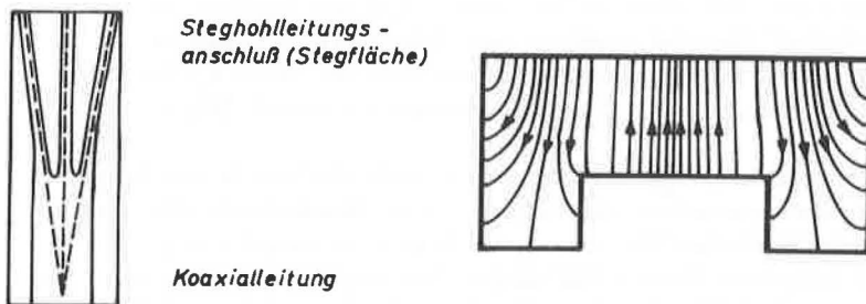
Abb. 5.7 Steifenleitungsstruktur als Koaxial-Steghohlleitungsübergang mit verringerter H_{30} - Anregung und Feldlinienbild ( E_{\text{transversal}} ) der H_{30} - Welle in der Steghohlleitung (halber Querschnitt)
