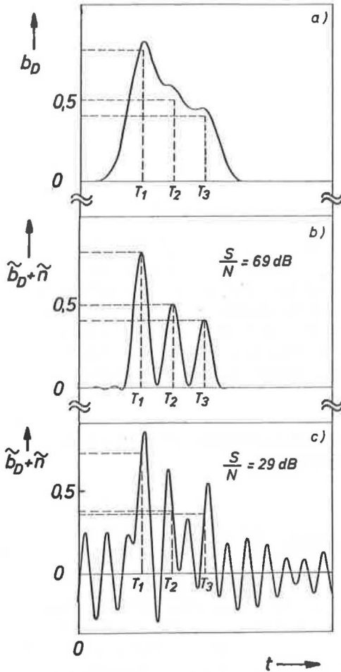
Abb. 4.3 Zahlenbeispiel für die Anwendung eines inversen Filters zur Verbesserung der Auflösung (Bandbreite \Delta f = 2,3 \text{ GHz} )
