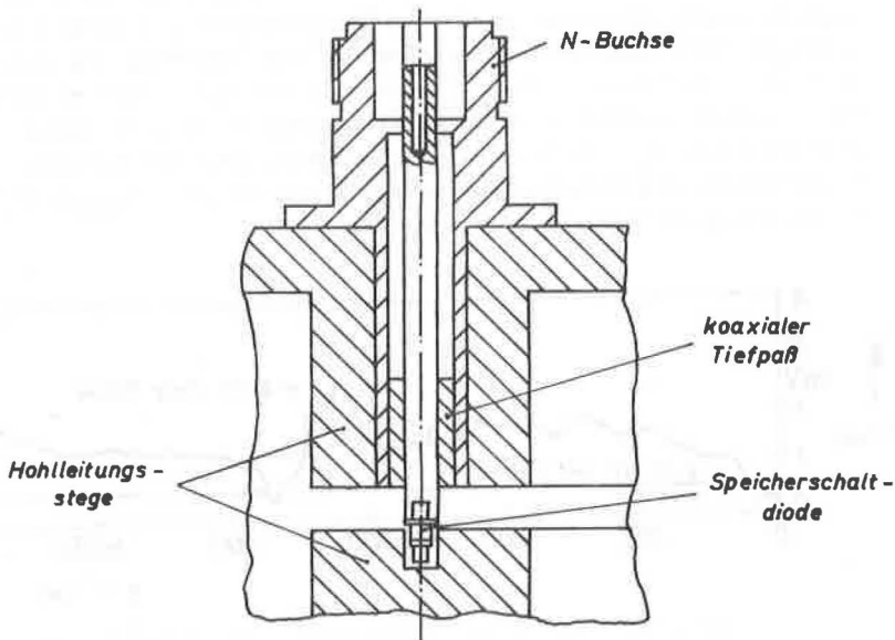
Abb. 5.8 Steghohlleitung mit integrierter Speicherschaltodiode
