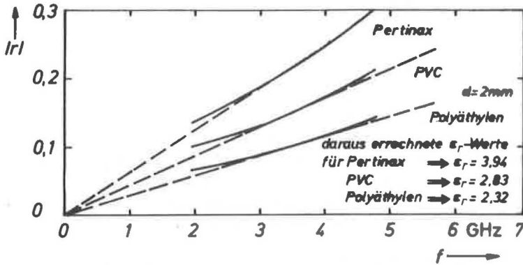
Abb. 6.1 Ermittlung der Dielektrizitätszahl dünner ( d \ll \lambda_0 / \sqrt{\epsilon_r} ) dielektrischer Schichten aus der Frequenzabhängigkeit des Reflexionsfaktors [67]
