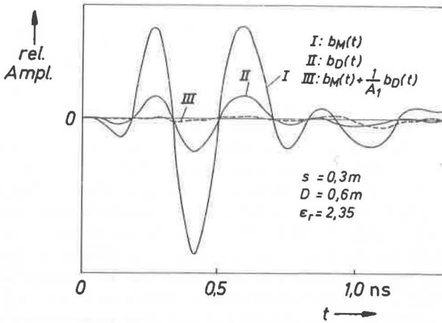
Abb. 5.16 Vergleich der Empfangssignale b_M(t) und b_D(t) für einen metallischen und dielektrischen "Halbraum"
