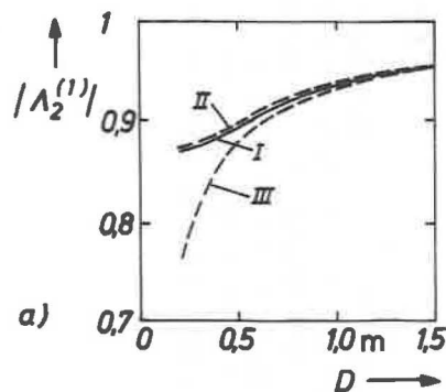
Abb. 3.5 Abweichung der normierten Reflexion an der zweiten Grenzschicht gegenüber der Reflexion einer senkrecht einfallenden ebenen homogenen Welle (zweidimensionaler TE-Fall; f = 6 GHz; a = 0,2 m; d_1 = 0,2 m; s = 0 ; \epsilon_{r,1} = 2 ; \epsilon_{r,2} = 1 ) a: Einfachreflexion, b: Zweifachreflexion, c: Dreifachreflexion I: Numerische Auswertung von Gl. (3.36a), II: Näherung nach Gl. (3.39) III: Näherung nach Gl. (3.38)
