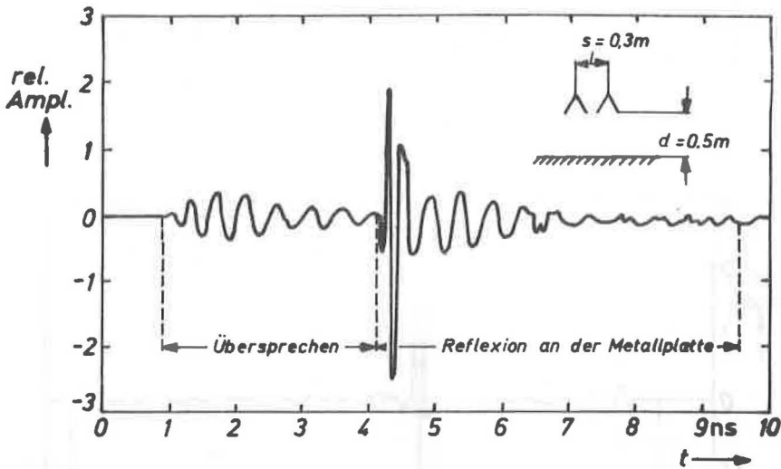
Abb. 5.3 Empfangener Impuls in einer Anordnung bestehend aus zwei Steghohlleitungshornantennen vor einer Metallplatte (Halbraum) ohne Verwendung von zusätzlichen Hochpaßfiltern
