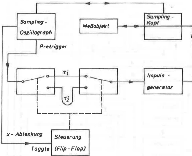
Abb. 5.11 Blockschaltbild zur Pretriggerumtastung
