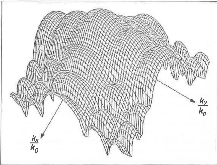
Abb. 8.2 Verlauf des Betrages der zweidimensionalen Fouriertransformierten der Aperturbelegung einer Hornantenne mit den Abmessungen a = 0,2 m und b = 0,14 m bei f = 6 GHz und einer Phasenbelegung mit \Delta\varphi = 100^\circ
