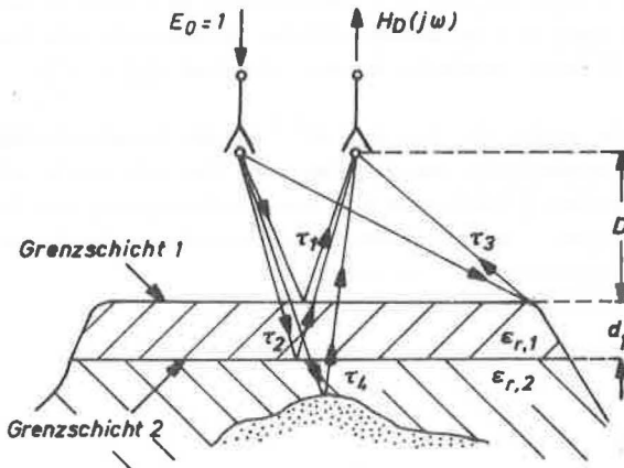
Abb. 3.1 Modell einer Schichtstruktur mit in der Breite und Tiefe begrenzter Ausdehnung; \tau_1 \dots \tau_4 sind die Laufzeiten zu den Grenzschichten bzw. Inhomogenitäten. H_D(j\omega) = Übertragungsfunktion
