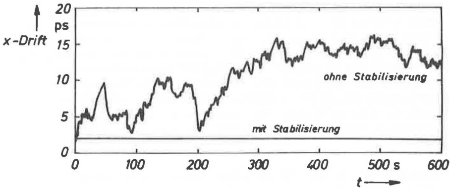
Abb. 5.10 Horizontal drift des Samplingsystems ohne und mit Stabilisierung
