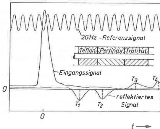
Abb. 5.15 TDR-Messung dielektrischer Einsätze in der Koaxialleitung
