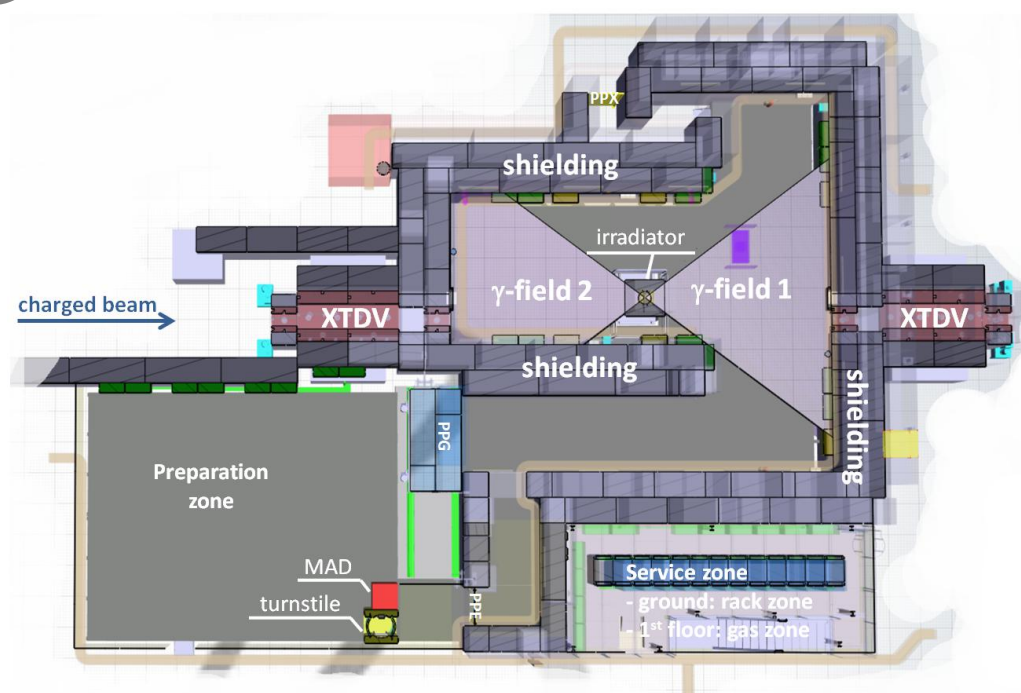
(a) Schéma de l'intérieur du Bunker du GIF++.
