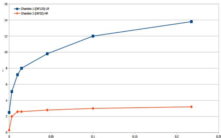
Fig. 5.56 Courant ( \mu\text{A} ) parcourant la chambre de basse résistivité la plus proche de la source (bleu) et "float glass" (orange) en fonction de l'inverse du facteur d'atténuation. La tension appliquée est fixée à 6900V.
