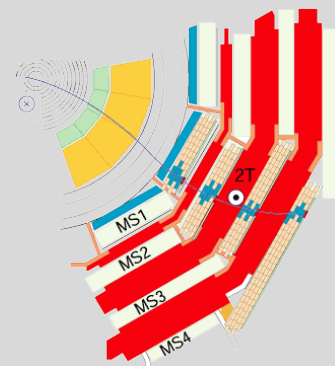
Fig. 3.25 Coupe dans le plan transverse d'un quart du détecteur CMS montrant la trajectoire d'un muon (courbe bleue).
