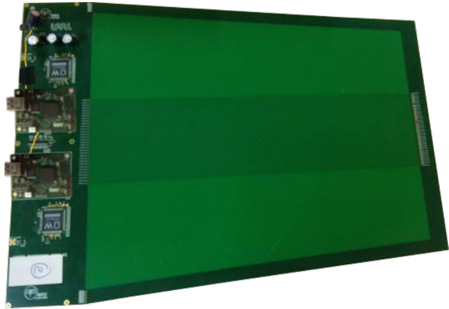
Fig. 6.2 Photo du PCB avec lecture des strips des deux côtés.
