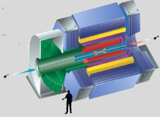
Fig. 4.5 Schéma de l'expérience BaBar.
