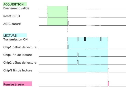
Fig. 5.17 Diagramme temporel du cycle d'acquisition et de lecture.
