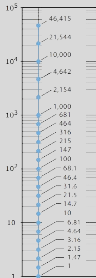
Fig. 5.43 Les 24 valeurs d'atténuation configurables.
