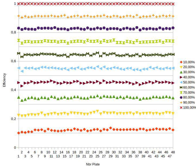
Fig. 5.20 Efficacités obtenues avec le processeur Analysis pour les 48 chambres du SDHCAL en utilisant la simulation SimDigital . Les particules incidentes sont des muons de 100 GeV et chaque couleur représente une carte d'efficacité fixée lors de la simulation.
