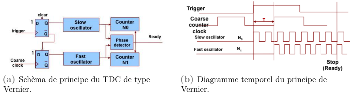
Fig. 7.1 Schéma de principe et diagramme temporel du principe des TDC utilisant le principe de Vernier. Le temps calculé par le TDC est donné par T = N_0 T_{slow} - N_1 T_{fast} avec N_0 ( N_1 ) le nombre d'oscillations de l'oscillateur lent (rapide).
