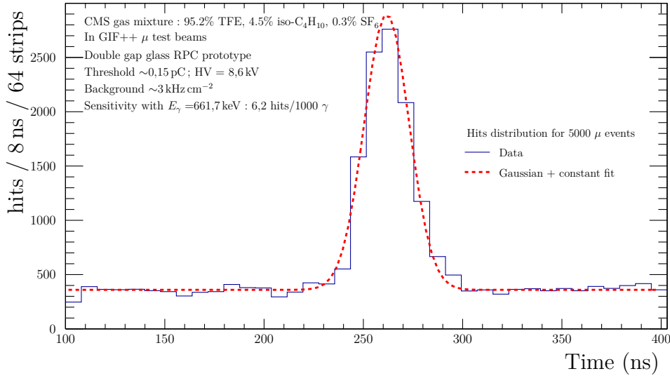
Fig. 5.85 Distribution temporelle des hits . La distribution correspond à 5000 événements déclenchés par des muons. La tension appliquée est fixée à 8,6 kV et le seuil à 0,15 pC. Le signal provenant des muons est observé autour de t_0 = 270 ns et peut être ajusté par la somme d'une Gaussienne de résolution \sigma = 11 ns et d'une constante. La zone du signal correspond à une fenêtre de \pm 3\sigma autour de t_0 . Le flux de \gamma de la source est estimé à 3 kHz cm -2 .
