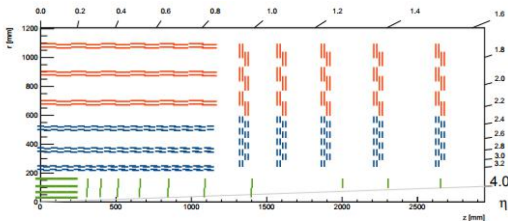
Fig. 3.35 Schéma d'un quart du trajectographe prévu pour la mise à niveau de CMS [21].
