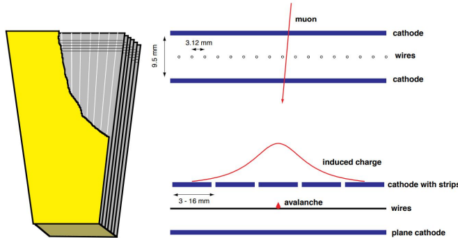
Fig. 3.30 Schéma d'une chambre CSC [17].
