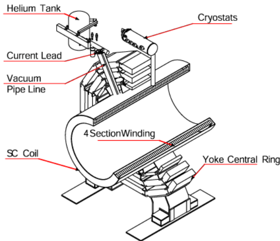
Fig. 3.23 Schéma de l'aimant supraconducteur de CMS [14].
