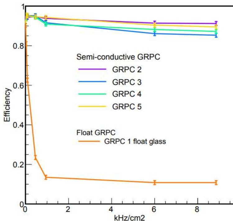
Fig. 5.24 Efficacité en fonction du flux de particules pour différentes GRPC. La ligne orange correspond à une chambre composée de verre "Standard" dit float glass de résistivité de l'ordre de \sim 10^{13} \Omega \text{ cm} . Les autres courbes correspondent à des chambres composées de verre de basse résistivité.
