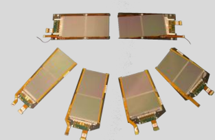
Fig. 3.7 Différents modules utilisés pour la construction du TOB et du TEC.
