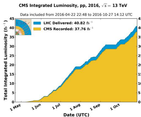
Fig. 2.20 Luminosité intégrée en fonction du jour de l'année 2016 délivrée (bleu) et enregistrée (orange) par CMS pendant les faisceaux stables et pour les collisions pp , à 13 TeV d'énergie dans le centre de masse [4].
