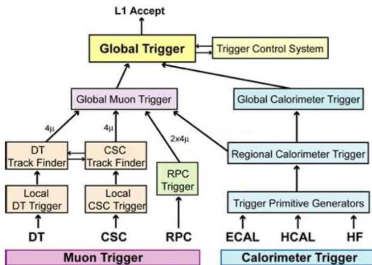
Fig. 3.34 Schéma du Level-1 Trigger (L1) [18].
