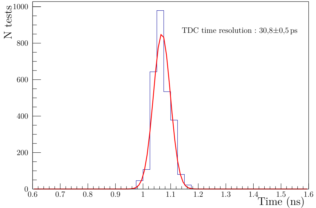
Fig. 6.7 Résolution temporelle d'un strip du PCB. Le signal est un échelon de tension d'amplitude 10 V et de durée 10 ns. Le signal traverse un condensateur de 1 pF.
