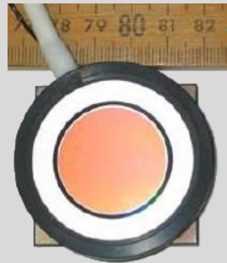
Fig. 3.18 Photo d'un MPPC.
