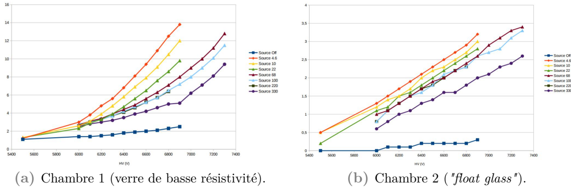
Fig. 5.55 Intensité parcourant les chambres en fonction de la haute tension appliquée pour différentes valeurs du facteur d'atténuation de la source.
