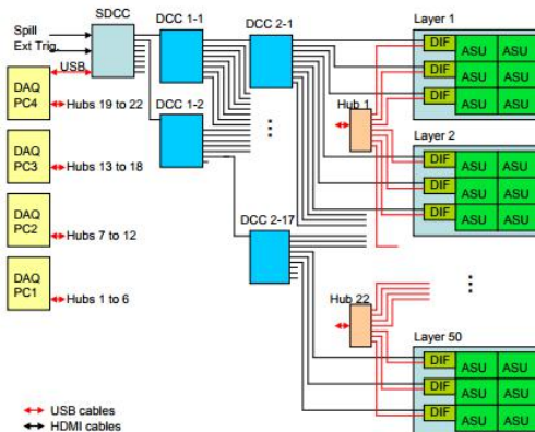
Fig. 5.19 Architecture de la DAQ du SDHCAL. Dans notre cas le nombre d'ASU est d'un par layer (chambre) ainsi que d'une DIF par chambre. Le nombre de chambres étant dans notre cas inférieur à 9, l'utilisation des DCC est inutile.
