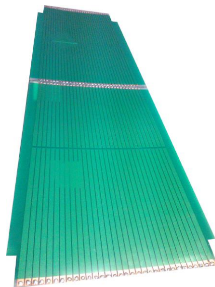
Fig. 5.61 Les 4 partitions de 32 strips selon \eta .
