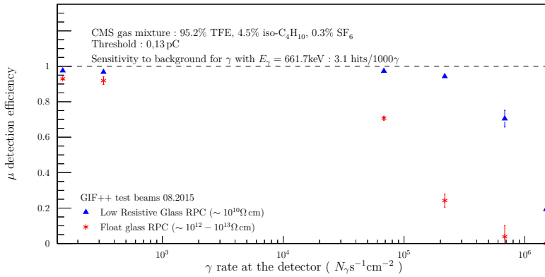
Fig. 5.47 Efficacité en fonction du courant de \gamma obtenue pour différentes valeurs d'atténuation de la source. Les effets d'écrantage dus à la présence des autres chambres placées devant la source ne sont pas inclus.
