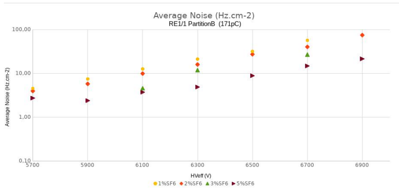
Fig. 5.91 Taux de bruit dans la partition B de la chambre RE1/1 en fonction de la tension appliquée pour différentes proportions de \text{SF}_6 . Le seuil appliqué est de 0,17 pC.
