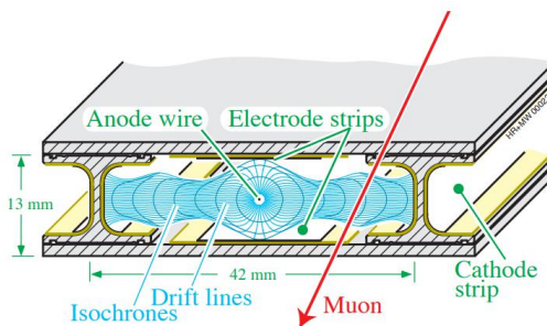
Fig. 3.29 Schéma d'un tube d'une chambre à dérive [16].
