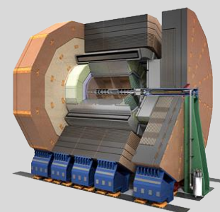
Fig. 5.4 Photo du prototype SDHCAL construit à Lyon.
