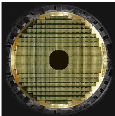
(b) Un bouchon du ECAL (EE).
