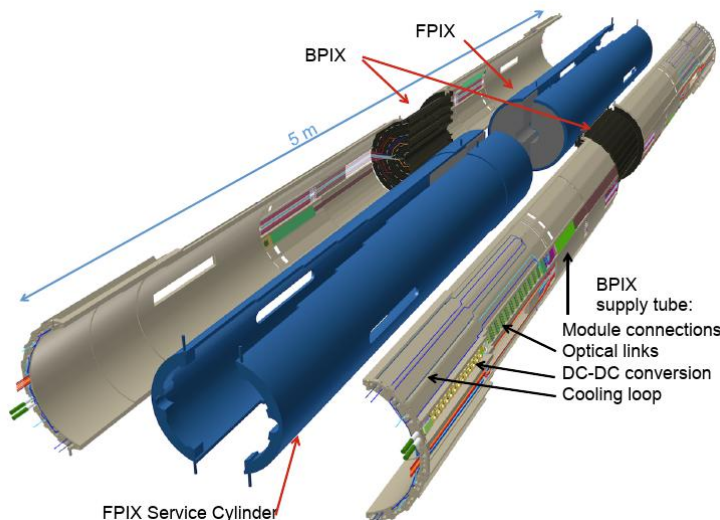
Fig. 3.5 Vue explosée du nouveau détecteur à pixels. La figure montre les positions des différentes partitions FPIX et BPIX ainsi que leurs cylindres contenant leurs services respectifs. Les services nécessaires au détecteur (connectiques, fibres optiques, convertisseurs DC-DC) sont situés à haut \eta , hors du volume de trajectographie [11].
