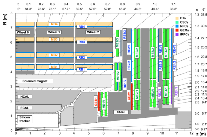
Fig. 3.37 Schéma d'un quart du détecteur CMS montrant les différentes technologies qui seront utilisées dans les bouchons du spectrographe à muons [20].
