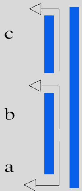
Fig. 4.25 Schéma d'une chambre RPC dans les bouchons [45].
