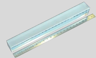
Fig. 3.10 Un cristal de \text{PbWO}_4 .
