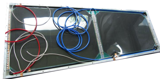
(b) Gap(ii) et gap(iii) hermétiques formés par collage des verres dans la cassette, avec les strips et le gap(i) au dessous.
