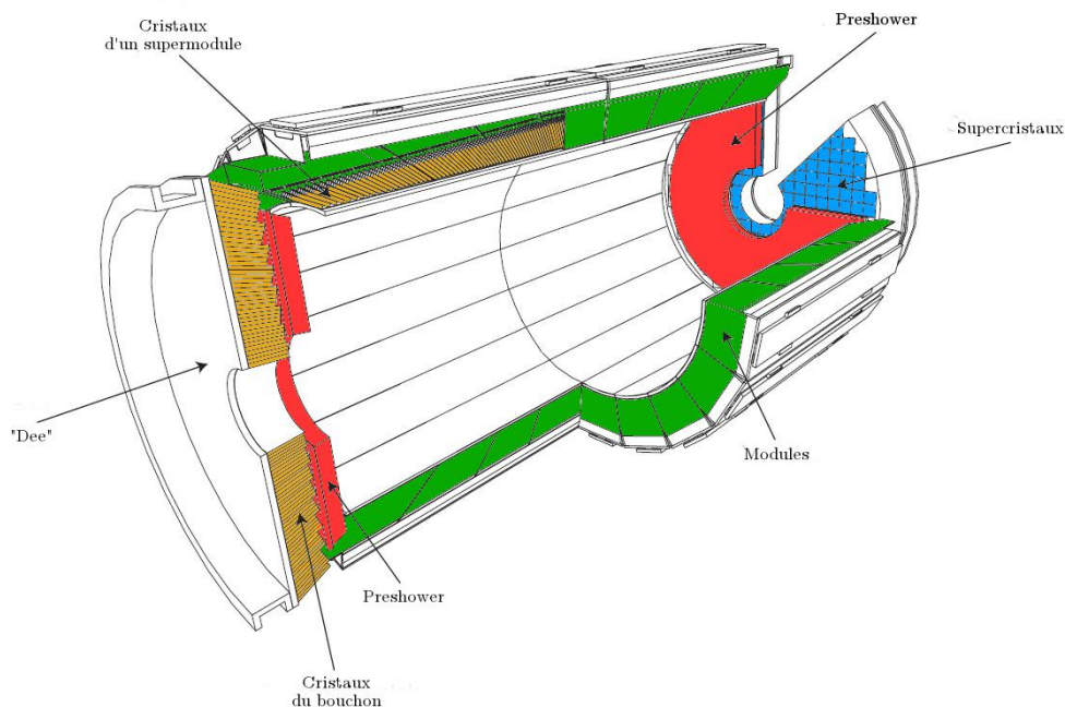
Fig. 3.9 Schéma du ECAL de CMS [12].
