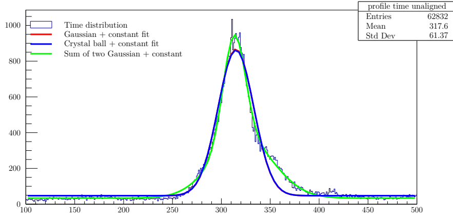
Fig. 5.80 Distribution du nombre de hits par timestamp des strips non-alignés et ajustement de cette distribution par la somme d'une gaussienne et d'une constante (vert), la somme de deux gaussiennes et d'une constante (rouge) et une Crystal-Ball (bleu).
