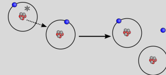
Fig. 4.10 Éjection d'un électron Auger.
