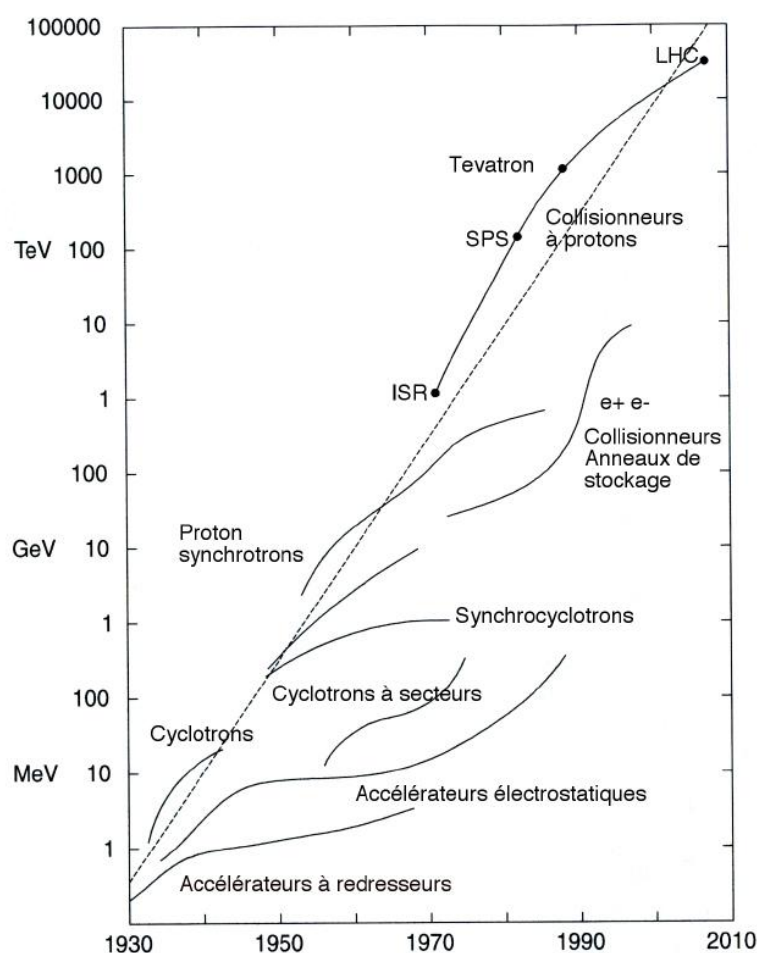
Fig. 2.7 Diagramme de LIVINGSTON : énergie des faisceaux de particules accélérées pour différentes machines en fonction du temps. Afin de pouvoir comparer les différents accélérateurs et technologies, l'énergie des collisionneurs, qui s'exprime dans le centre de masse, a été recalculée comme si l'énergie des particules observées était le résultat d'une collision avec un proton au repos (cible fixe).
