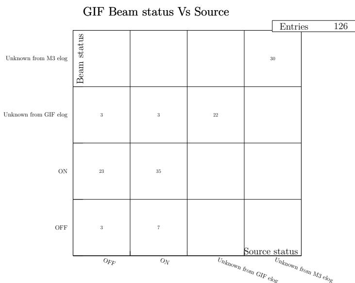
Fig. 5.98 Corrélation entre le statut du faisceau et le statut de la source pour les 126 runs ayant été inscrits dans le bon elog. 30 runs ont été écrits dans le mauvais elog (M3) suite à une erreur de configuration.
