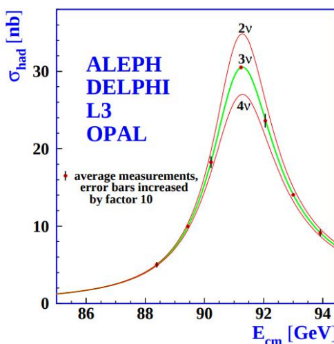
Fig. 1.24 Mesures de la section efficace de production hadronique près de la résonance du Z^0 . Les courbes indiquent les sections efficaces prédites pour deux, trois et quatre espèces de neutrinos de masses négligeables avec les couplages du Modèle Standard [3].
