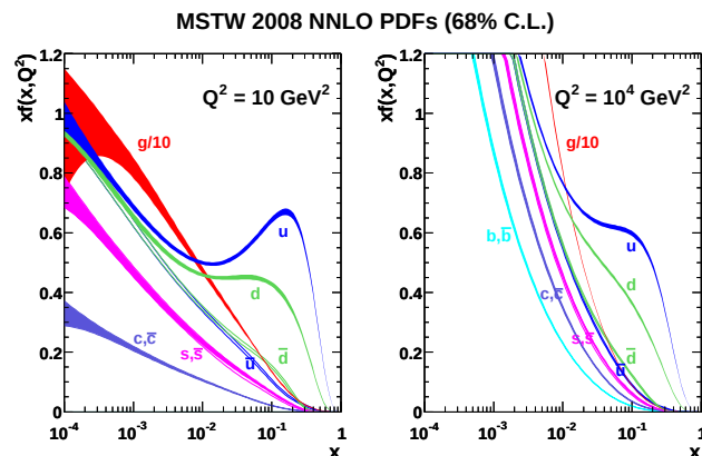
Fig. 2.22 Produit de x avec la distribution de parton non-polarisée f(x) , où f = u, \bar{u}, d, \bar{d}, c, \bar{c}, s, \bar{s}, b, \bar{b}, g et leurs incertitudes, en utilisant la paramétrisation NNLO MSTW2008 à l'échelle 10 \text{ GeV}^2 (gauche) et 10\,000 \text{ GeV}^2 (droite) [5].
