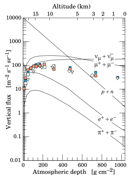
Fig. 5.65 Composition du flux cosmique dans l'atmosphère terrestre pour des particules ayant une énergie supérieure à 1 GeV. Les points colorés représentent les mesures de flux de muons négatifs réalisées par plusieurs expériences [29].
