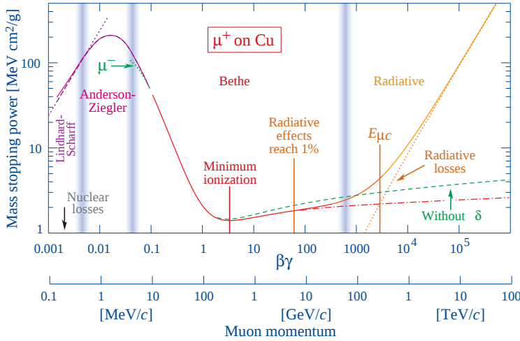
Fig. 4.8 Perte d'énergie moyenne -\left\langle \frac{dE}{dx} \right\rangle pour des anti-muons dans du cuivre en fonction de \beta\gamma = \frac{p}{Mc} sur neuf ordres de grandeur en quantité de mouvement (douze ordres de grandeur en énergie cinétique)[29].
