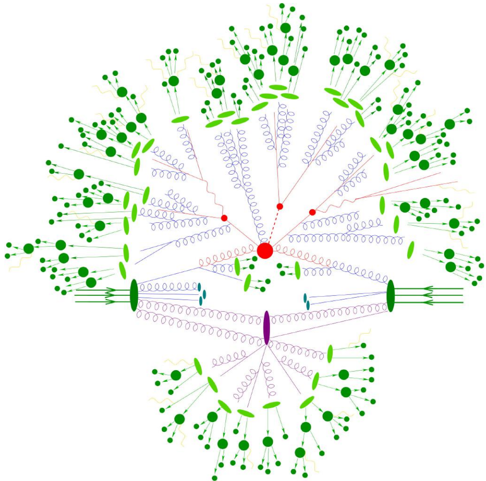
Fig. 2.24 Schéma d'une collision proton-proton inélastique. Deux partons venant de deux protons différents interagissent inélastiquement (rouge), d'autres partons de ces deux protons produisent des collisions secondaires (magenta). Les partons ainsi créés s'hadronisent (rouge) en créant des jets de particules (vert clair). Ces particules instables se désintègrent, en cascade, en particules stables (vert foncé).
