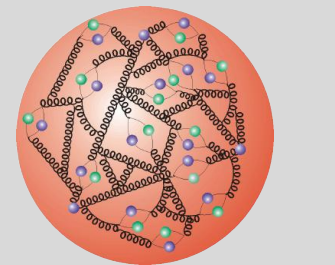
(d) Interaction forte : confinement.
