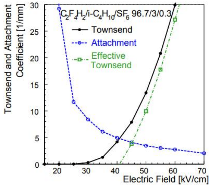
Fig. 4.19 Coefficient de TOWNSEND et coefficient d'attachement calculés grâce à Imonte [35] pour T = 296,15 K et p = 1013 mbar pour un mélange de gaz donné [34].
