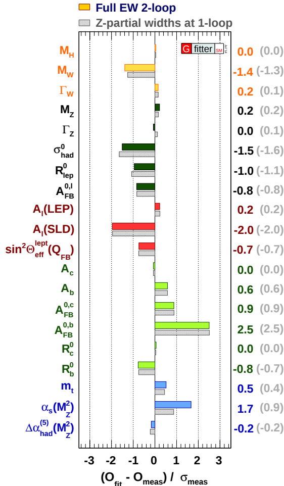
Fig. 1.21 Comparaison des résultats d'ajustement avec les mesures directes de certains paramètres du Modèle Standard [2].
