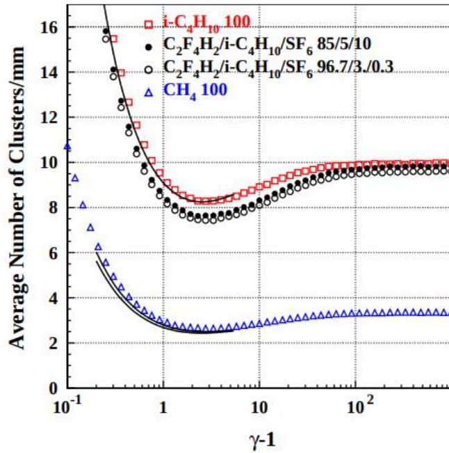
Fig. 4.17 Nombre de collisions donnant lieu à des ionisations (nombre d'amas) par mm en fonction de \gamma - 1 , avec \gamma = \frac{1}{\sqrt{1-\beta^2}} , pour différents mélanges de gaz, tel que prédit par HEED [31], avec T = 296,15 K et p = 1013 mbar. Les lignes correspondent à des mesures prises de [33].
