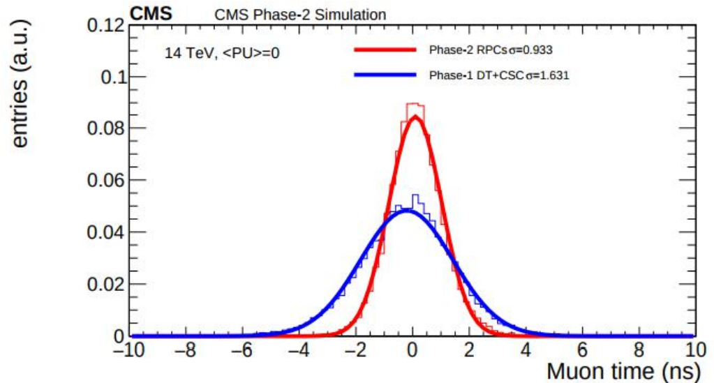
Fig. 4.32 Résolution temporelle simulée pour des traces de muons dans la région vers l'avant, dans le cas où seules sont présentes les chambres CSC et DT (bleu), et dans le cas où les chambres RPC des zones RE3/1 et RE4/1 sont incluses (rouge) [49].
