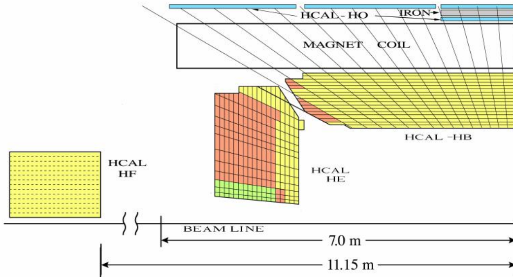
Fig. 3.20 Schéma en coupe d'un quart du HCAL de CMS [13].
