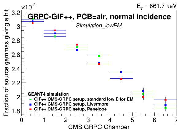
Fig. 5.49 Taux de conversion : probabilité qu'un photon de 661,7 keV produise un hit dans les chambres du télescope au GIF++. Les chambres sont numérotées de 0 à 6, la chambre 0 étant la plus proche de la source.
