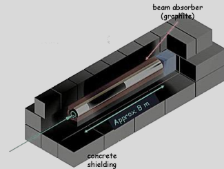
Fig. 2.19 Schéma d'un "dump block".
