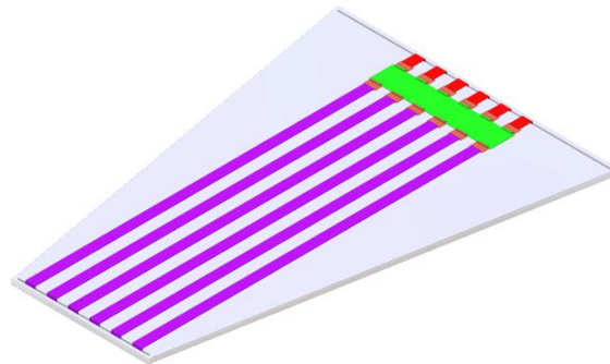
Fig. 7.2 Schéma d'une chambre iRPC avec l'électronique PETIROC2. La mezzanine est en vert. Les câbles coaxiaux venant des deux côtés des strips (en violet et en rouge) sont connectés à la mezzanine par des cartes adaptatrices d'impédance (en orange). Le détecteur et le PCB avec les strips sont à l'intérieur de la mécanique et ne sont pas visibles.
