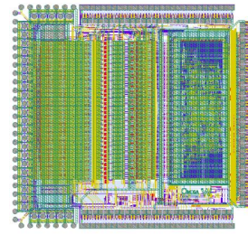
Fig. 6.4 Schéma électronique du PETIROC2.
