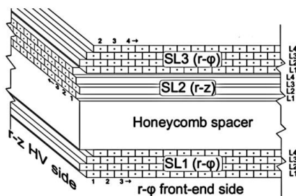
Fig. 3.28 Schéma d'une chambre à dérive [16].
