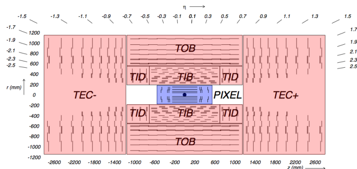
Fig. 3.3 Schéma du trajectographe de CMS. Chaque trait représente un module du détecteur. Les lignes doubles correspondent à des modules mis dos-à-dos produisant des hits dits "stéréos". Le détecteur à pistes est composé de quatre sous-détecteurs : les tonneaux internes (TIB), les tonneaux externes (TOB), les disques internes (TID) et les bouchons (TEC).
