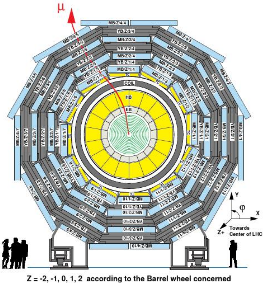
Fig. 3.27 Coupe transversale de la partie centrale de CMS [16].
