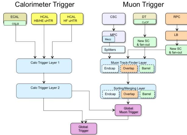
Fig. 3.36 Schéma du nouveau L1 pour la partie calorimètre et muons [22].
