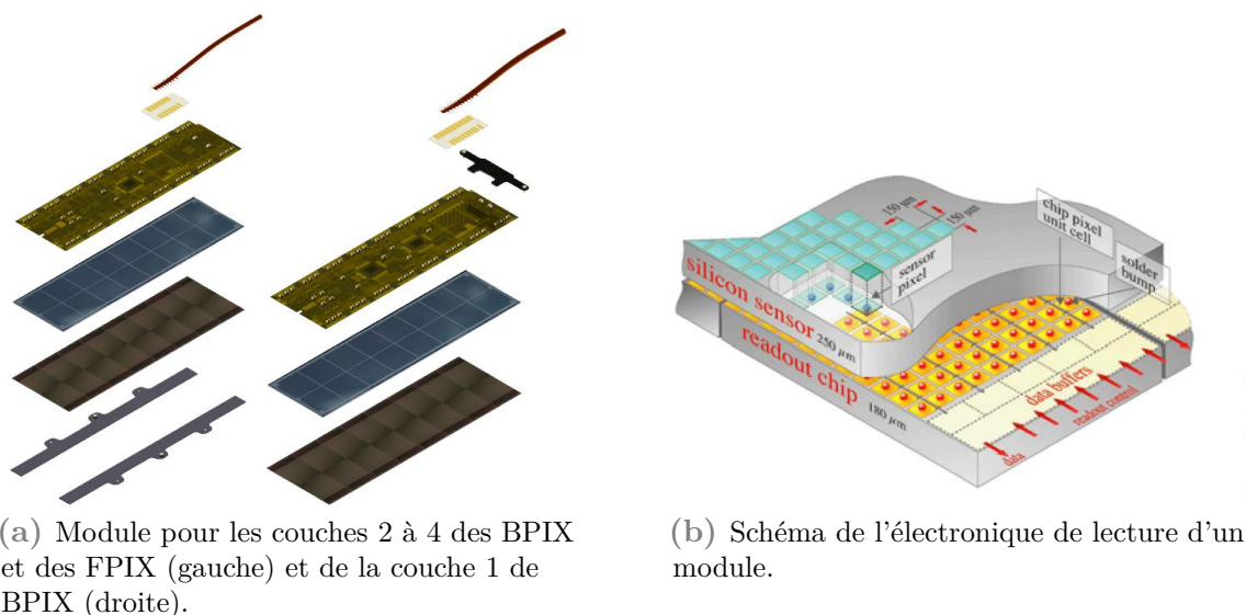
Fig. 3.6 Modules de pixels [11].
