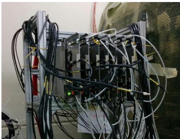
Fig. 5.45 Le télescope dans le bunker du GIF++.
