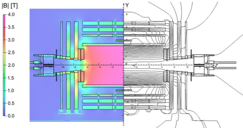
Fig. 3.24 Valeur du champ magnétique (gauche) et lignes de champ (droite) selon une coupe longitudinale du détecteur CMS, prédits par la simulation pour une valeur du champ central de 3,8 T [15].
