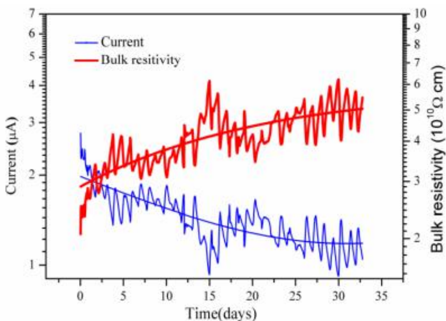
Fig. 5.1 Évolution du courant (courbe bleue) et de la résistivité volumique (courbe rouge) en fonction du temps pour une électrode de verre de basse résistivité soumise à une tension de 1000 V pendant 32 jours.
