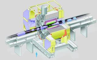
Fig. 4.5 Schéma de l'expérience BaBar.
