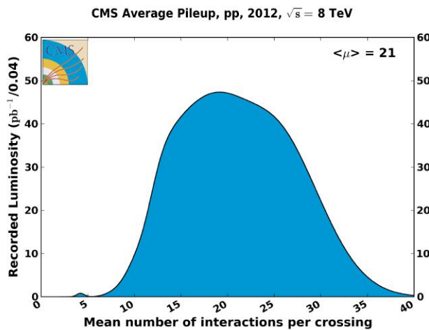
Fig. 2.25 Distribution du nombre de collisions par croisement de faisceaux [4].
