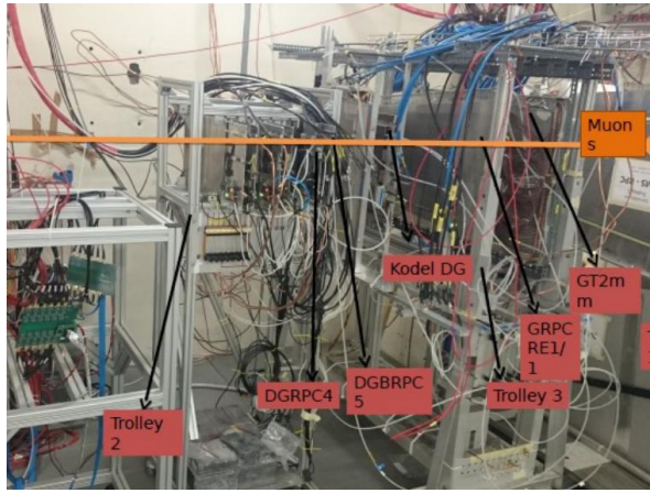
Fig. 5.95 Les nouvelles chambres à strips sur leur bâti.
