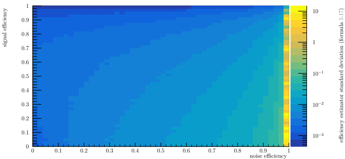
Fig. 5.83 Déviation standard du biais de la formule 5.17. 2 500 000 expériences ont été réalisées au total, réparties dans 50×50 bins.
