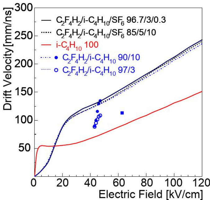
Fig. 4.20 Vitesses de dérive calculées en utilisant le programme MAGBOLTZ [37] pour différents mélanges de gaz à la température T = 296,15 K et la pression p = 1013 mbar.
