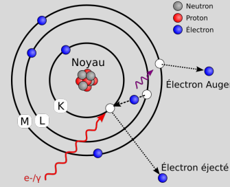
Fig. 4.9 Émission d'un photon lors de la désexcitation d'un atome.
