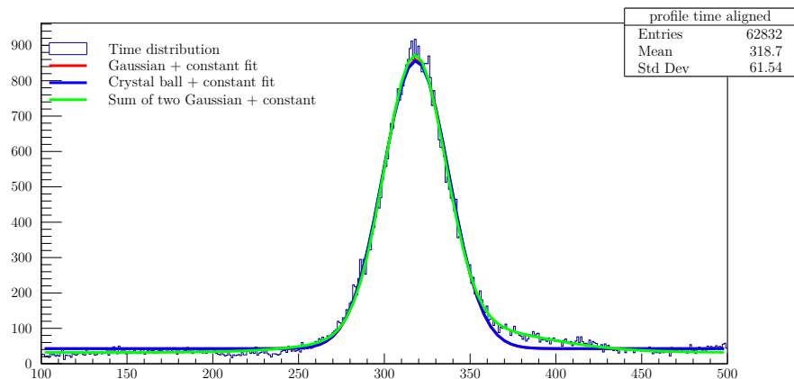
Fig. 5.79 Distribution du nombre de hits par timestamp des strips alignés et ajustement de cette distribution par la somme d'une gaussienne et d'une constante (vert), la somme de deux gaussiennes et d'une constante (rouge) et une Crystal-Ball (bleu).
