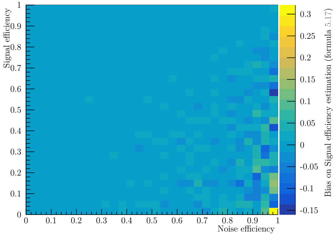
Fig. 5.82 Biais ( \epsilon_{vrai} - \epsilon_{corrigée} ) pour la formule 5.17 de correction de l'efficacité. \epsilon_{vrai} est l'efficacité réelle sans contamination par le bruit et \epsilon_{corrigée} = \epsilon_2 est l'efficacité trouvée après avoir appliqué la formule 5.17. Les courbes sont obtenues par un programme Monte Carlo où le nombre de triggers a été fixé à 50 000.
