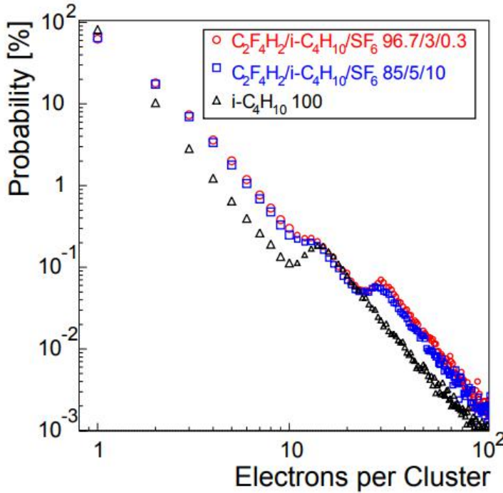
Fig. 4.18 Distributions du " cluster size " pour un mélange gazeux typique utilisé pour les RPC calculées en utilisant HEED [31]. Les particules incidentes sont des pions de 7 GeV pour le mélange avec 10% d'isobutane et 120 GeV pour le mélange avec 0,3%. La température du gaz est T = 296,15 K et la pression p = 1013 mbar. En coupant à 500 électrons et par intégration on trouve un nombre d'électrons moyen par amas de 1,9 pour l'isobutane, 2,6 pour le mélange à 10% de \text{SF}_6 et 2,8 pour le mélange à 0,3% de \text{SF}_6 .
