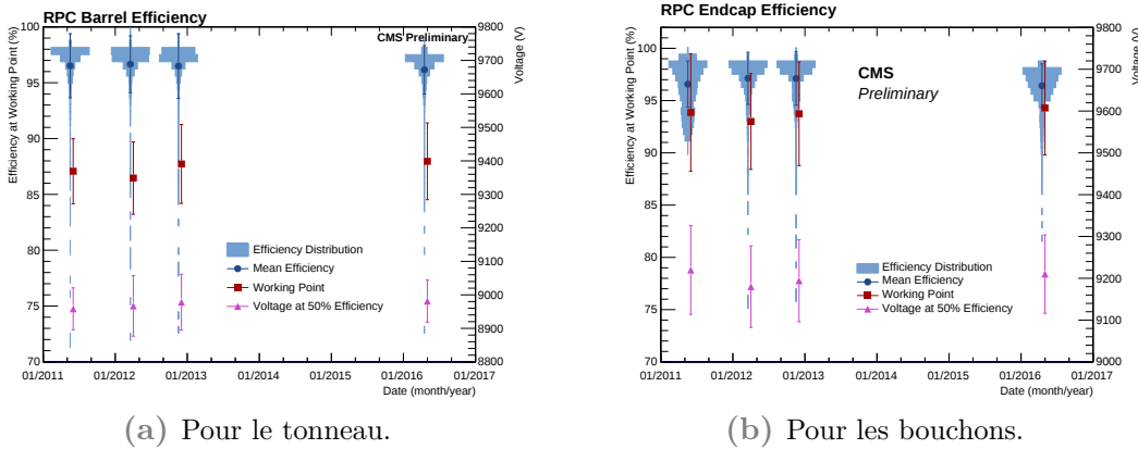
Fig. 4.31 Point de fonctionnement moyen, efficacité moyenne au point de fonctionnement et tension moyenne pour laquelle l'efficacité est de 50% pour les différents scans en tension effectués depuis 2011 [48].
