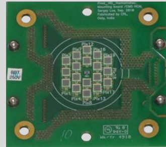
Fig. 3.17 Photo d'une tuile du HO avec des fibres WLS insérées dans les 4 \sigma -rainures.
