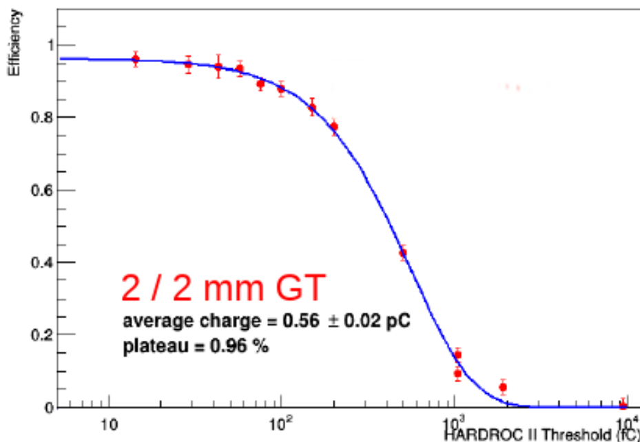
Fig. 5.102 Efficacité en fonction du seuil appliqué pour la chambre en Bakélite. La tension appliquée est fixée à 9300 V.
