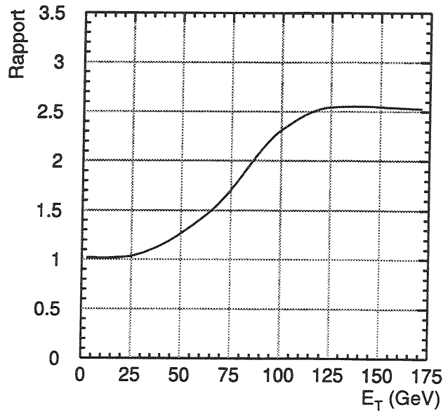
FIG. 6.9 - « Rapport de la prédiction du modèle de Glauber (avec absorption nucléaire) à la distribution d\sigma_{\mu\mu}^{J/\psi}/dE_{\perp} . »
