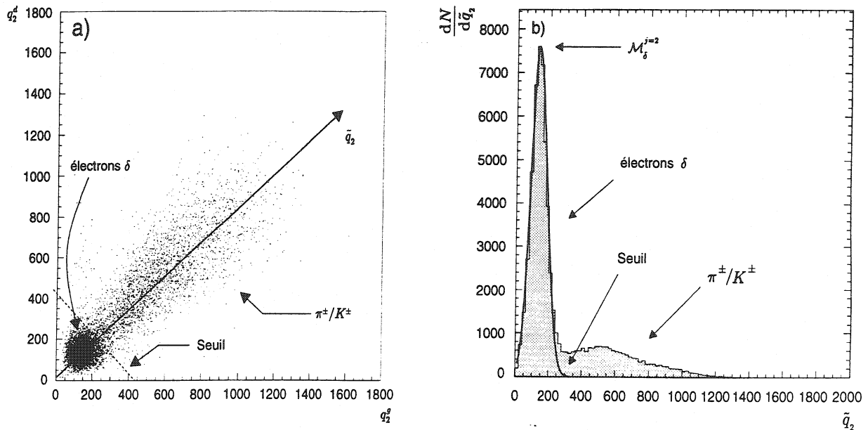
FIG. 3.6- a - « Corrélation ( q_2^d, q_2^g ) des signaux délivrés par les lames 2 droite et gauche. »
