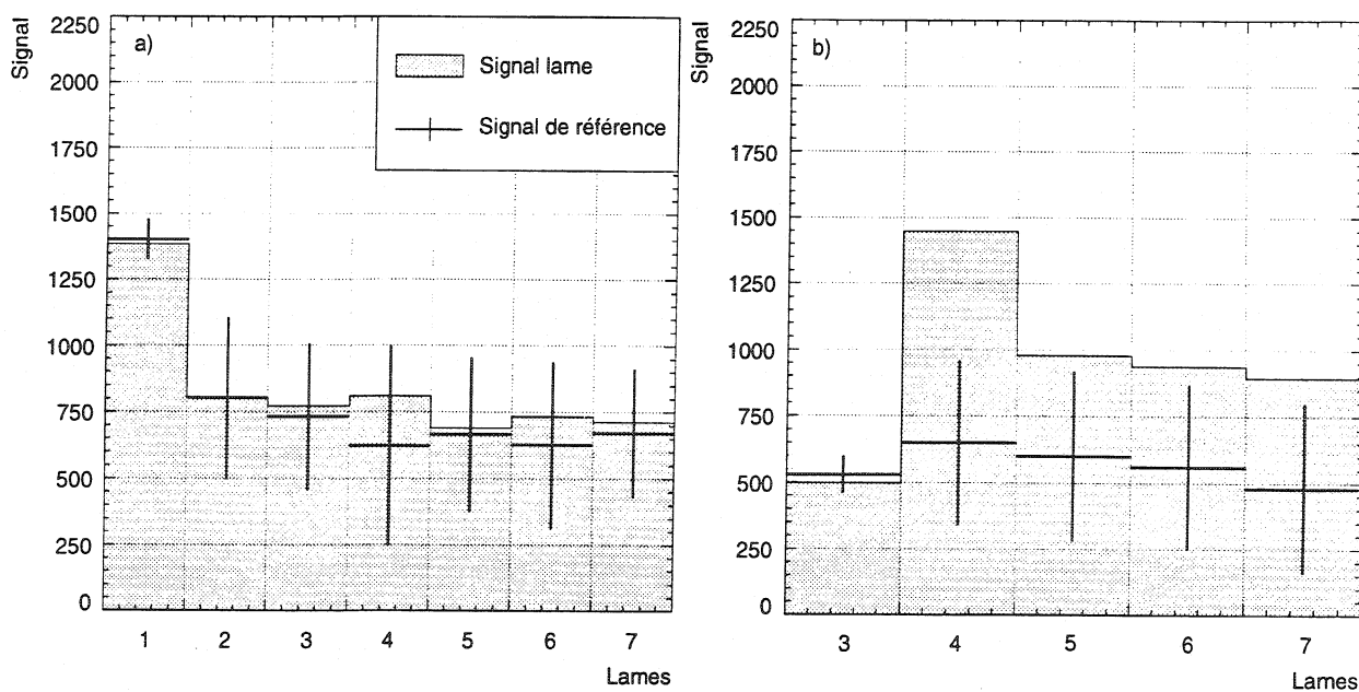
FIG. 3.12- a - « Événement typique avec une interaction dans la ciblette 1, sans réinteraction. » b - « Événement typique avec une interaction dans la ciblette 3 et une réinteraction dans la ciblette 4. La réinteraction se manifeste par des signaux tous au dessus des signaux de référence à partir d'une certaine paire de lames. »
