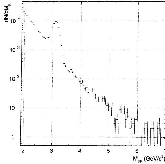
FIG. 4.5 - « Spectre en masse invariante ( M_{\mu\mu} > 1.9 \text{ GeV}/c^2 ) des muons \mu^+\mu^- produits dans les interactions Pb-Pb à 158 \text{ GeV}/c par nucléon. »
