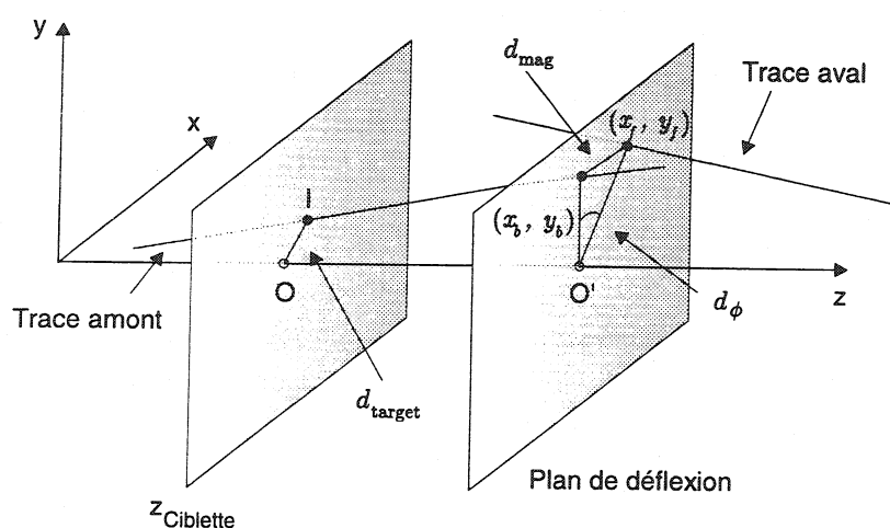
FIG. 4.3 - « Coupures géométriques. »
