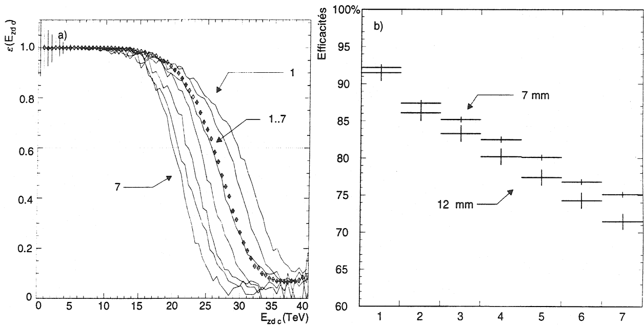
FIG. 3.9- a - « Efficacités d'identification du vertex en fonction de E_{zdc} et des 7 ciblettes (d'épaisseur 1 mm). L'efficacité de reconnaissance toutes ciblettes confondues est indiquée par les losanges. » b - « Efficacités intégrées ciblette par ciblette, pour une cible de 7 mm (points supérieurs) et de 12 mm (points inférieurs). »
