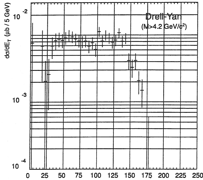
FIG. 6.2 - « Dépendance en énergie transverse de la section efficace de production du processus Drell-Yan ( M_{\mu\mu} \geq 4.2 \text{ GeV}/c^2 ) dans les interactions Pb-Pb à 158 GeV/c par nucléon. Chaque intervalle en E_{\perp} représente 5 GeV. »
