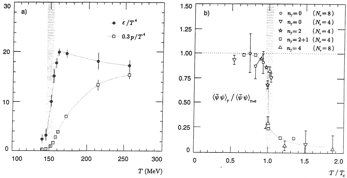
FIG. 1.3- a - « Densité d'énergie \epsilon et pression p , rapportées à T^4 , en fonction de la température T , calculées sur réseau avec deux saveurs de quarks. Extrait de [Karsh95]. » b - « Evolution avec la température du paramètre d'ordre \langle \bar{\psi}\psi \rangle de la symétrie chirale, calculée sur réseau avec plusieurs saveurs de quarks. Extrait de [Karsh95]. »
