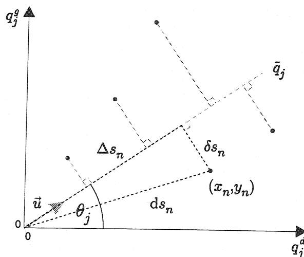
FIG. A.1 - « Représentation partielle du nuage de points (q_j^d, q_j^g) . La droite principale du nuage de points est la droite qui minimise la somme des carrés des distances \delta s_n . »
