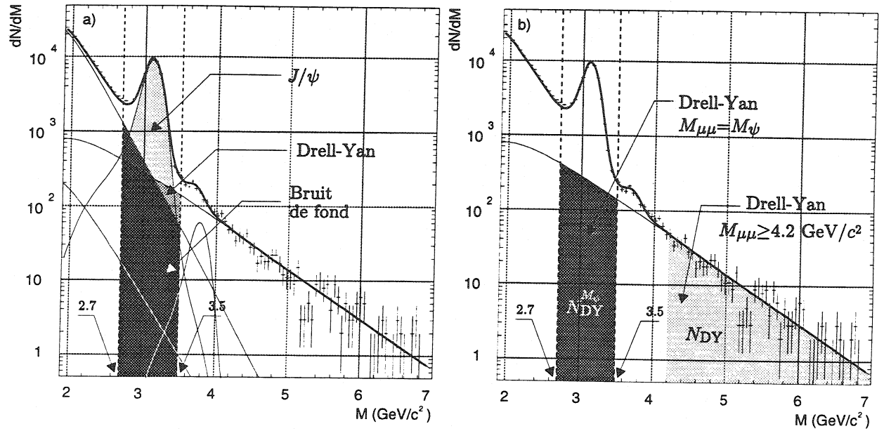
FIG. 6.3- a - « Distribution en masse invariante des dimuons de signe opposé. Dans la zone de masse M_\psi = [2.7 \dots 3.5] ( \text{GeV}/c^2 ) la distribution est la somme des contributions dues à la désintégration du J/\psi , au processus Drell-Yan, à la désintégration du \psi' , à la production de charme D\bar{D} et au bruit de fond. Les contributions \psi' et D\bar{D} sont négligées pour le calcul de la dépendance en énergie transverse de la section efficace de production du J/\psi . » b - « La distribution en énergie transverse du processus Drell-Yan dans le région de masse M_\psi = [2.7 \dots 3.5] ( \text{GeV}/c^2 ) est égale à la distribution en énergie transverse au-delà de 4.2 \text{ GeV}/c^2 , normalisée par le rapport N_{\text{DY}}^{M_\psi} / N_{\text{DY}} . »
