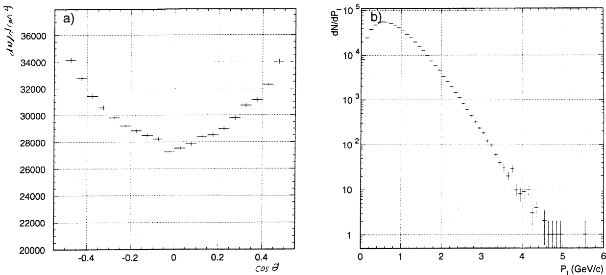
FIG. 4.11- a - « Distribution en \cos(\theta) générée des dimuons provenant du processus Drell-Yan. » b - « Distribution en p_\perp générée des dimuons provenant du processus Drell-Yan. »
