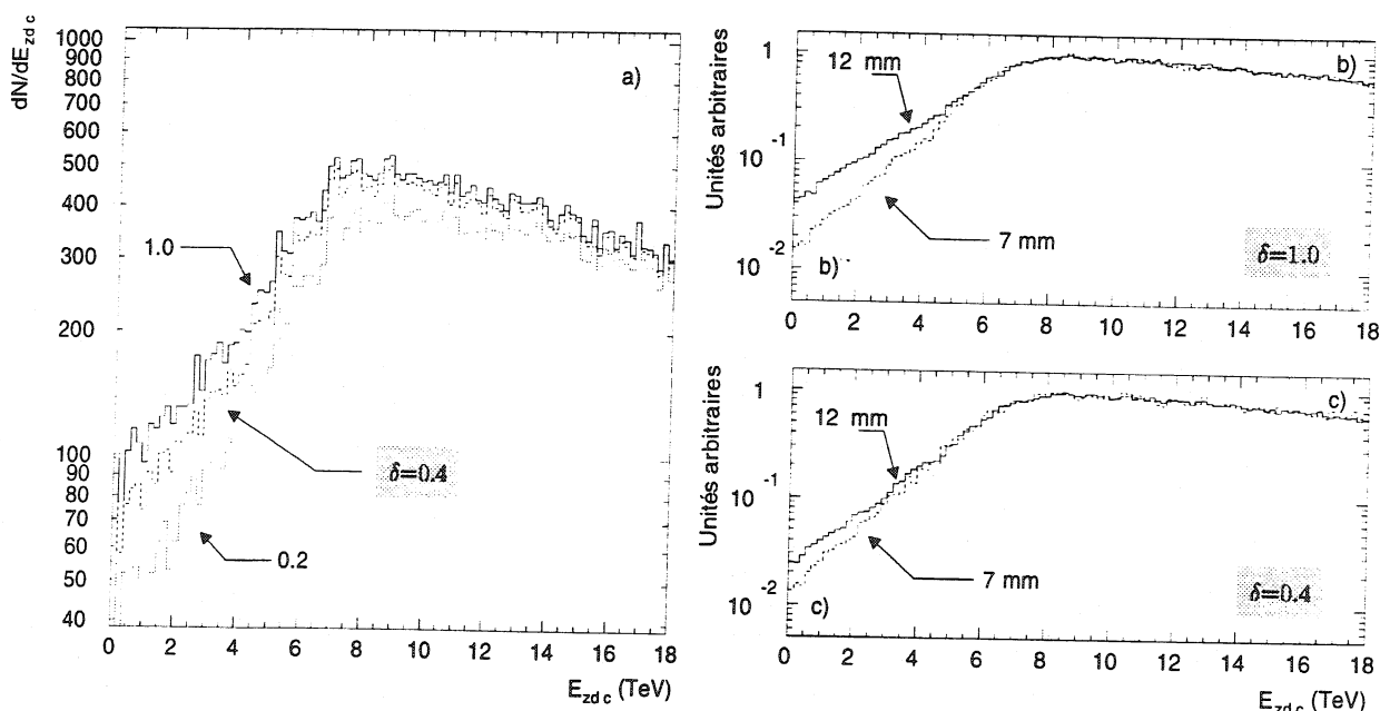
FIG. 3.14- a - « Effet de la coupure \delta_{cut} ( 0.2 \leq \delta_{cut} \leq 1 ) sur la distribution en énergie E_{zdc} (interactions dans la première ciblette, suivie de 11 mm de plomb en aval). » b - « Distributions en E_{zdc} pour une cible de 7 mm et de 12 mm d'épaisseur, avant coupure. » c - « Distributions en E_{zdc} pour une cible de 7 mm et de 12 mm d'épaisseur, après coupure. »
