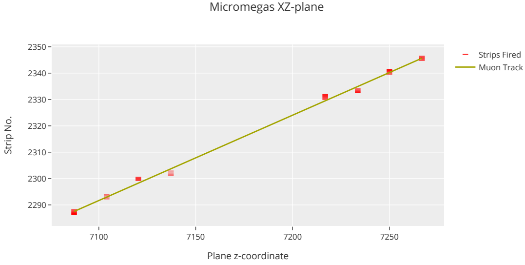
Figure 4.: La trajectoire des muons à travers un secteur MicroMegs est représentée en vert, les bandes déclenchées étant représentées par des lignes horizontales rouges
