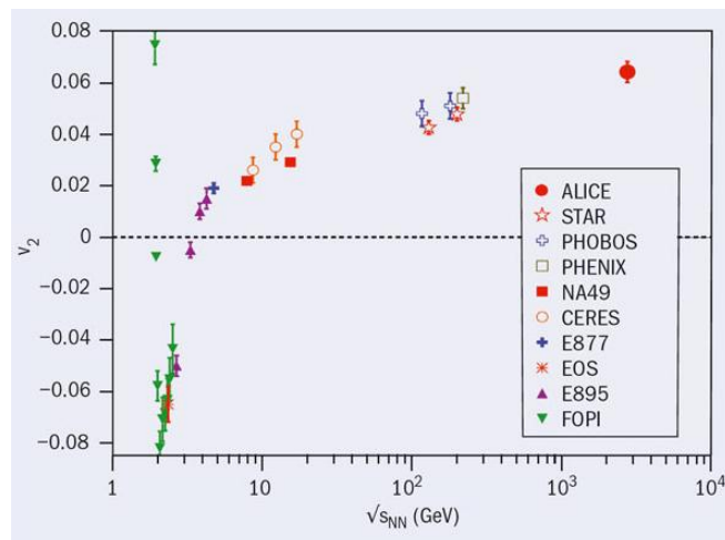
Figure 18 : Flot elliptique mesuré par l'expérience ALICE pour des collisions Pb-Pb à \sqrt{s_{NN}} = 2.76 TeV pour une classe de centralité intermédiaire (20-30%) et comparaison avec les résultats d'autres expériences à plus basse énergie.
