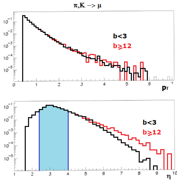
Figure 85 : Distribution en impulsion transverse (figure du haut) et en pseudo-rapidity (figure du bas), des \mu provenant de la désintégration des \pi et K , normalisées à une particule, avant l'application des coupures de sélection des \mu .
