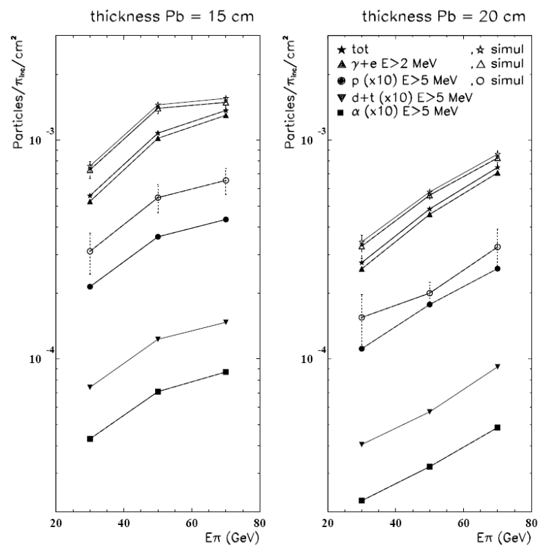
Figure 70 : Nombre de particules produites par \pi incident et par \text{cm}^2 en fonction de l'énergie incidente du faisceau de \pi . Comparaison avec une simulation GEANT.
