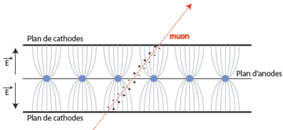
Figure 45 : Principe de fonctionnement d'une chambre à fils à cathodes segmentées.
