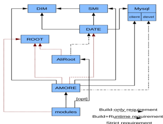
Figure 98 : Schéma représentant les dépendances de AMORE par rapport aux autres logiciels utilisés dans ALICE.
