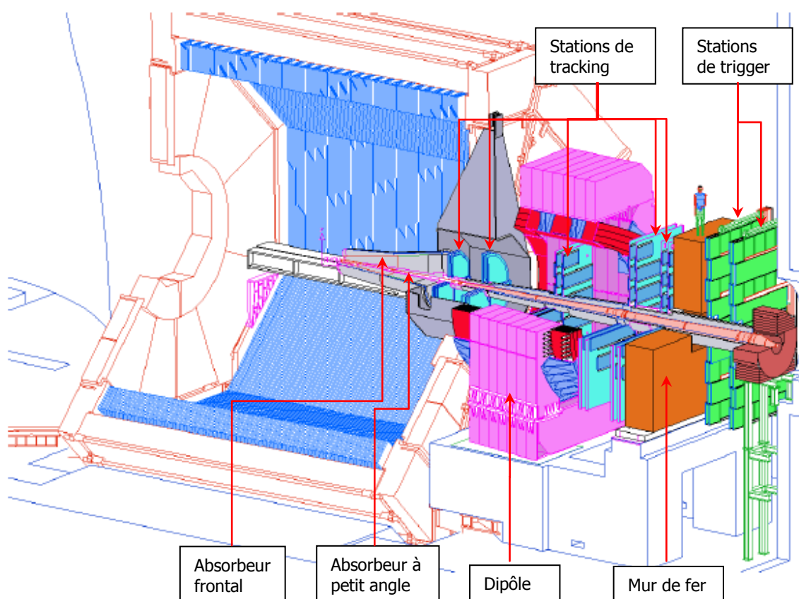
Figure 42 : Schéma du spectromètre à muons de ALICE.
