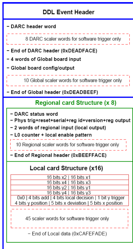
Figure 93 : Structure des données d'un DDL du Muon Trigger.
