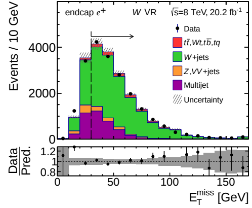
(d) Endcap electron channel in the W + jets VR.
