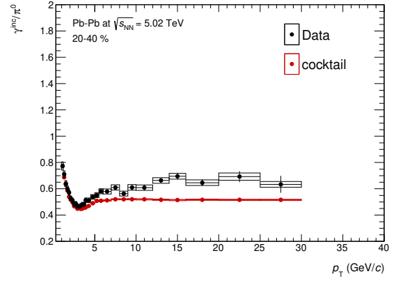
(d) The \gamma^{\text{inc}}/\pi^0 ratio in 20-40% Pb-Pb collisions.
