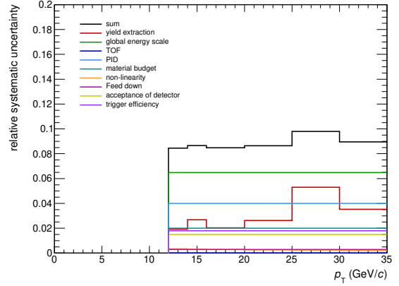
(b) kPHI7
