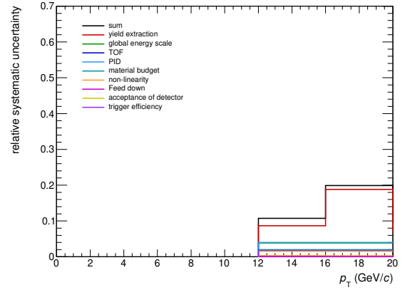
(b) kPHI7
