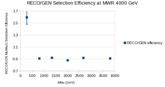
(d) Muon channel, m_{W_R} = 4 TeV
