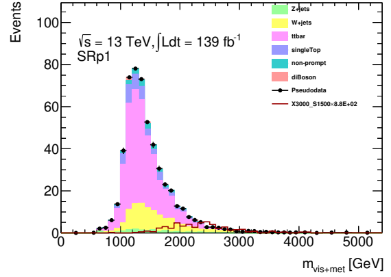
(d) SRp1, m_X = 3.0 TeV and m_S = 1500 GeV
