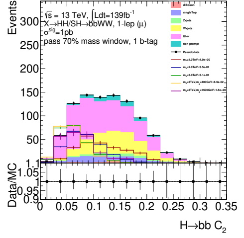
(d) SRf2, C_2^{H \rightarrow b\bar{b}}
