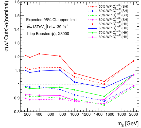
(d) SH samples with m_X = 3.0 \text{ TeV}
