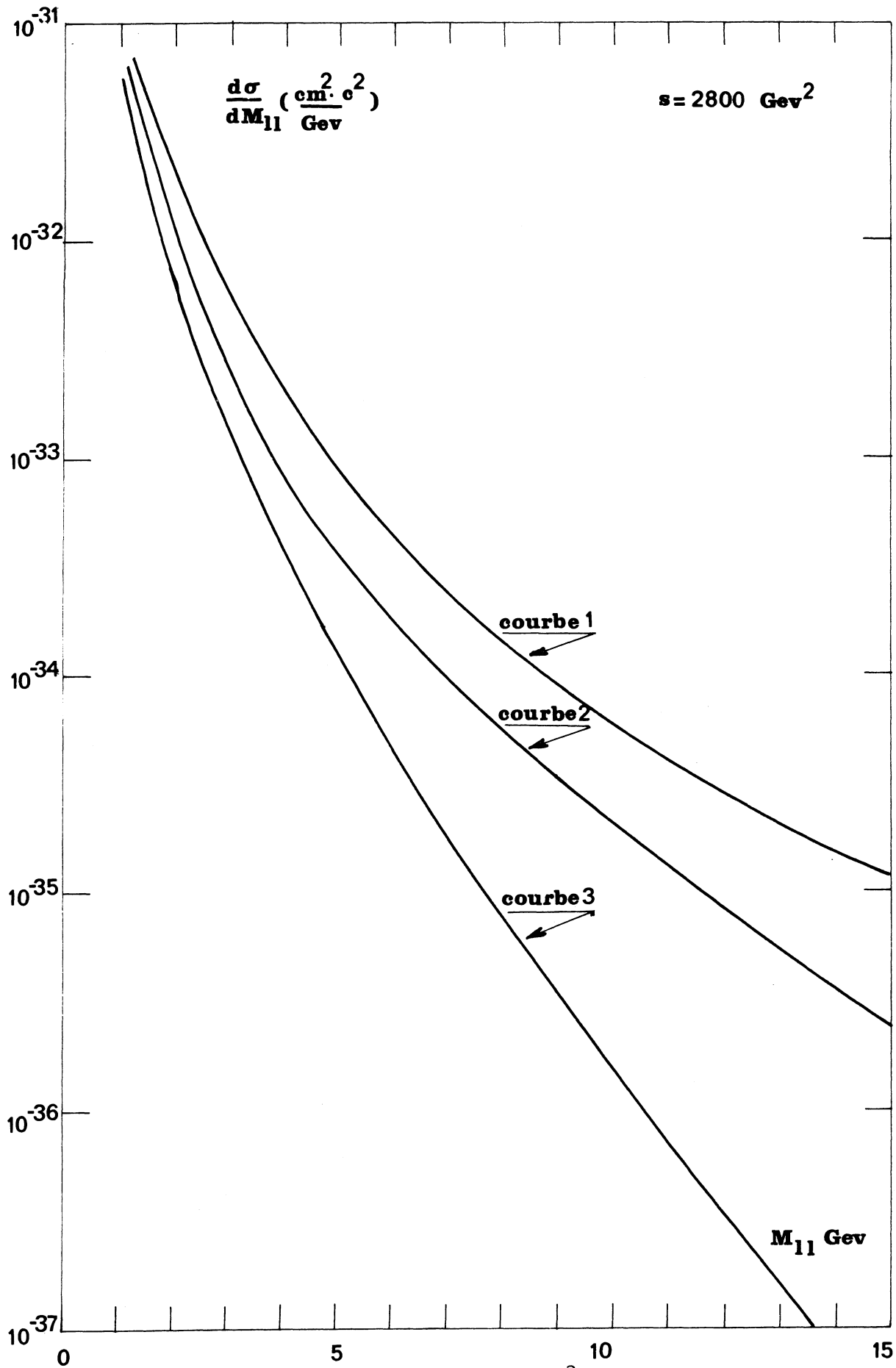
Fig. III-4 : Section efficace d\sigma/dM à s = 2800 \text{ GeV}^2 en fonction de la masse de la paire de lepton. La courbe 1 correspond au modèle de Drell et Yan La courbe 2 au modèle BBK La courbe 3 au modèle BBK modifié
