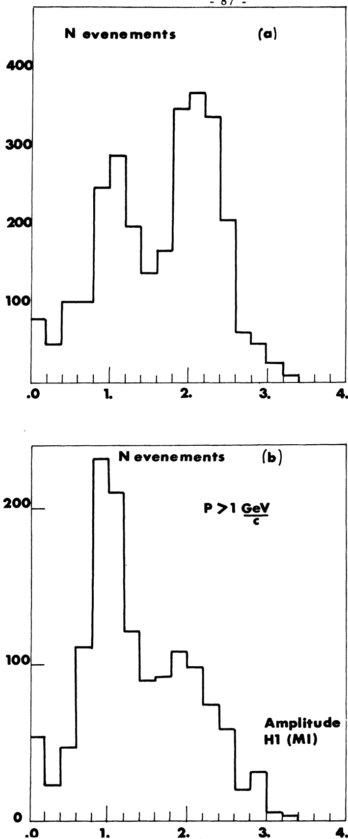
Fig. II-7 : Distribution des hauteurs d'impulsion pour les événements monotraces dans l'hodoscope H1.
