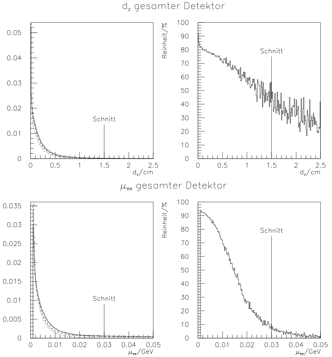
Abbildung 7.4: d_z(\mu_{ee}) -Verteilung aller Paare nach der Konversionsselektion ohne d_z(\mu_{ee}) -Schnitt in den Daten (durchgezogene Linie) und in der Monte Carlo Simulation (gestrichelte Linie, wahre Konversionen gepunktet) und die Reinheit der Paarselektion als Funktion von d_z(\mu_{ee})
