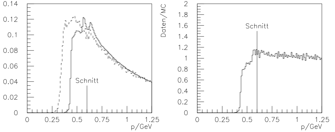
Abbildung 7.6: Impulsverteilung aller 'GAMPEX'-Photonen in den Daten (durchgezogene Linie) und in der Monte Carlo Simulation (gestrichelte Linie) und das Verhältnis aus Datenverteilung und Monte Carlo-Verteilung
