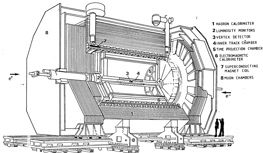
Abbildung 3.1: Querschnitt des ALEPH-Detektors [10]
