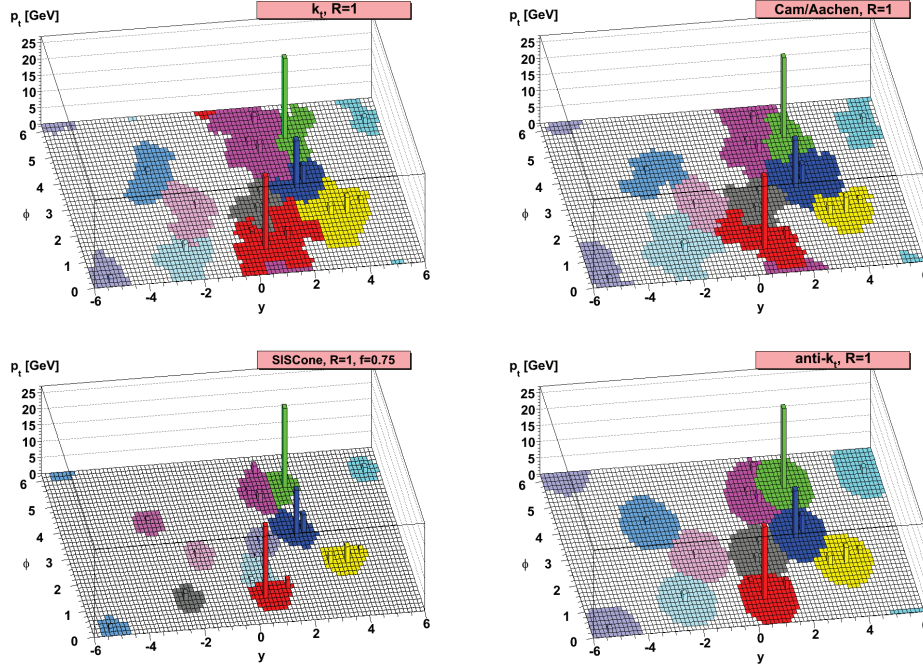
Figure 4.4: Exemple d'événements générés avec HERWIG et accompagné de fantômes aléatoirement générés. Les différentes couleurs représentent les jets avec leur aire de captage (source [51]).
