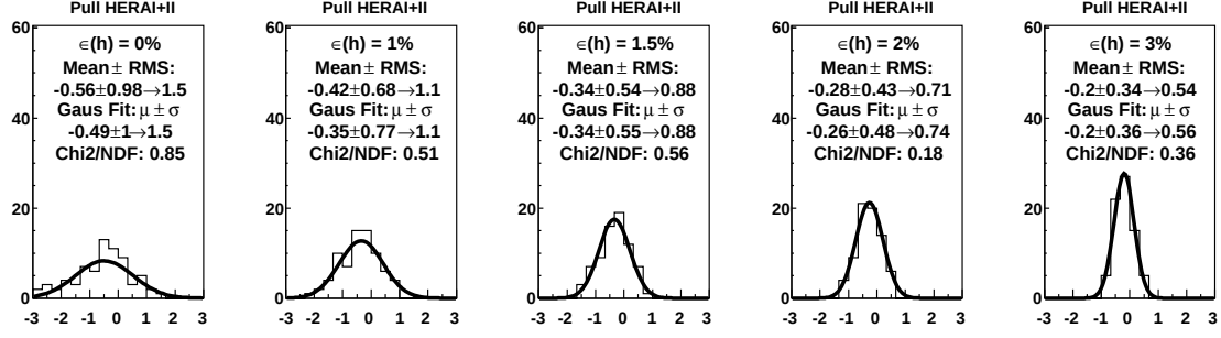
Figure 6.11: Les distributions de Pull pour différentes hypothèses de l'incertitude hadronique \epsilon_h : de gauche à droite \epsilon_h = 0\% , 1\% , 1.5\% , 2\% , 3\% .
