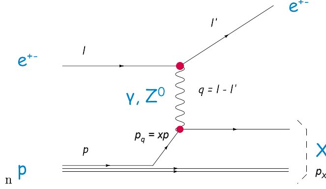
Figure 1.5: Le diagramme de la diffusion inélastique profonde en ordre dominant en \alpha_{\text{EM}} .
