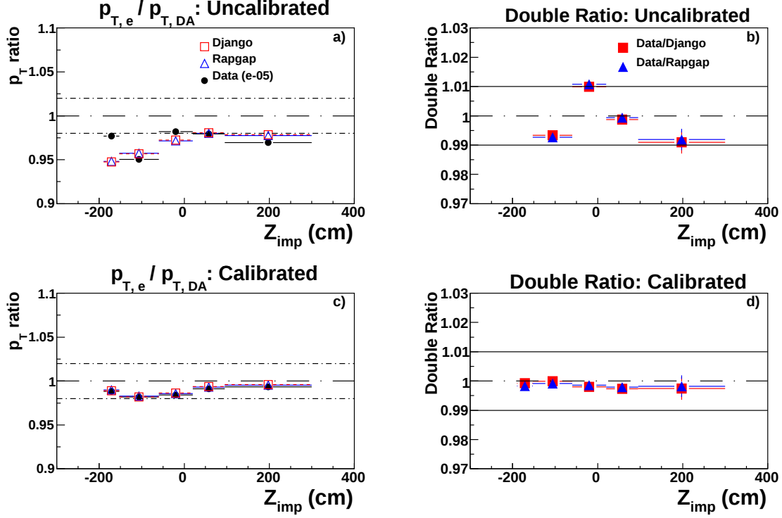
Figure 5.16: La calibration de l'électron: Ratio avant la calibration (a) et après la calibration (c) ainsi que le double ratio avant (b) et après (d) la calibration en fonction du Z_{\text{imp}} . Exemple de la période e^-05 .
