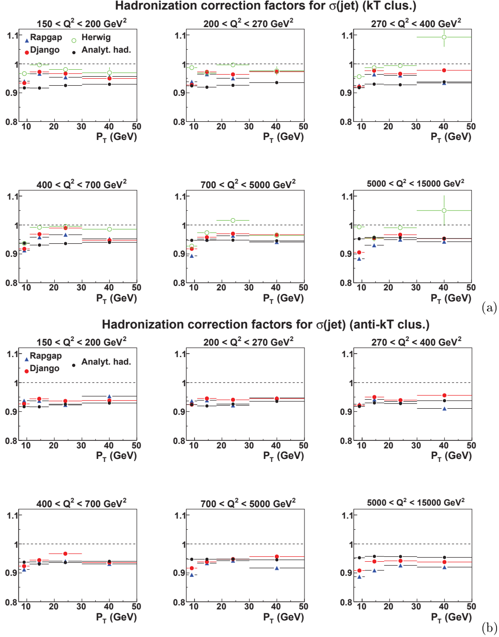
Figure 7.10: Les facteurs de correction d'hadronisation estimés en fonction de P_T dans différentes régions en Q^2 pour la section efficace inclusive jet par DJANGO (cercles rouges) et RAPGAP (triangles bleus) qui utilisent le modèle de cordes pour simuler l'hadronisation. Les facteurs du haut ont été calculés pour l'algorithme d'agrégation k_T et ceux du bas pour l'algorithme anti- k_T . Les résultats du haut sont comparés à HERWIG (cercles ouverts verts) qui utilise le modèle de cluster pour simuler l'hadronisation et ceux du haut et du bas à l'hadronisation analytique (points noirs).
