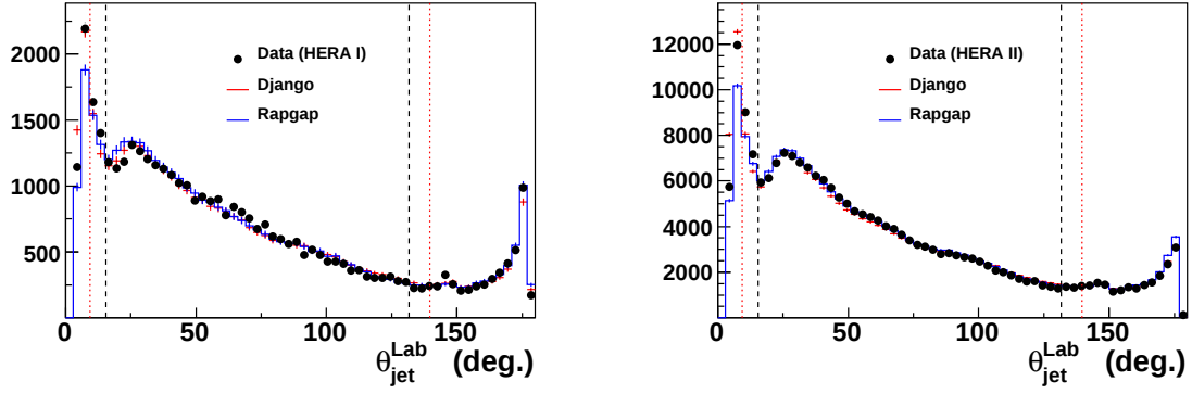
Figure 6.7: La distribution de l'angle polaire des jets inclusifs \theta_{jet}^L pour la période HERA I (a) et HERA II (b), les coupures appliquées dans notre analyse (analyse HERA I [5]) étant représentées par les lignes verticales en pointillés noirs (rouges).
