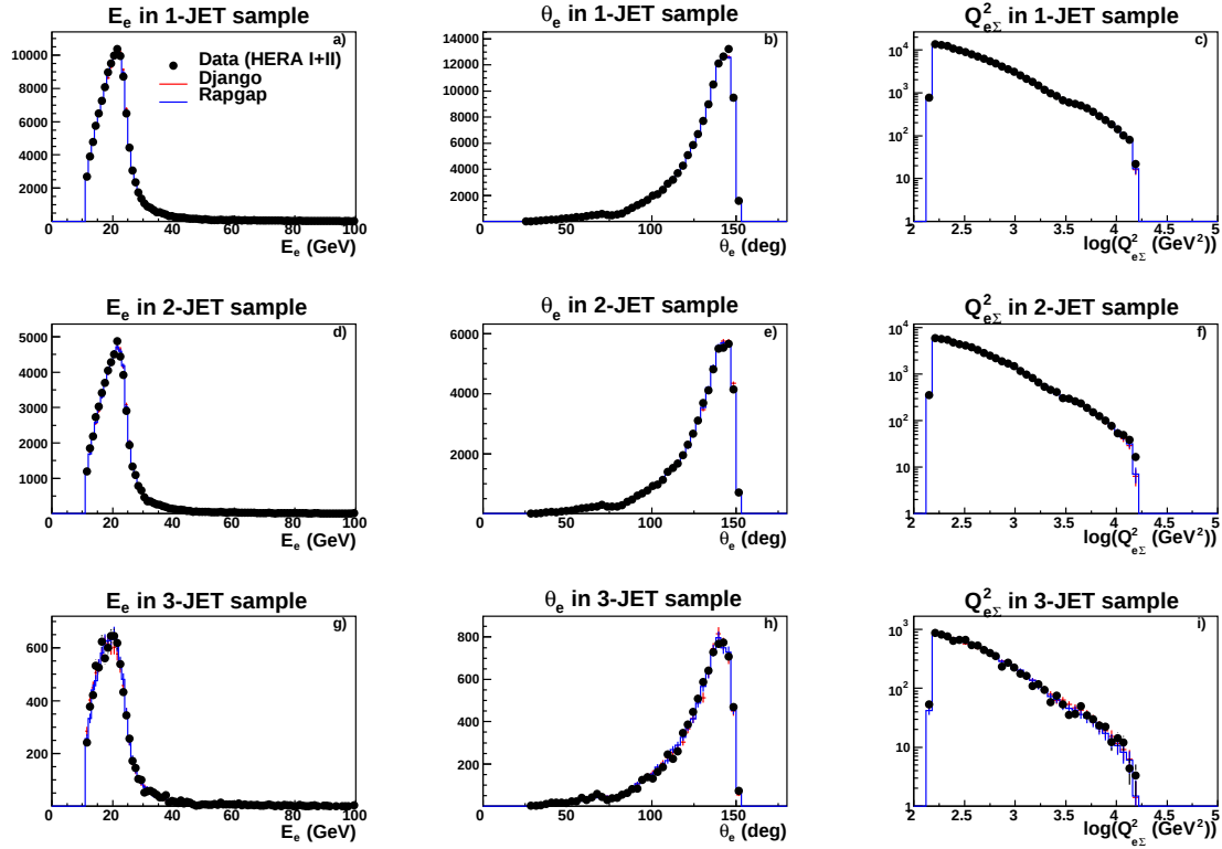
Figure 6.13: Les distributions (de gauche à droite) de E_e , \theta_e et Q^2_{e\Sigma} dans (de haut en bas) les échantillons 1-JET, 2-JET et 3-JET pour l'ensemble de la période HERA I+II. Les MC sont normalisés au nombre total d'événements dans les données.
