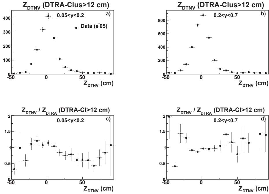
Figure 5.13: La distribution des vertices Z_{DTNV} dans l'échantillon où l'électron n'est pas associé à une trace pour les données e^-05 dans le régime faiblement inélastique 0.05 < y < 0.2 - colonne de gauche et le régime intermédiaire 0.2 < y < 0.7 - colonne de droite. Les distribution (a-b) sont normalisées à la luminosité des données alors que (c-d) sont normalisées à la distribution des vertices hadroniques Z_{DTRA} dans le même échantillon.
