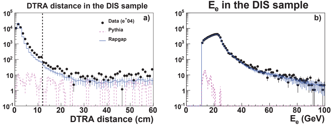
Figure 5.9: La distribution des données (points noirs) pour la période e^+04 est comparée à la simulation RAPGAP (ligne continue bleue) en DIS NC et PYTHIA (ligne en pointillés magenta) en photoproduction: (a) La distance entre la trace DTRA et le cluster électron, la ligne en tirets indiquant la coupure appliquée; (b) L'énergie de l'électron E_e une fois la coupure sur la distance DTRA appliquée. Les distributions sont normalisées à la luminosité des données. Le taux résiduel de photoproduction est négligeable après la coupure.
