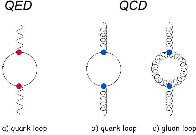
Figure 1.4: Les corrections au propagateur du photon en QED et du gluon en QCD.
