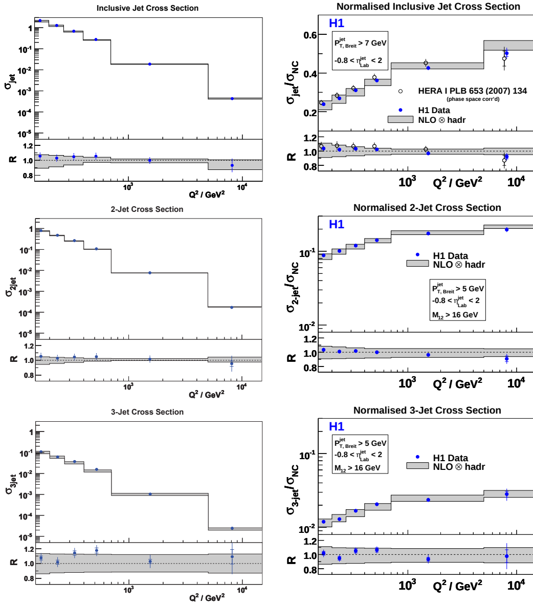
Figure 7.17: Les sections efficaces jet mesurées en fonction de Q^2 . De haut en bas sont représentées les sections efficaces inclusive jet, 2-jet et 3-jet. La colonne de droite représente les sections efficaces simples et la colonne de gauche normalisées à la section efficace DIS NC. Ces dernières sont des résultats préliminaires de la collaboration H1 [144]. Sur chaque graphique la partie supérieure représente la valeur absolue de l'observable et la partie inférieure le rapport entre les mesures expérimentales et les prédictions théoriques. Les mesures sont représentées par des points noirs positionnés au centre statistique de la case et entourés par des barres d'erreur correspondant à l'erreur statistique (barre intérieure) et à l'erreur totale (barre extérieure). Les prédictions théoriques avec leurs incertitudes sont représentées par une bande grise. Lorsqu'elles sont disponibles les mesures précédentes publiées par la collaboration H1 sont représentées par des cercles ouverts.
