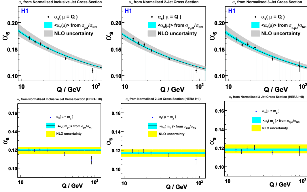
Figure 8.4: Mesures de \alpha_s(\mu) dans différentes régions en Q^2 : en haut en fonction de \mu = Q , qui correspond à la moyenne statistique du transfert d'impulsion dans chaque case; en bas extrapolé à \mu = m_Z . Les valeurs de \alpha_s(\mu = Q) sont obtenues par un fit combiné à partir de quatre points individuels pour la section efficace normalisée inclusive jet (1 ère colonne) et 2-jet (2 ème colonne), mais un seul point pour la section efficace normalisée 3-jet (3 ème colonne). Pour chaque observable les résultats sont comparés à la mesure centrale de \alpha_s(\mu_r) (courbe noire en haut et bleue en bas), obtenue en combinant les mesures individuelles par une procédure de fit, représentée avec son incertitude expérimentale (bande bleue) et théorique (bande grise en haut et jaune en bas).
