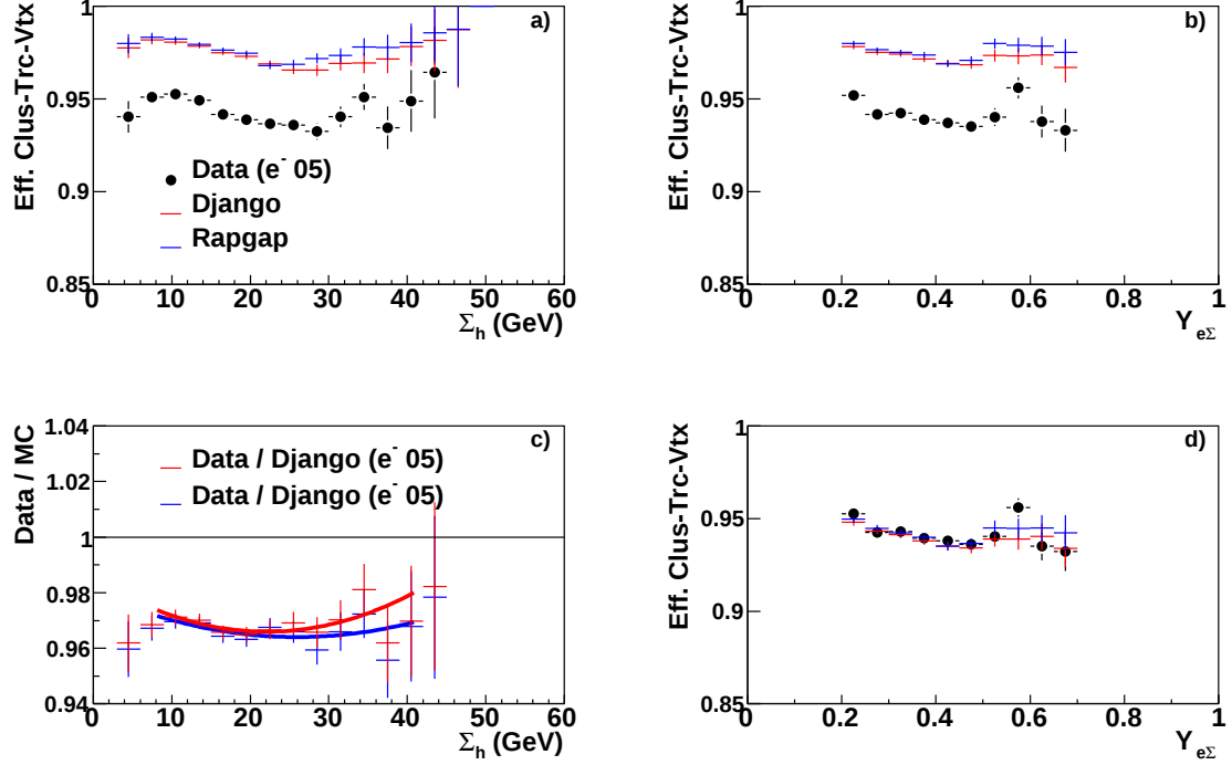
Figure 5.14: L'inefficacité de l'association vertex-trace-cluster pour la période e^- 05 en fonction de \Sigma_h avant la repondération (a) ainsi que les facteurs de correction utilisés pour la repondération (c). L'effet de la repondération sur une variable hadronique alternative y_{e\Sigma} avant la repondération (b) et après la repondération (d).
