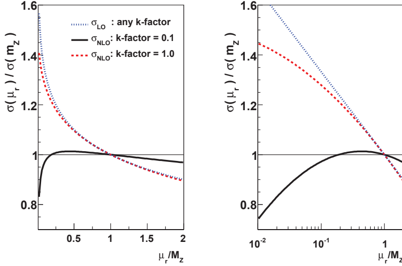
Figure 2.11: La variation des prédictions théorique à l'ordre dominant (LO) et subdominant (NLO) avec \mu_r pour deux valeurs du k-facteur k_2 = 0.1, 1 . A gauche l'échelle linéaire est utilisée et à droite l'échelle logarithmique.
