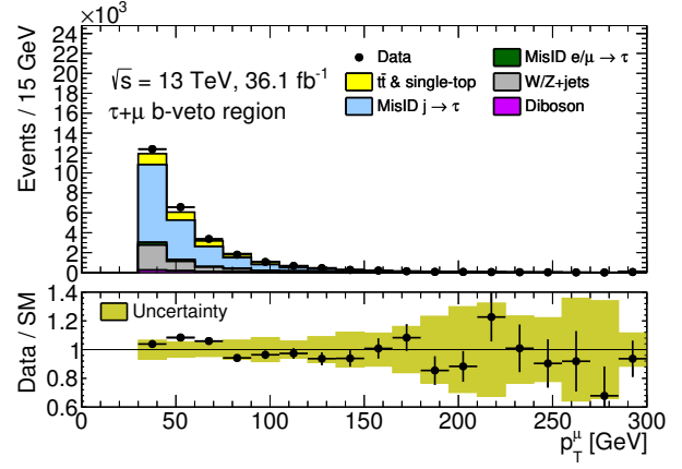
(b) p_T^\mu
