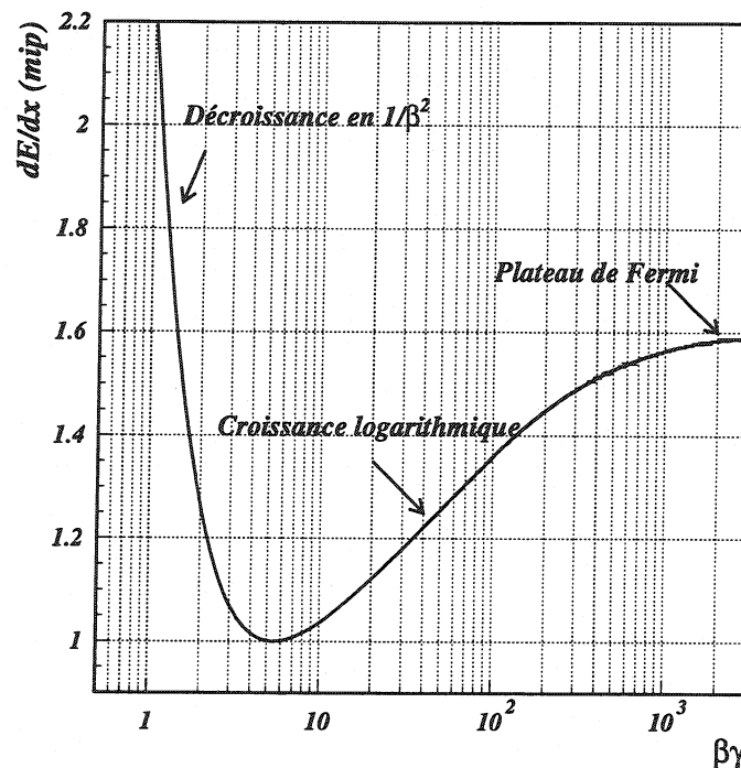
FIG. 5.5 – dE/dx en fonction de \beta\gamma .
