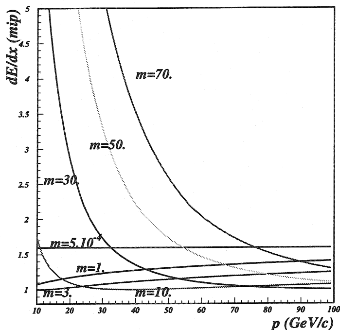
FIG. 5.8 – Perte d'énergie pour différentes hypothèses de masse ( \text{GeV}/c^2 ) en fonction de l'impulsion.
