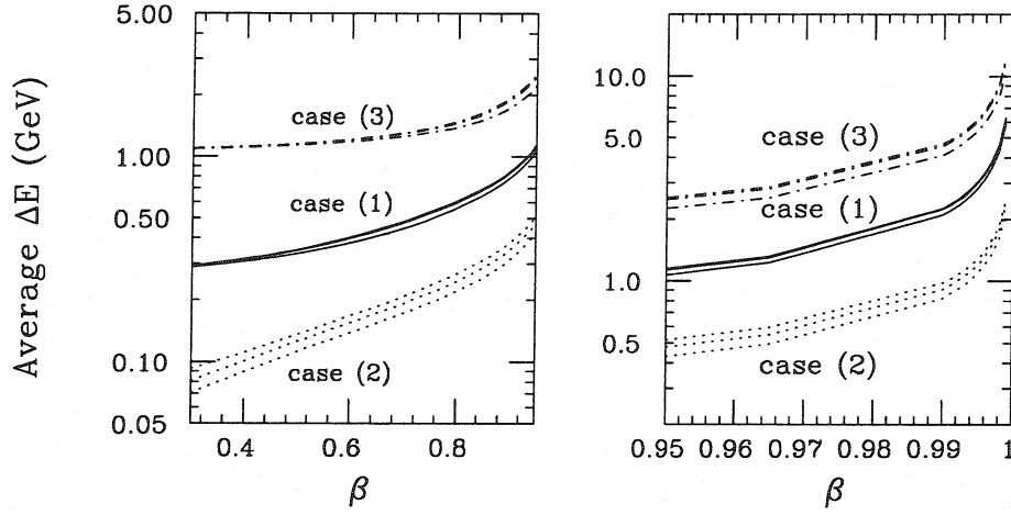
FIG. 3.3 – Perte d'énergie moyenne \langle \Delta E \rangle en fonction de la vitesse \beta du R^0 pour les trois modèles de sections efficaces et pour trois hypothèses de masse: m_{R^0} = 5, 25 et 140 \text{ GeV}/c^2 [9].
