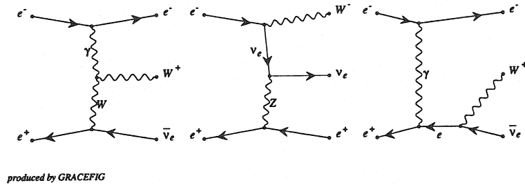
FIG. 6.7 – Diagrammes de Feynman correspondant à la production d'un seul W et donnant l'état final W\bar{\nu} .
