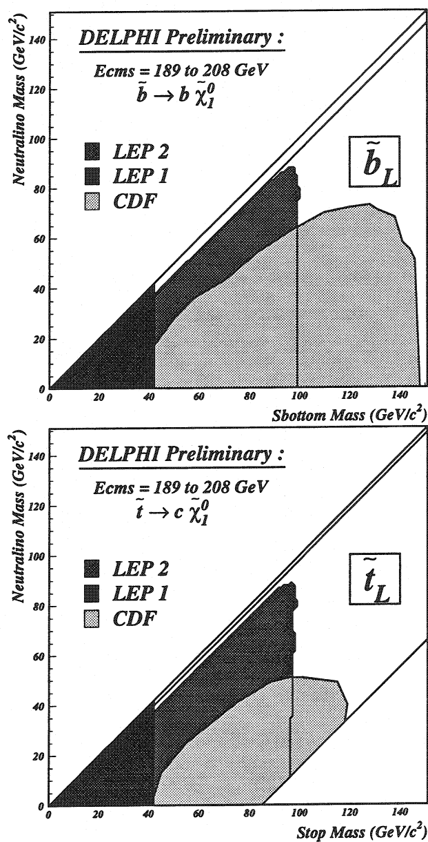
FIG. 7.30 – Régions exclues à 95% de niveau de confiance par l'expérience DELPHI à LEP1 et à LEP2, et par l'expérience CDF. L'histogramme du haut correspond à un sbottom purement gauche et celui du bas à un stop purement gauche.
