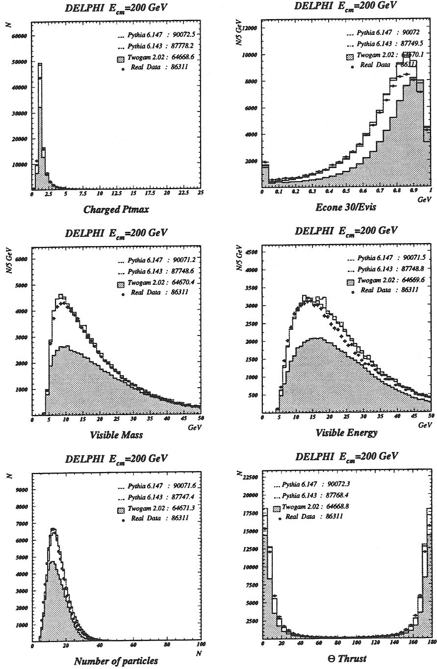
FIG. 6.18 – Comparaison entre les données de DELPHI collectées à \sqrt{s} = 200 GeV et la simulation (PYTHIA 6.143, PYTHIA 6.147 et TWOGAM 2.04, au deuxième niveau de sélection, après l'étape de repondération des poids des événements simulés.
