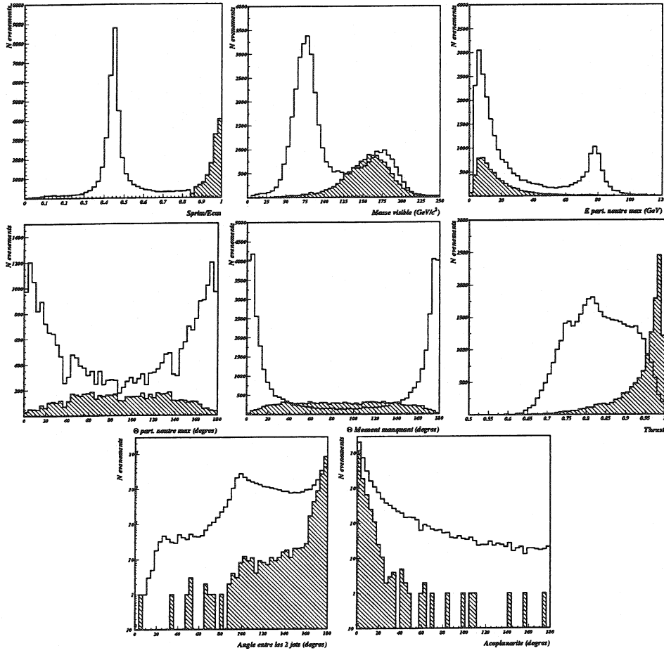
FIG. 6.4 – Distributions simulées du fond e^+e^- \rightarrow Z^0/\gamma^* \rightarrow q\bar{q}(\gamma) après reconstruction des événements par le détecteur DELPHI. La région hachurée correspond aux événements pour lesquels \sqrt{s'}/\sqrt{s} \geq 0.85 et la courbe noire aux événements pour lesquels \sqrt{s'}/\sqrt{s} < 0.85
