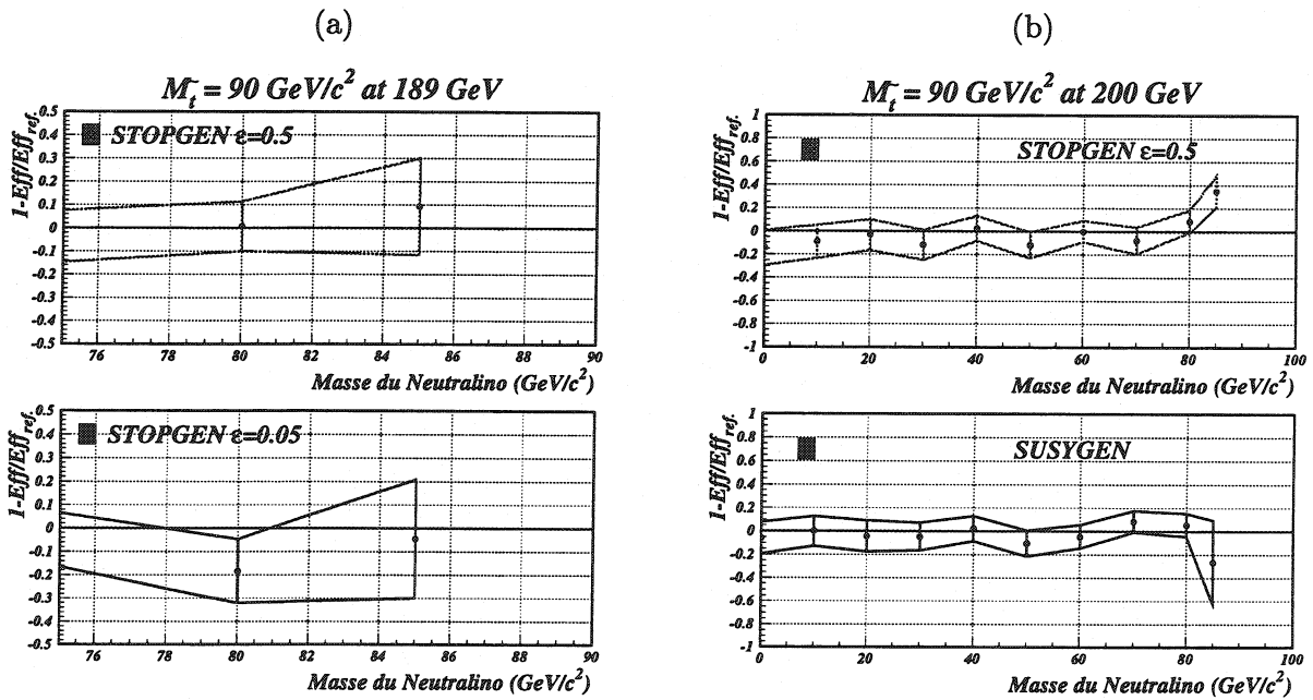
FIG. 7.25 – Différences relatives sur les efficacités de détection des signaux stop. (a) pour \Delta m \leq 10 \text{ GeV}/c^2 , le générateur de DELPHI est comparé à STOPGEN avec \epsilon_t = 0,05 et 0,5 . (b) pour \Delta m > 10 \text{ GeV}/c^2 , le générateur de DELPHI est comparé à STOPGEN avec \epsilon_t = 0,5 et à SUSYGEN.
