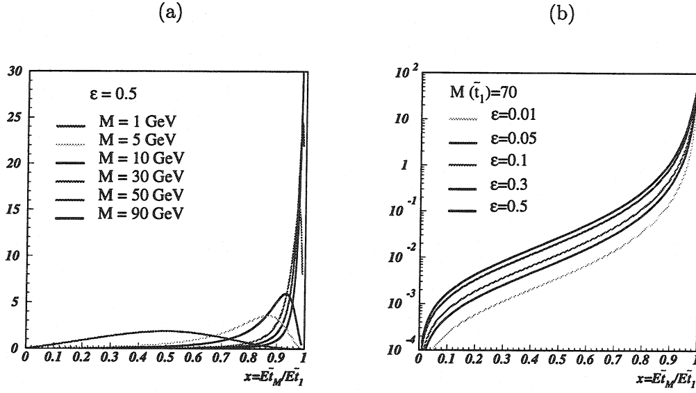
FIG. 2.8 – Distributions de Peterson: (2.8a) pour différentes valeurs de masse du stop avec \epsilon = 0.5 \text{ GeV}/c^2 , (2.8b) pour différentes valeurs de \epsilon avec m_{\tilde{t}_1} = 70 \text{ GeV}/c^2 .
