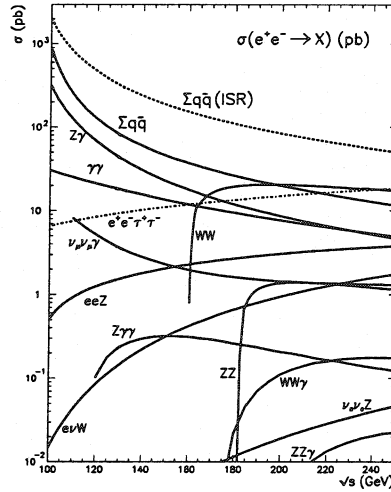
FIG. 6.1 – Sections efficaces des processus attendus à LEP2 en fonction de l'énergie dans le centre de masse.
