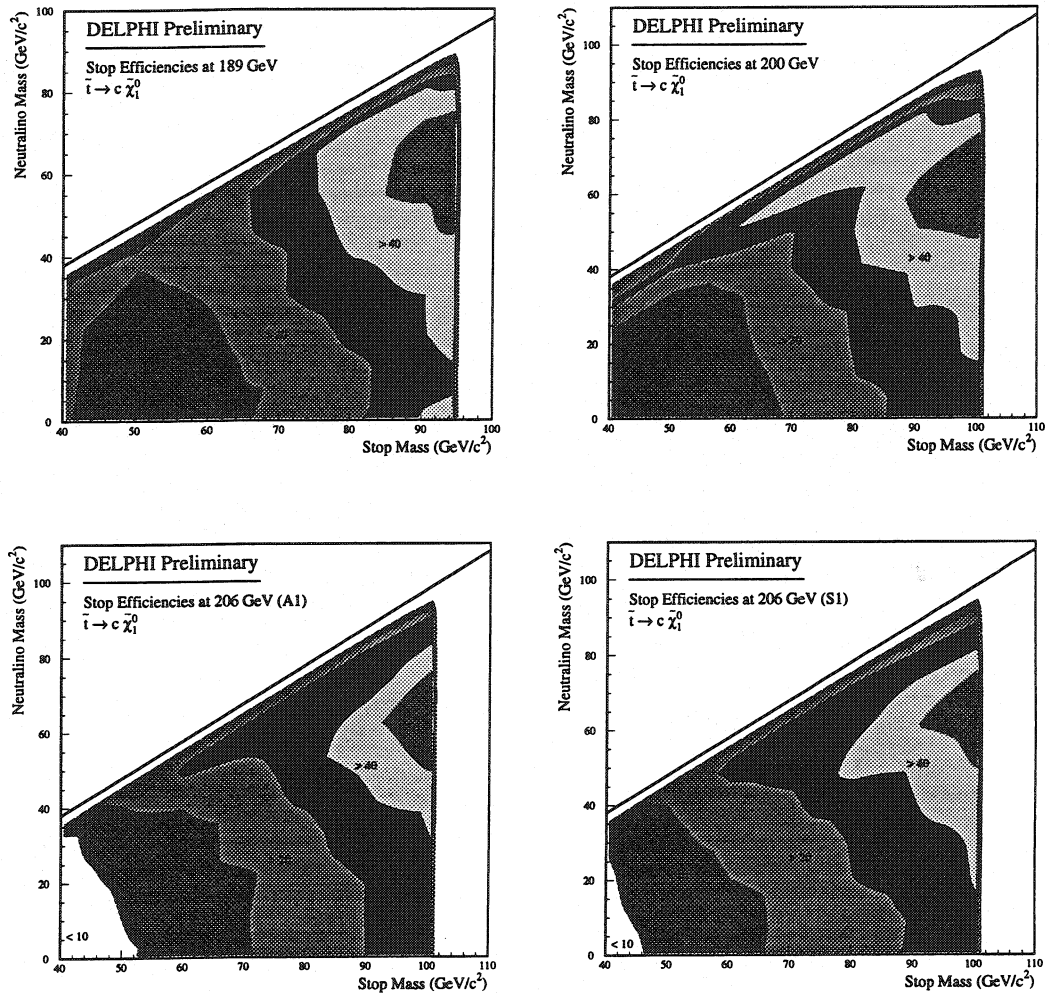
FIG. 7.22 – Efficacités de détection des signaux stop interpolées avec un pas de 1 GeV/c 2 dans le plan (m_{\tilde{t}_1}, m_{\tilde{\chi}_1^0}) .
