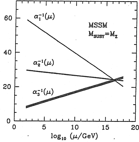
FIG. 1.4 – Evolution des constantes de couplage dans le MSSM.
