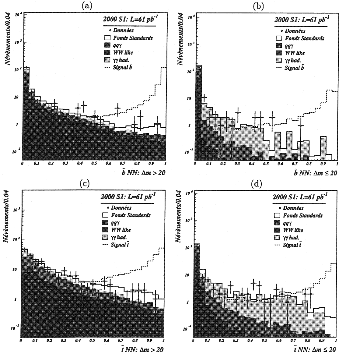
FIG. 7.17 – Données 2000 S1: sorties des réseaux de neurones des quatre analyses: (a) sbottom \Delta m > 20 \text{ GeV}/c^2 , (b) sbottom \Delta m \leq 20 \text{ GeV}/c^2 , (c) stop \Delta m > 20 \text{ GeV}/c^2 , (d) stop \Delta m \leq 20 \text{ GeV}/c^2 .
