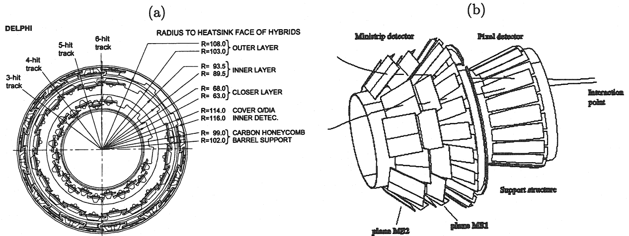
FIG. 4.6 – (a) Vue en coupe de la partie centrale du détecteur de vertex. (b) Le VFT
