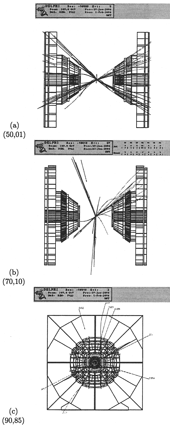
FIG. 3.7 – Topologies des événements stop en fonction de la masse du gluino.
