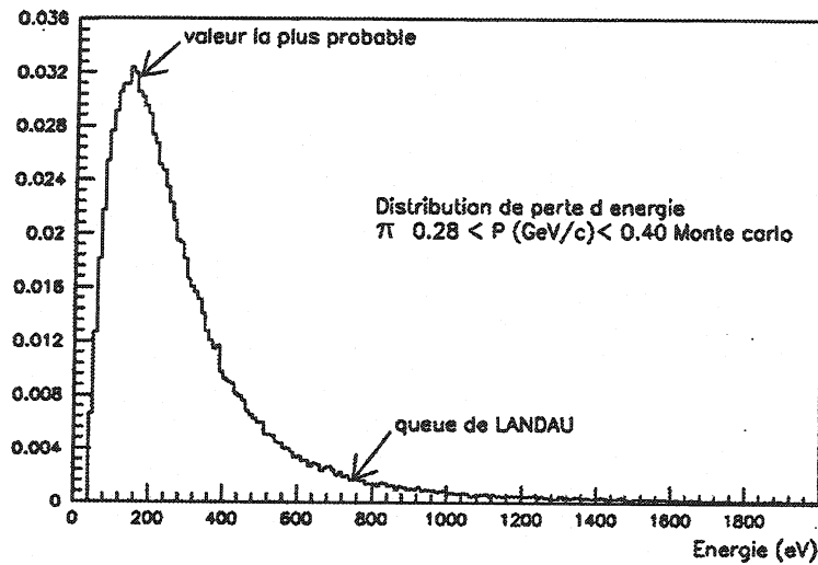
FIG. 5.6 – Distribution de perte d'énergie simulée pour des pions proches du minimum ionisant.
