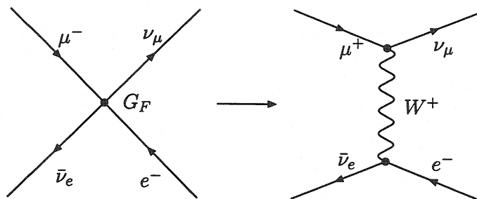
FIG. 1.1 – Diagrammes de désintégration du muon: \mu^- \rightarrow \nu_\mu e^- \bar{\nu}_e .
