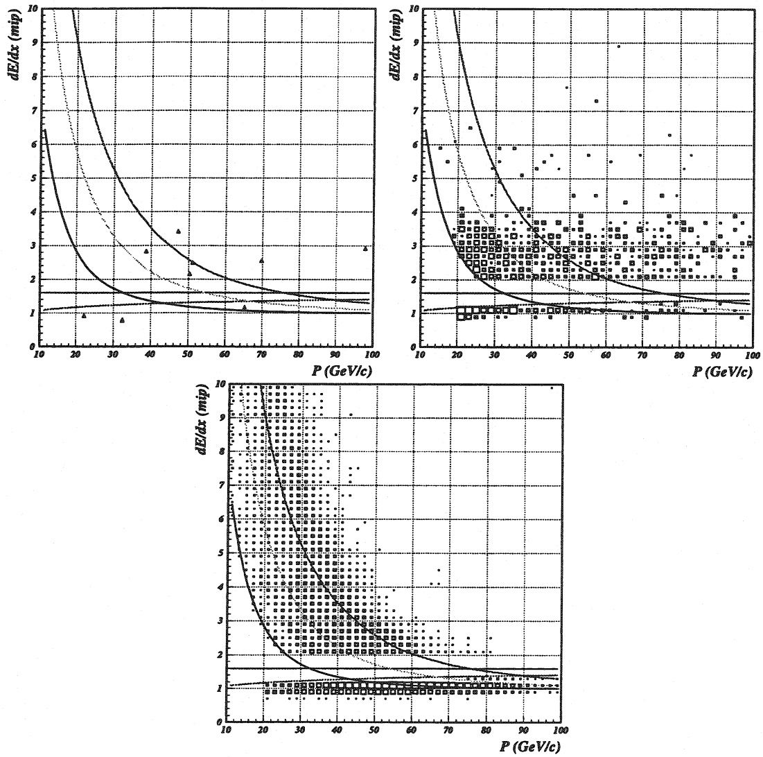
FIG. 8.13 – Recherche des événements q\bar{q}R^0R^\pm : dE/dx (mip) en fonction de l'impulsion (GeV/c) des candidats R^\pm sélectionnés: (a) pour les données réelles (b) pour les processus standards simulés, (c) pour les signaux stop et sbottom simulés.
