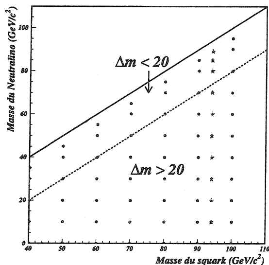
FIG. 7.2 – Points simulés dans le plan (m_{\tilde{q}_1}, m_{\tilde{\chi}_1^0}) pour les analyses de recherche des squarks. Les ronds correspondent aux points simulés à 200 et 206 GeV. A 189 GeV, la masse de squark simulée la plus grande est 94 GeV/c 2 (étoiles). La ligne à \Delta m = 20 GeV/c 2 montre la limite entre les deux analyses à haute et basse différence de masse.
