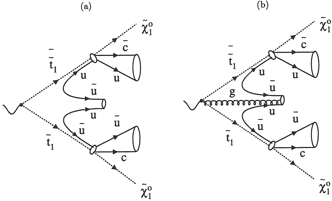
FIG. 2.9 – Schématisation de l'hadronisation du stop: (a) e^+e^- \rightarrow \tilde{t}_1 \bar{\tilde{t}}_1 (b) e^+e^- \rightarrow \tilde{t}_1 \bar{\tilde{t}}_1 g . Les ellipses indiquent les singlets de couleur SU(3) .
