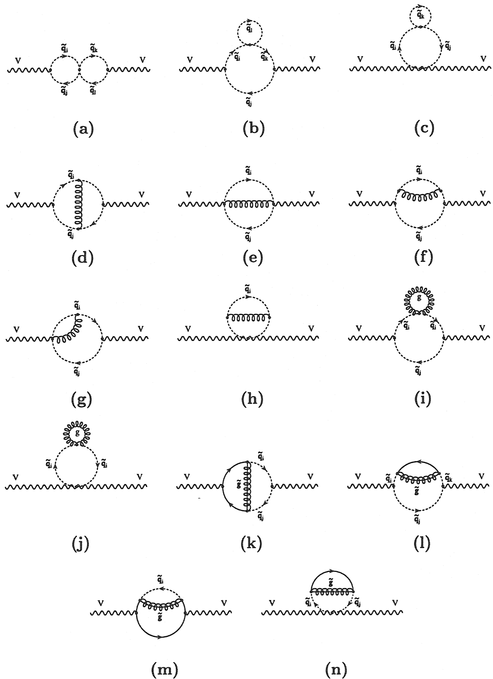
FIG. 9.2 – Contribution des squarks à l'énergie propre des bosons de jauge à deux boucles.
