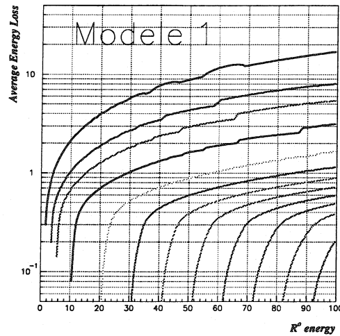
FIG. 3.5 – Perte d'énergie d'un R^0 au cours de 4 collisions en fonction de son énergie initiale. Les courbes correspondent à différentes hypothèses de masse: 1, 3, 5, 10, 20, 30, 40, 50, 60, 70, 80 et 90 \text{GeV}/c^2 . Le R^0 perdant un maximum d'énergie lorsque sa masse est petite.
