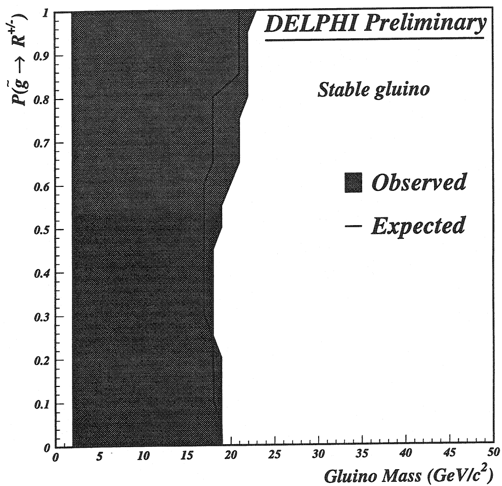
FIG. 8.32 – Région exclue à 95% de niveau de confiance dans le plan (m_{\tilde{g}}, P) . La région pleine correspond à l'exclusion observée et la ligne à l'exclusion attendue.
