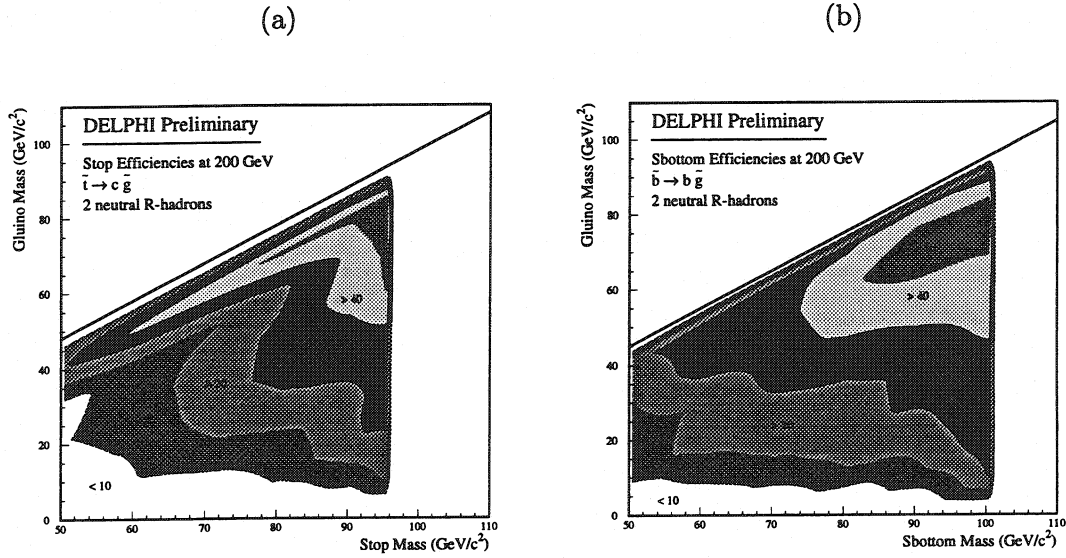
FIG. 8.22 – Efficacités de détection des signaux stop (a) et sbottom (b) où les deux gluinos s'hadronisent en R -hadrons neutres ( \sqrt{s} = 200 \text{ GeV} ).
