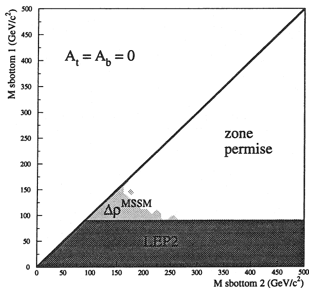
FIG. 9.3 – Régions exclues par la recherche directe des squarks à LEP2 et par la précision sur le paramètre \Delta\rho calculée dans le Modèle Standard. Les histogrammes montrent ces exclusions dans le plan (m_{\tilde{q}_1}, m_{\tilde{q}_2}) pour le stop (haut) et pour le sbottom (bas).
