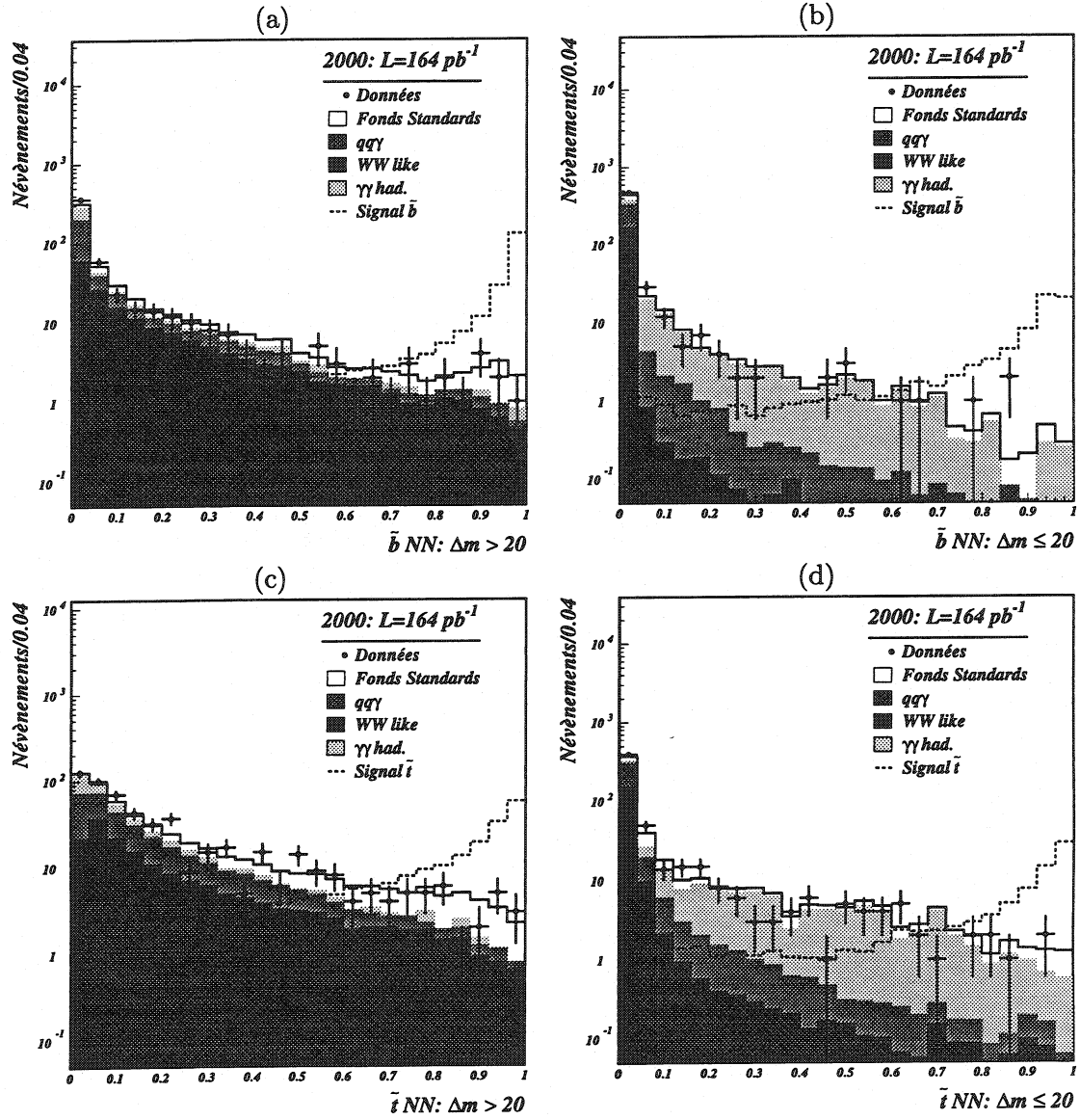
FIG. 7.16 – Données 2000: sorties des réseaux de neurones des quatre analyses: (a) sbottom \Delta m > 20 \text{ GeV}/c^2 , (b) sbottom \Delta m \leq 20 \text{ GeV}/c^2 , (c) stop \Delta m > 20 \text{ GeV}/c^2 , (d) stop \Delta m \leq 20 \text{ GeV}/c^2 .
