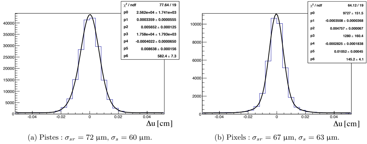
FIGURE 5.26 – Distributions de résidus mesurées sur le détecteur hybride PMM_2011.2, à basse intensité ( I \approx 10^5 \mu/s ).
