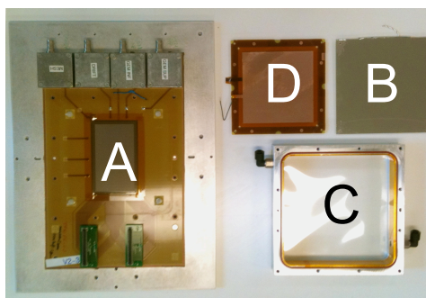
FIGURE 4.8 – Détecteur hybride de type TF10 utilisé pour les campagnes de tests de 2010. A : plancher bulk ( 4 \times 10 \text{ cm}^2 de zone active) ; B : électrode de dérive ; C : fenêtre de fermeture ; D : feuille GEM ( 10 \times 10 \text{ cm}^2 de zone active) [84].
