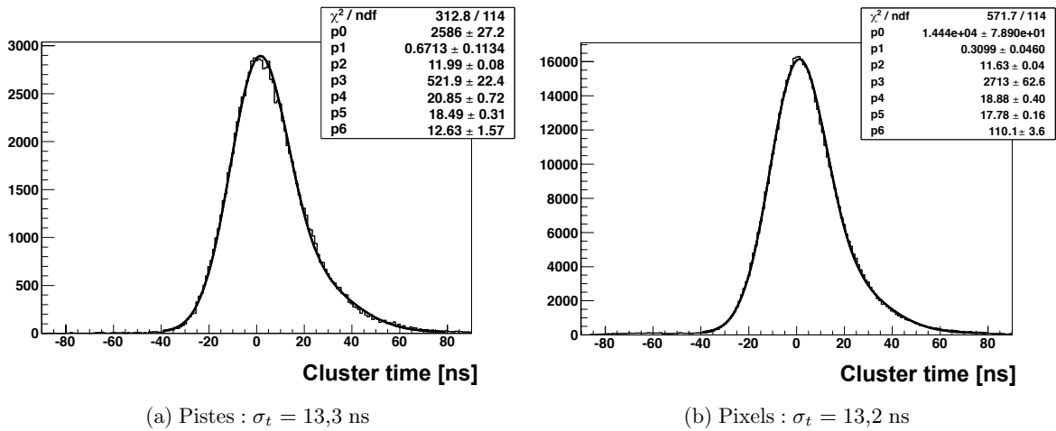
FIGURE 5.30 – Distribution du temps des clusters pour le détecteur hybride PMM_2011.2, dans le mélange gazeux Ne/C 2 H 6 /CF 4 en proportions 85/10/5 ( I \approx 5 \times 10^6 \mu\text{s} ).
