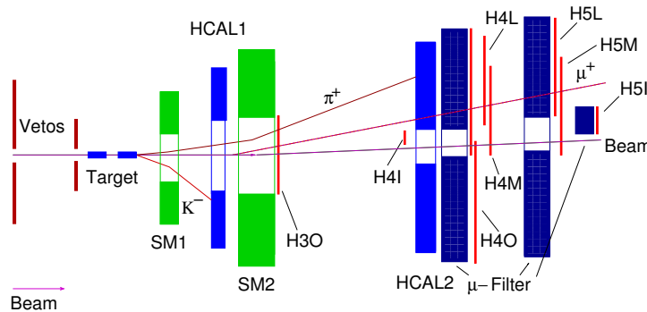
FIGURE 2.13 – Position des détecteurs participant au déclenchement de l'acquisition.
