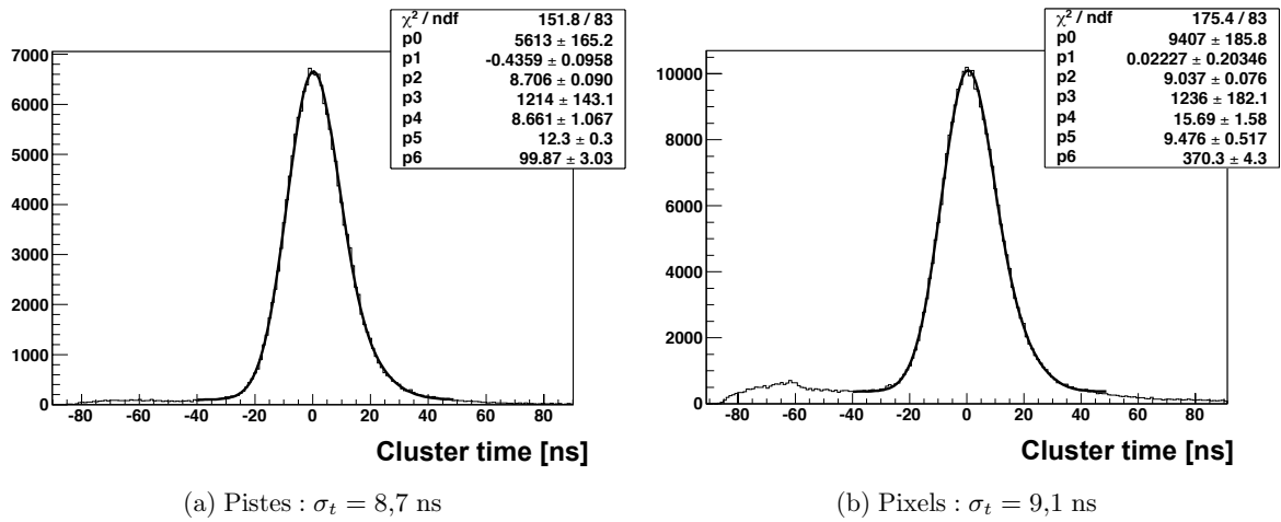
FIGURE 5.29 – Distribution du temps des clusters pour le détecteur hybride PMM_2011.2, dans le mélange gazeux Ne/C 2 H 6 /CF 4 en proportions 80/10/10 ( I \approx 3,5 \times 10^7 \mu\text{s} ).
