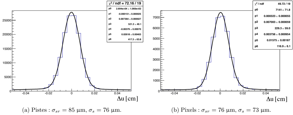
FIGURE 5.27 – Distributions de résidus mesurées sur le détecteur résistif PMM_2011.3, à basse intensité ( I \approx 10^5 \mu/s ).
