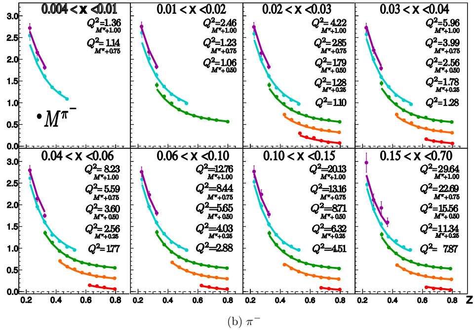
FIGURE 8.8 – Multiplicités de pions en fonction de z pour différents domaines en x et Q^2 , avec ajustement à l'ordre dominant. Chacune des 8 parties de la figure représente un domaine en x ; dans chacune d'entre elles les valeurs de multiplicités sont décalées d'une constante pour plus de lisibilité. Les valeurs de Q^2 moyennes indiquées correspondent à chacune des courbes et sont classées dans le même ordre que celles-ci.
