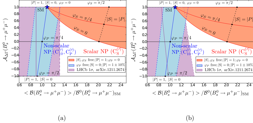
Figure 10: Régions permises dans le plan \mathcal{B}(B_s^0 \rightarrow \mu^+ \mu^-) / \mathcal{B}(B_s^0 \rightarrow \mu^+ \mu^-)_{\text{SM}} \times \mathcal{A}_{\Delta\Gamma} si les contributions de la nouvelle physique sont scalaires (rouge) ou non-scalaire (bleue) sur imprimée avec la contrainte expérimentale (violet) avec (b) ou sans (a) la dépendance en \mathcal{A}_{\Delta\Gamma} [17].
