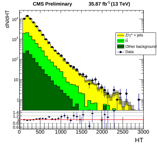
(d) Scalar sum of all jets p_T .
